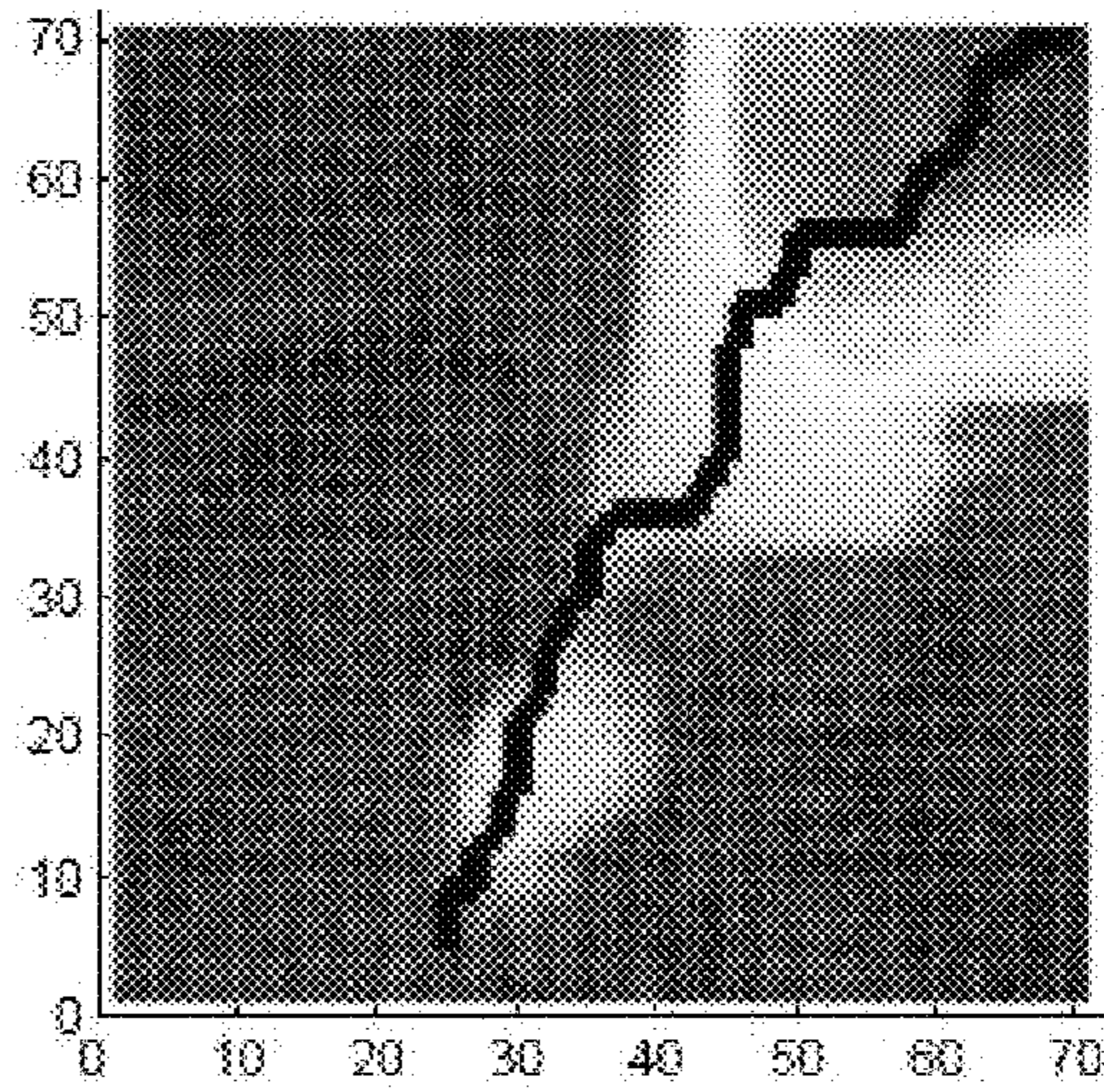
(d) \tau = 0.4
