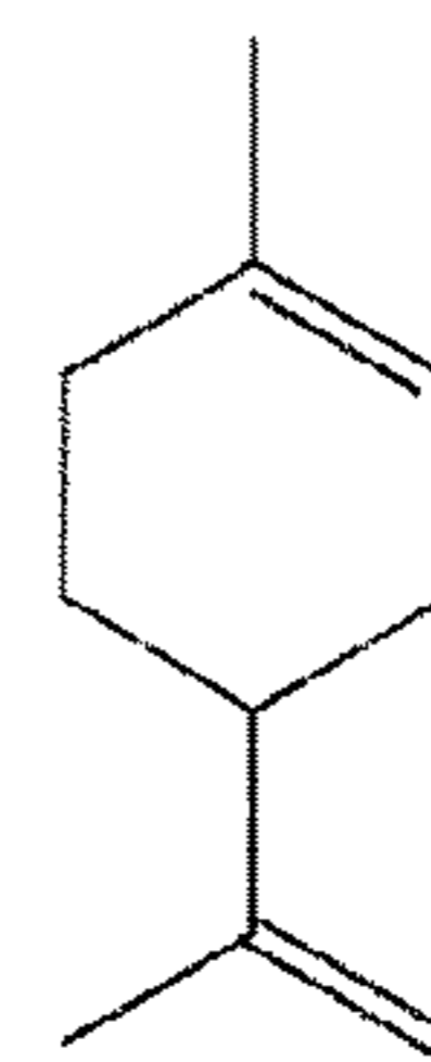
Limonene
