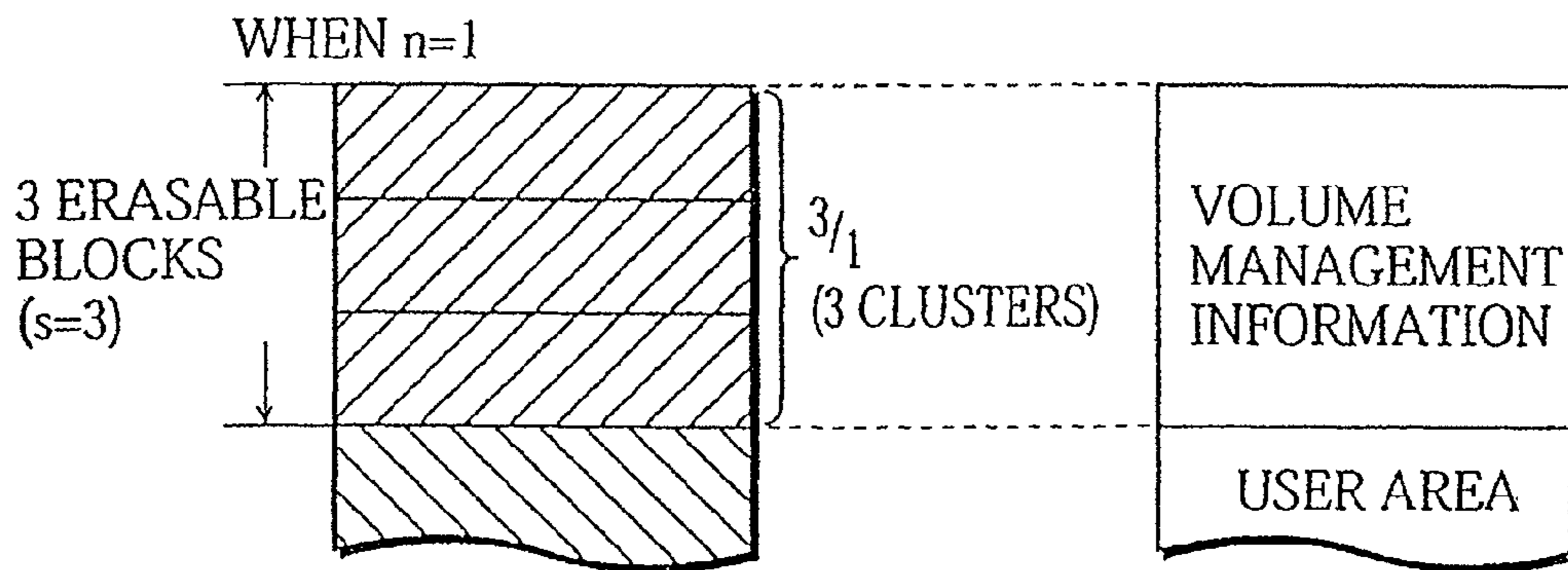
FIG. 11B
