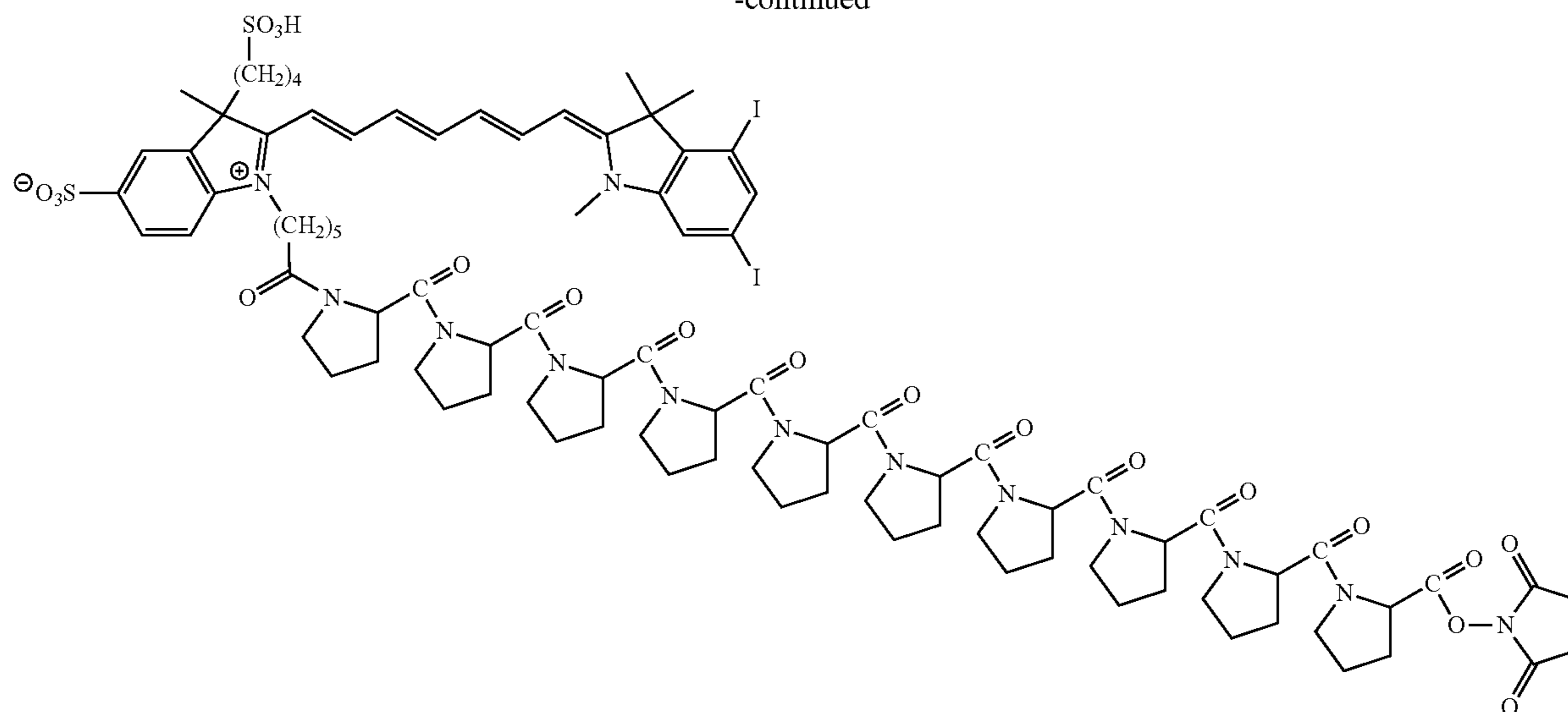
I-90 NHS ester
