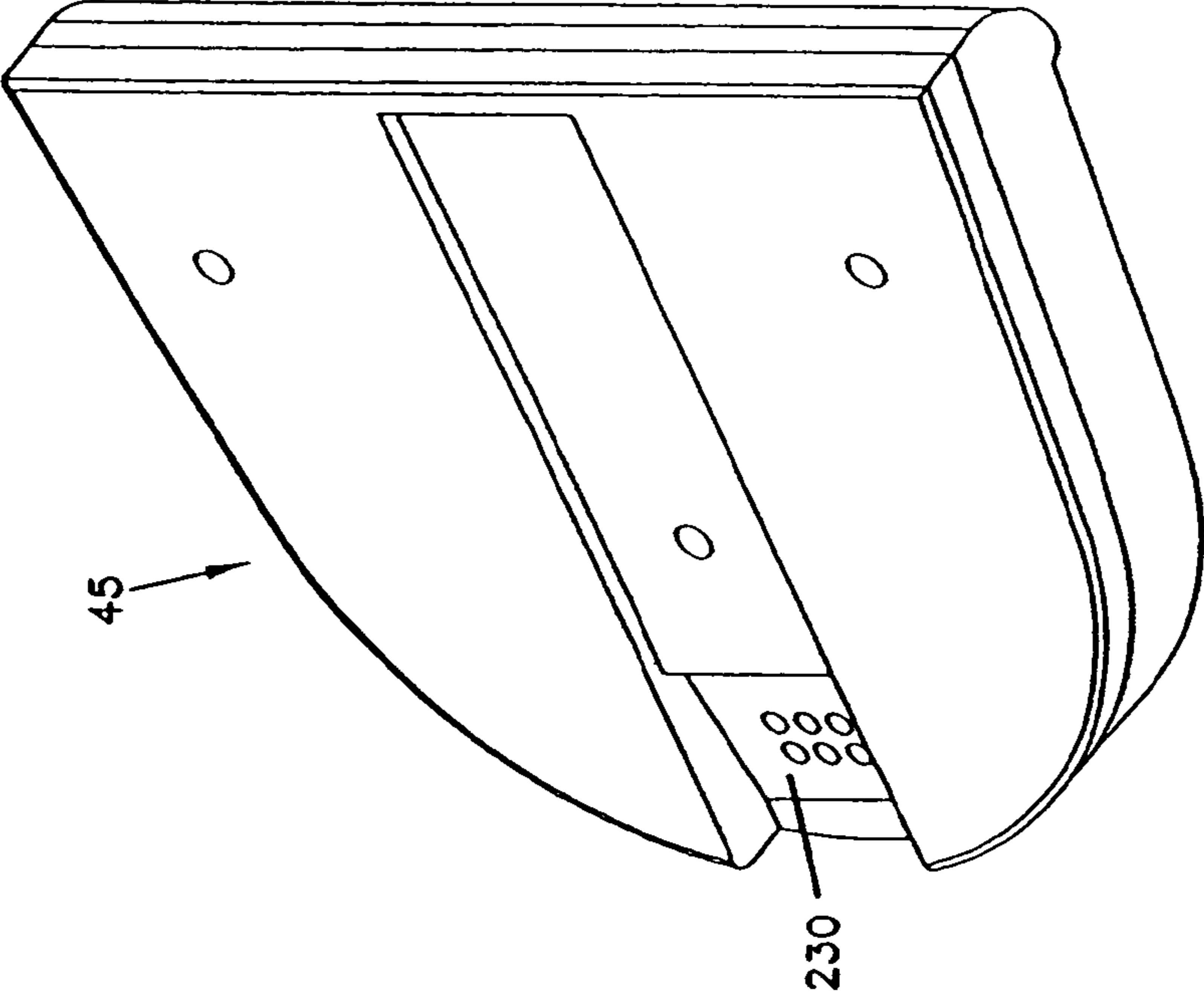
FIG. 28D
