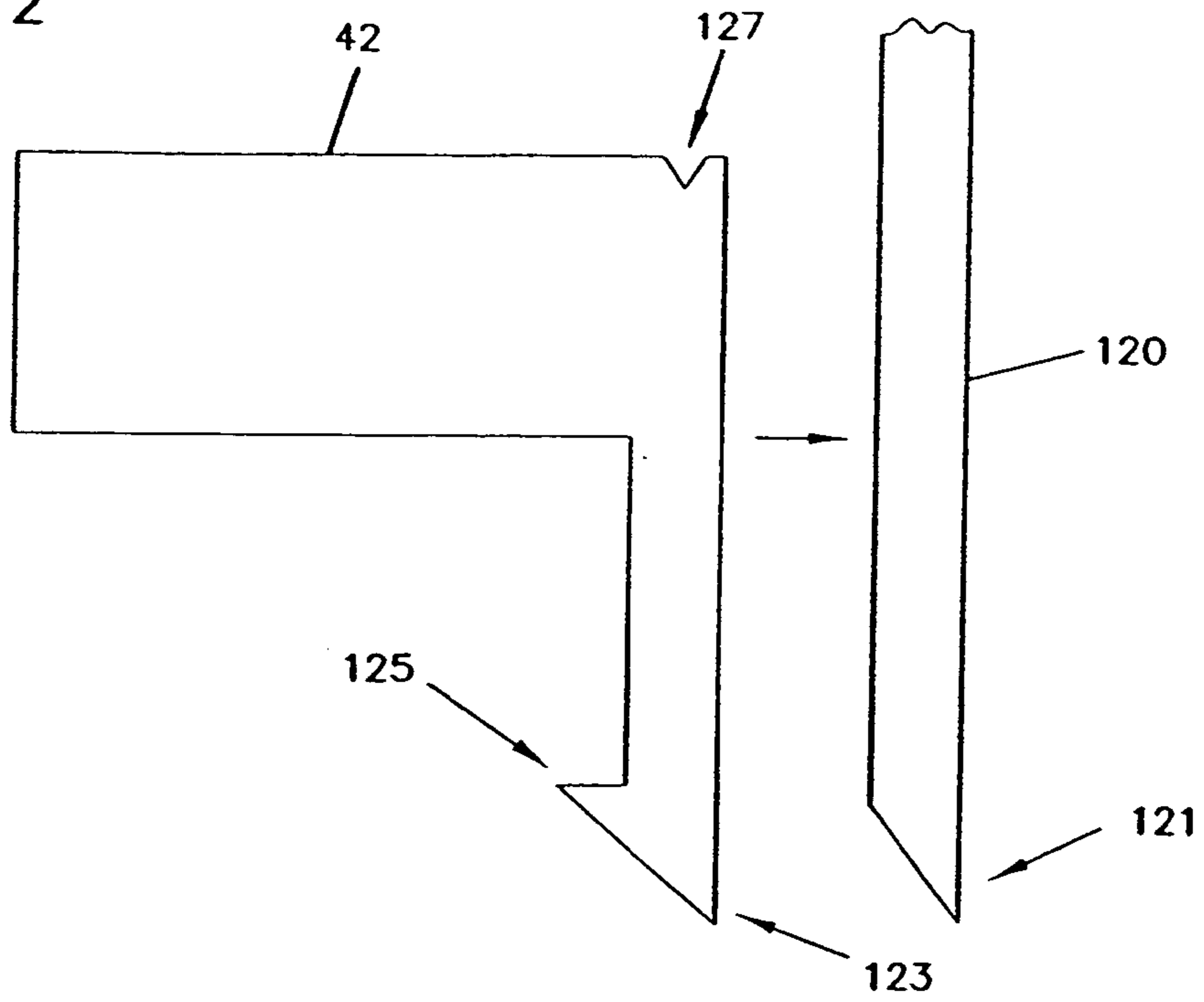
FIG. 13B
