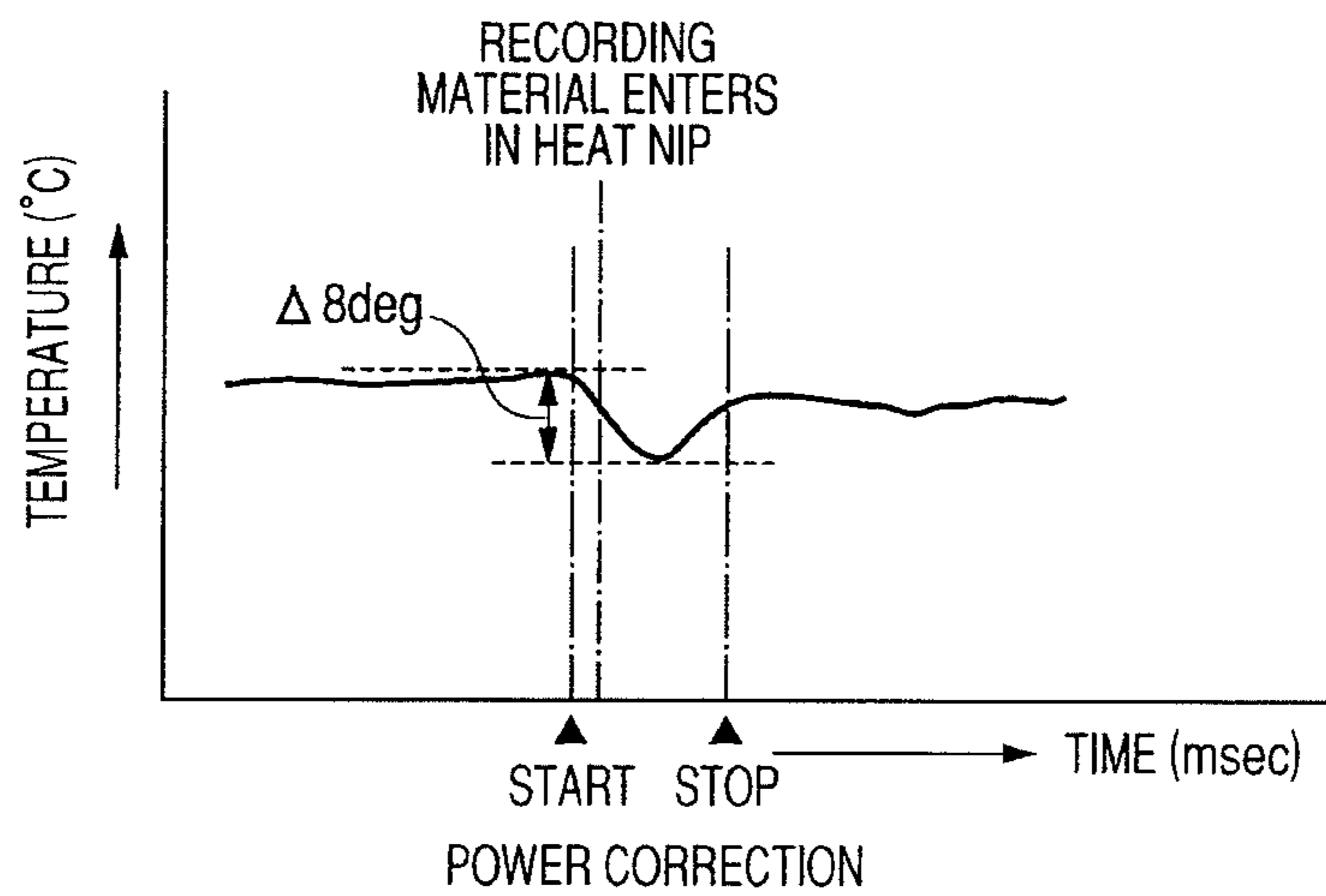
FIG. 16
