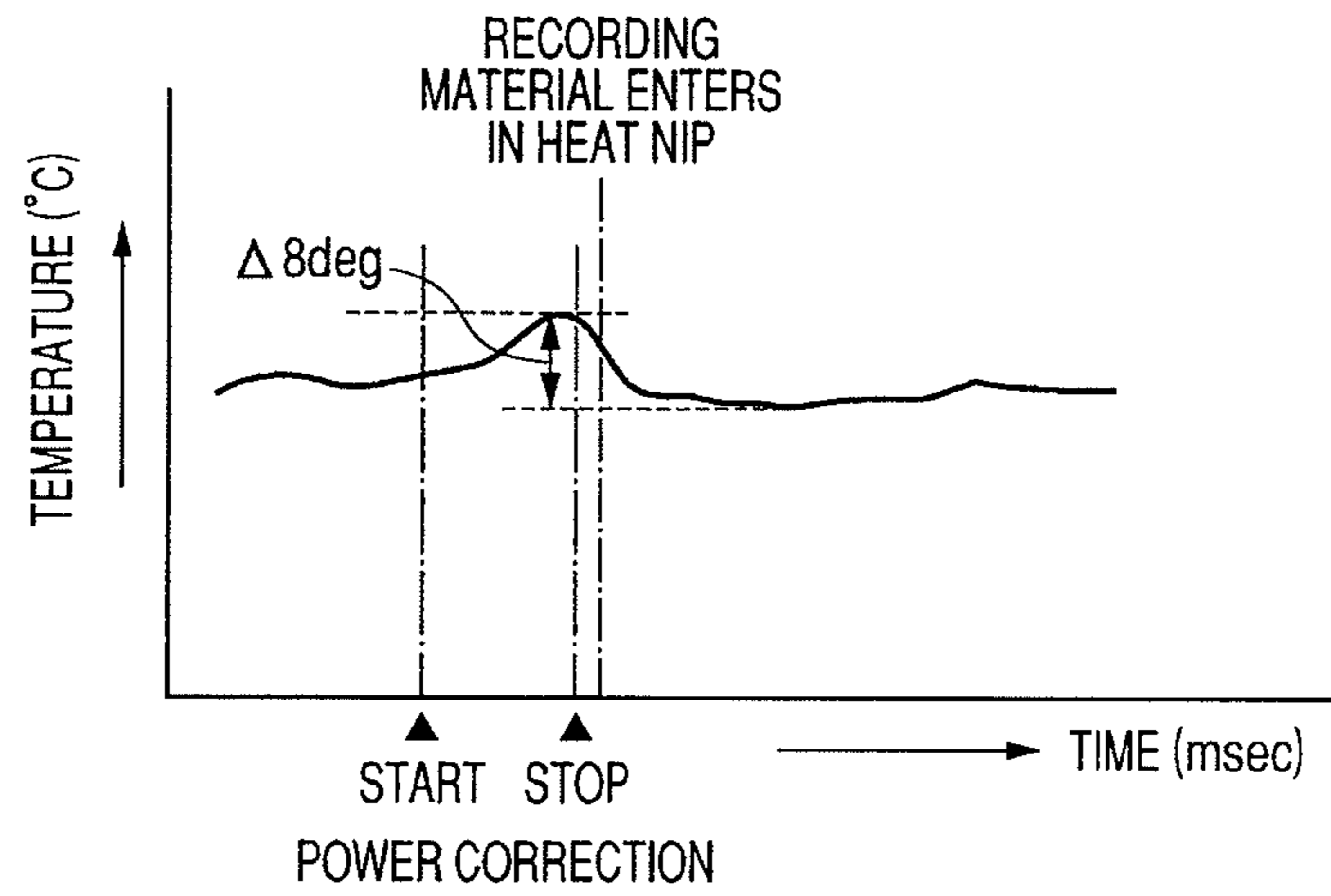
FIG. 15
