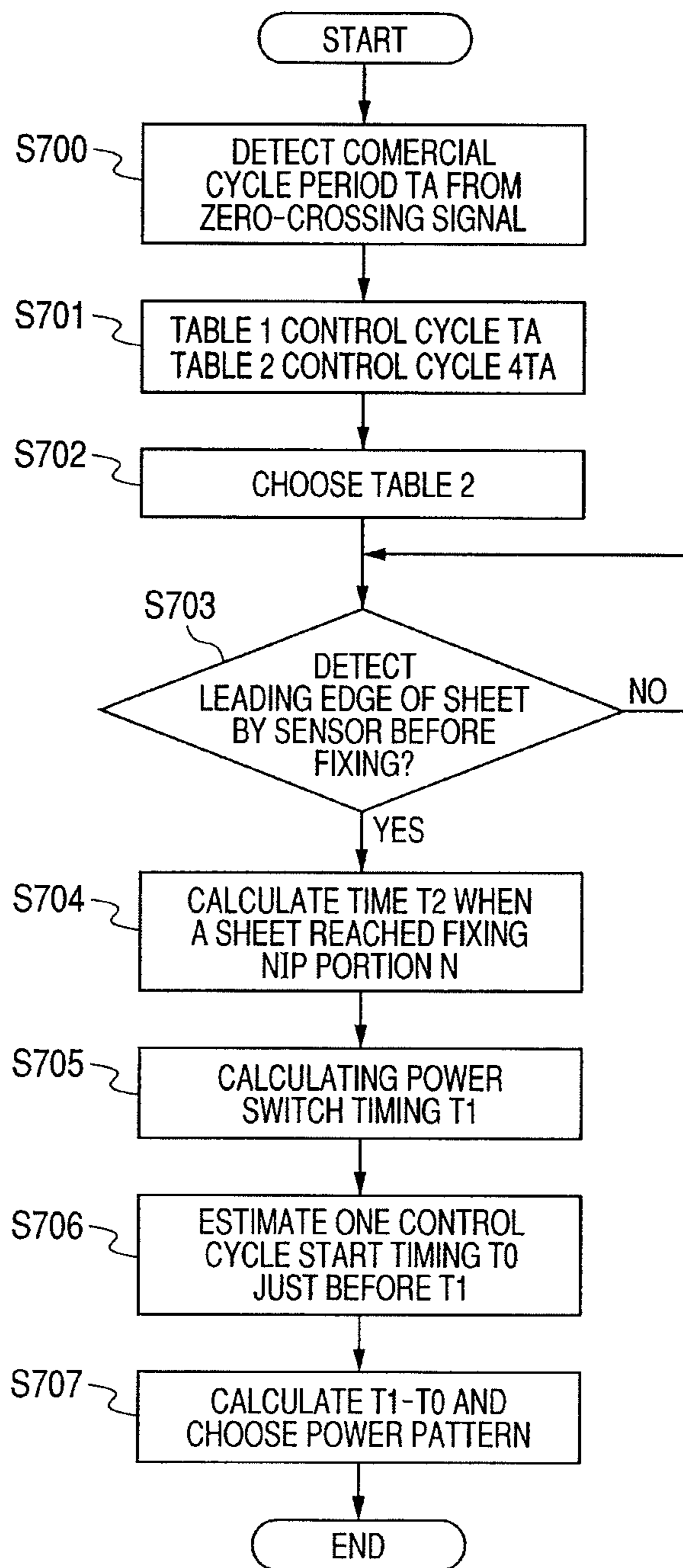
FIG. 26
