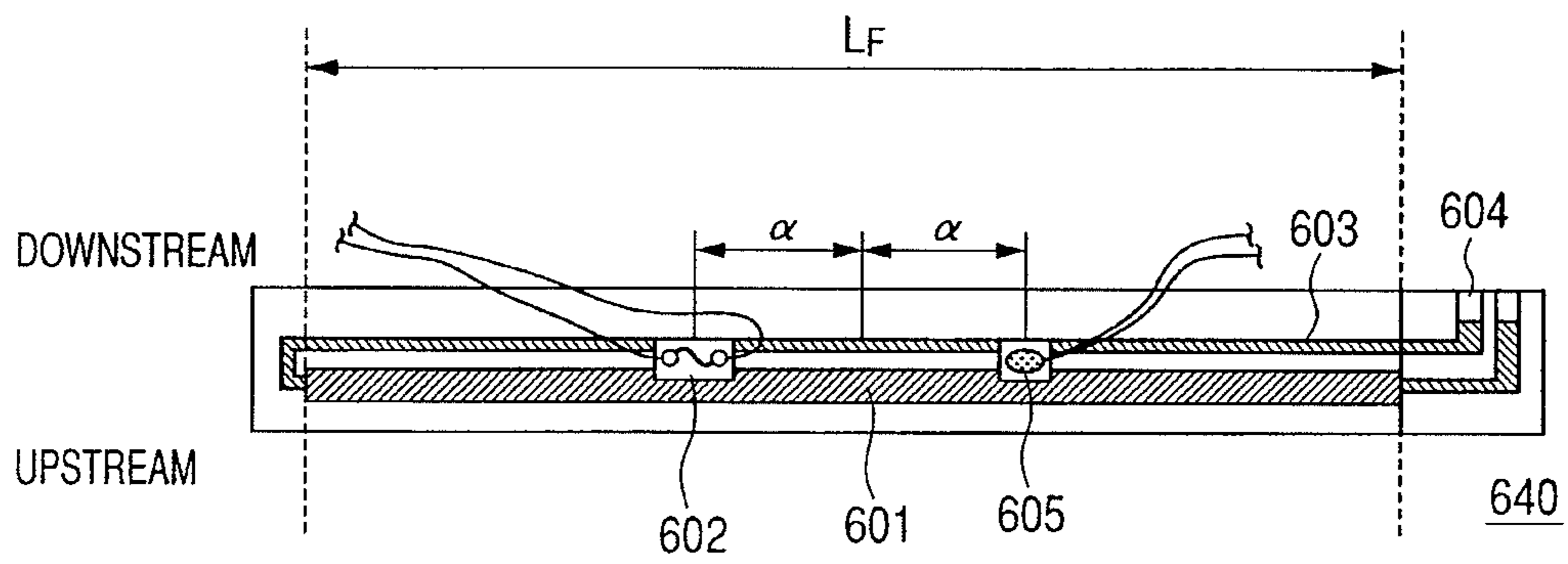
FIG. 20B
