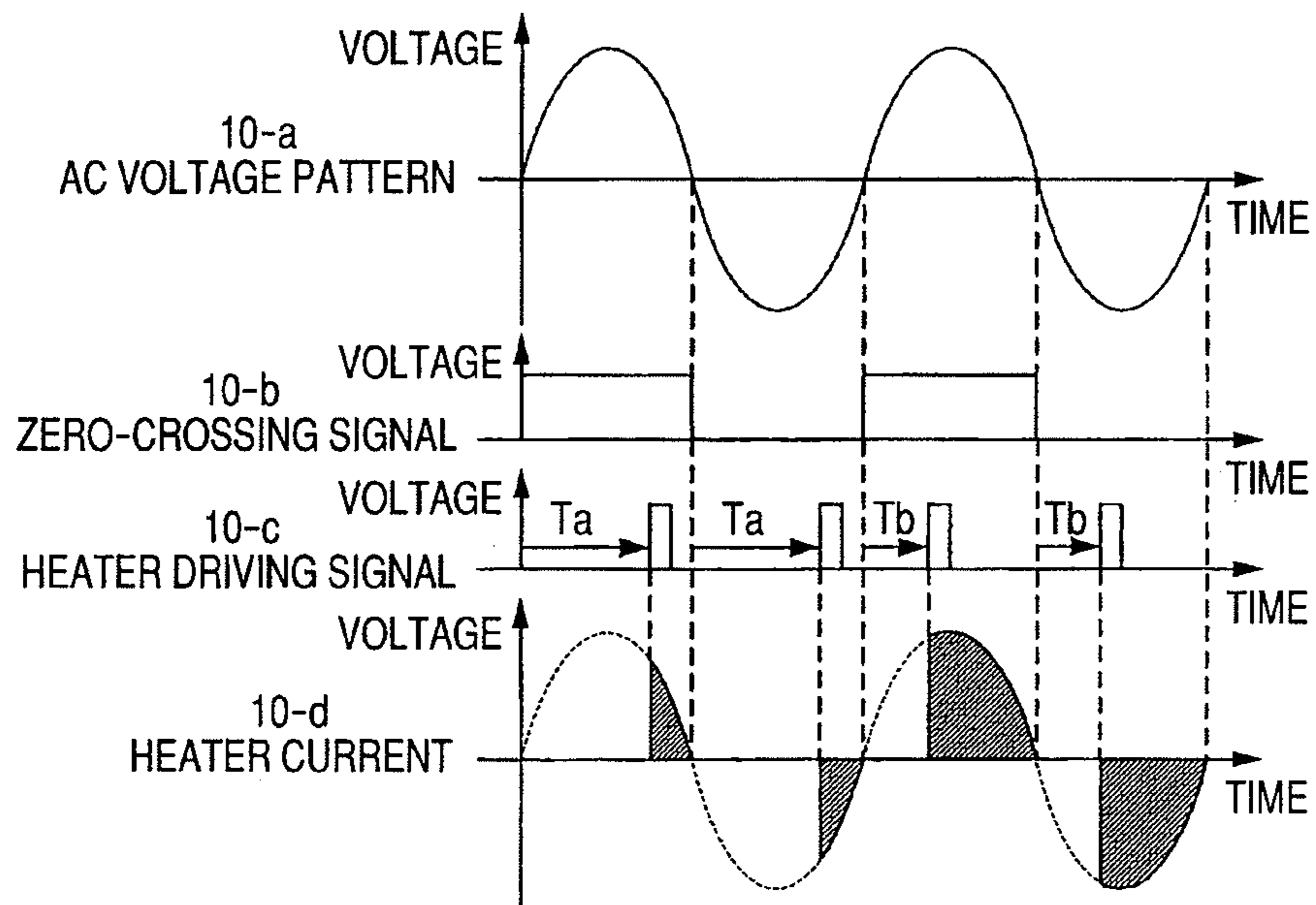
FIG. 22
