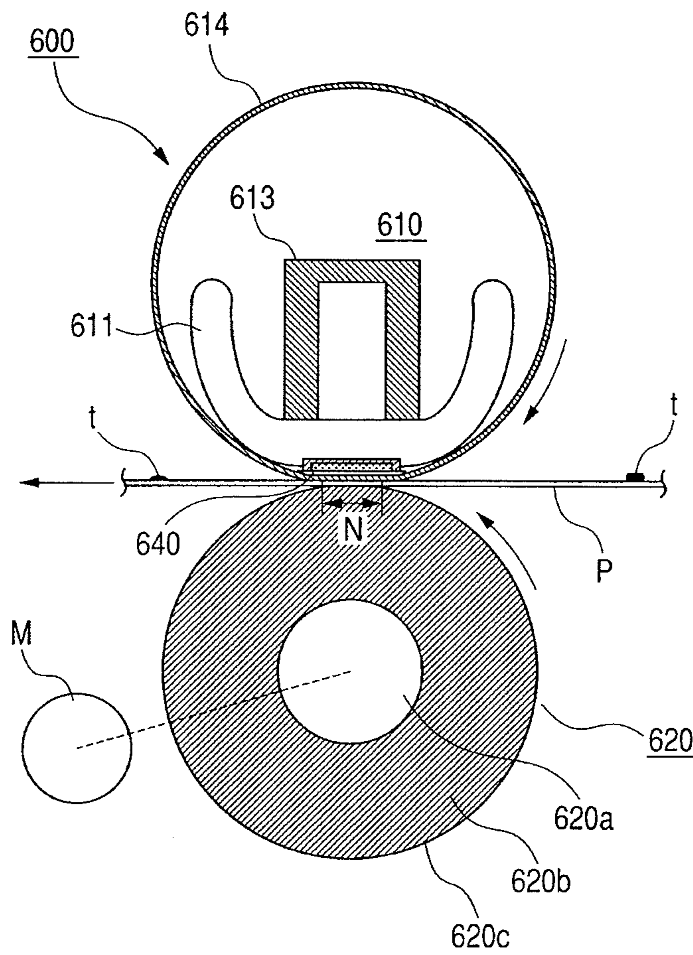
FIG. 19
