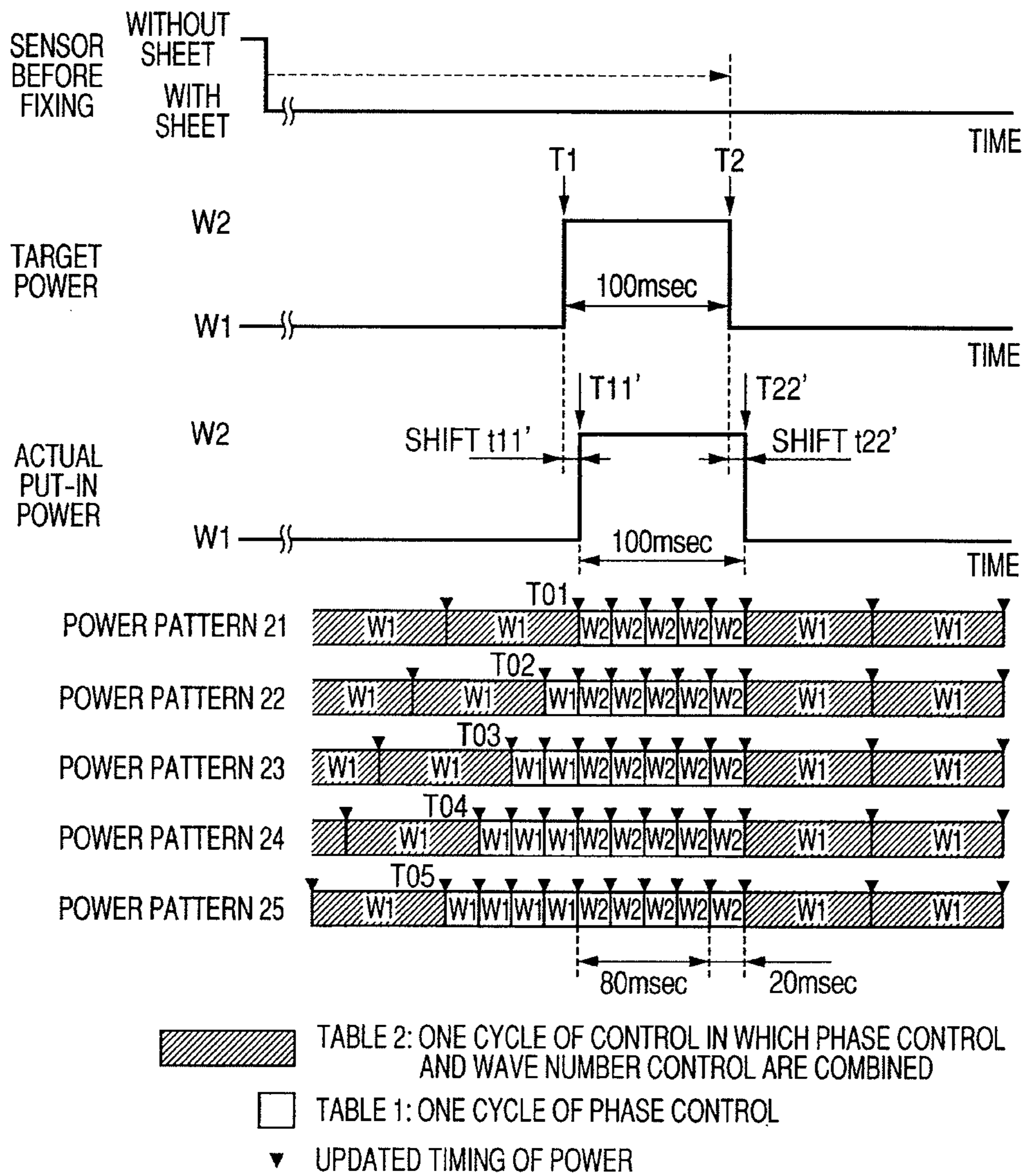
FIG. 27
