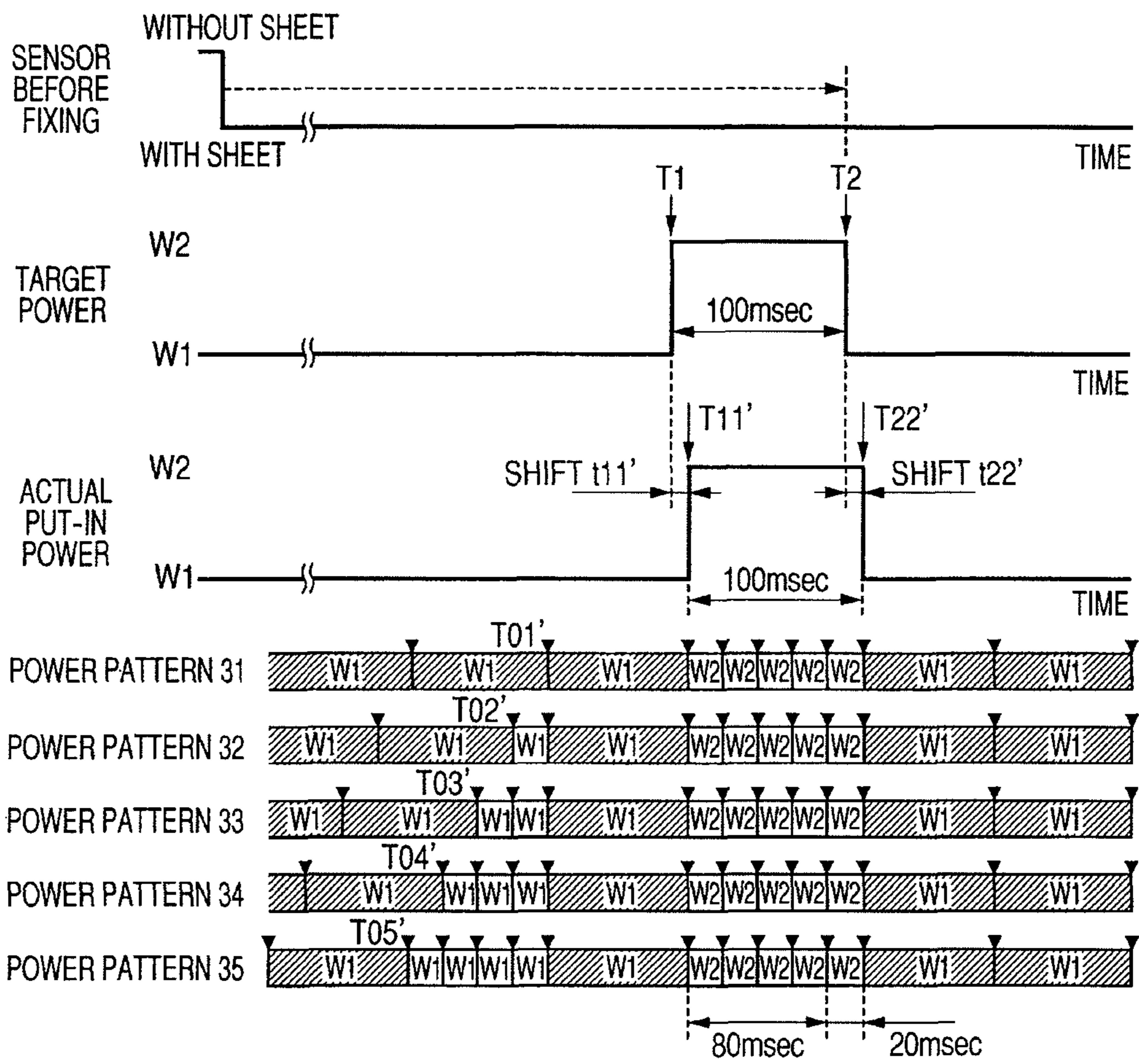
FIG. 28
