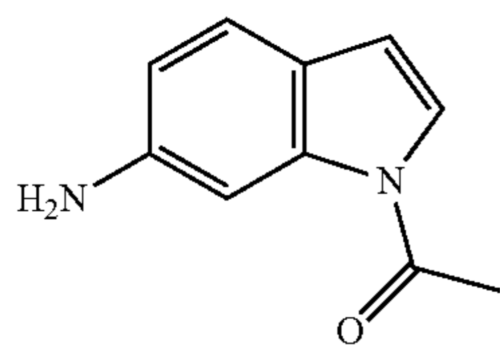
B-3; 1-(6-Amino-indol-1-yl)-ethanone
