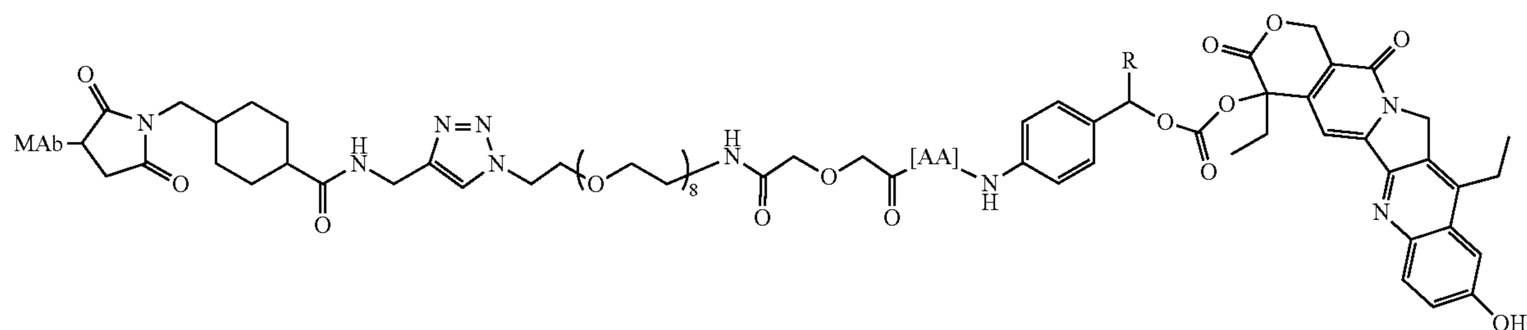
MAb-CLX-SN-38
