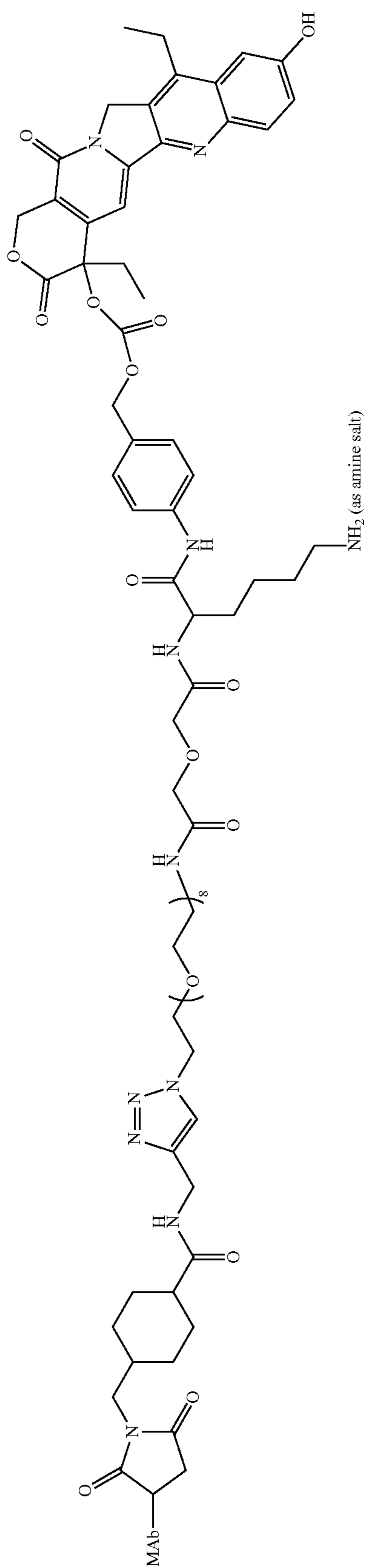
CL2A-SIN-38
