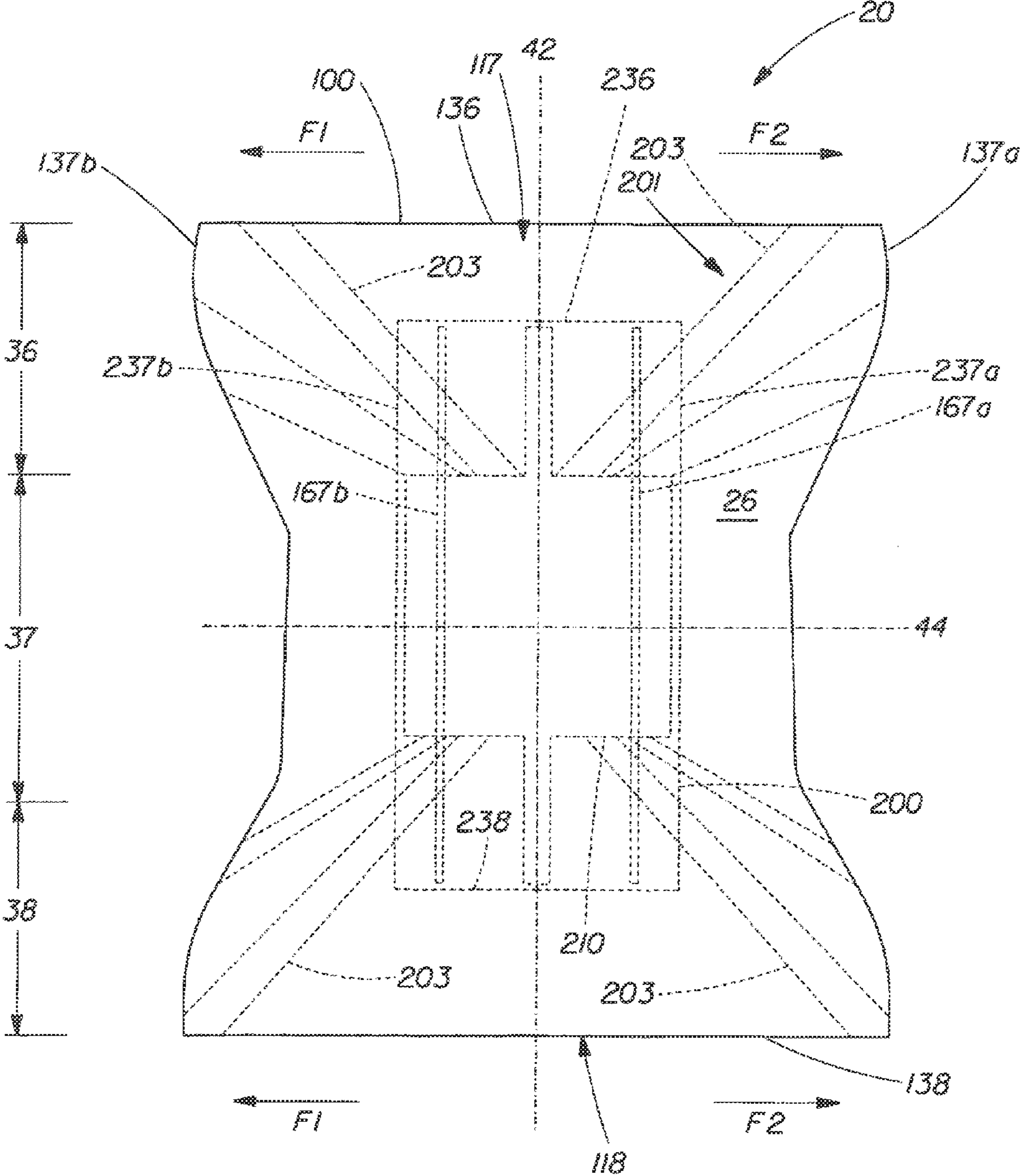
Fig. 30
