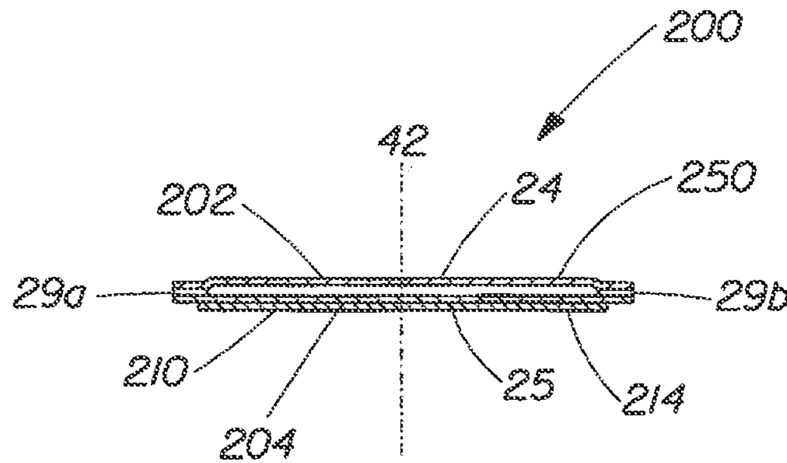
Fig. 24
