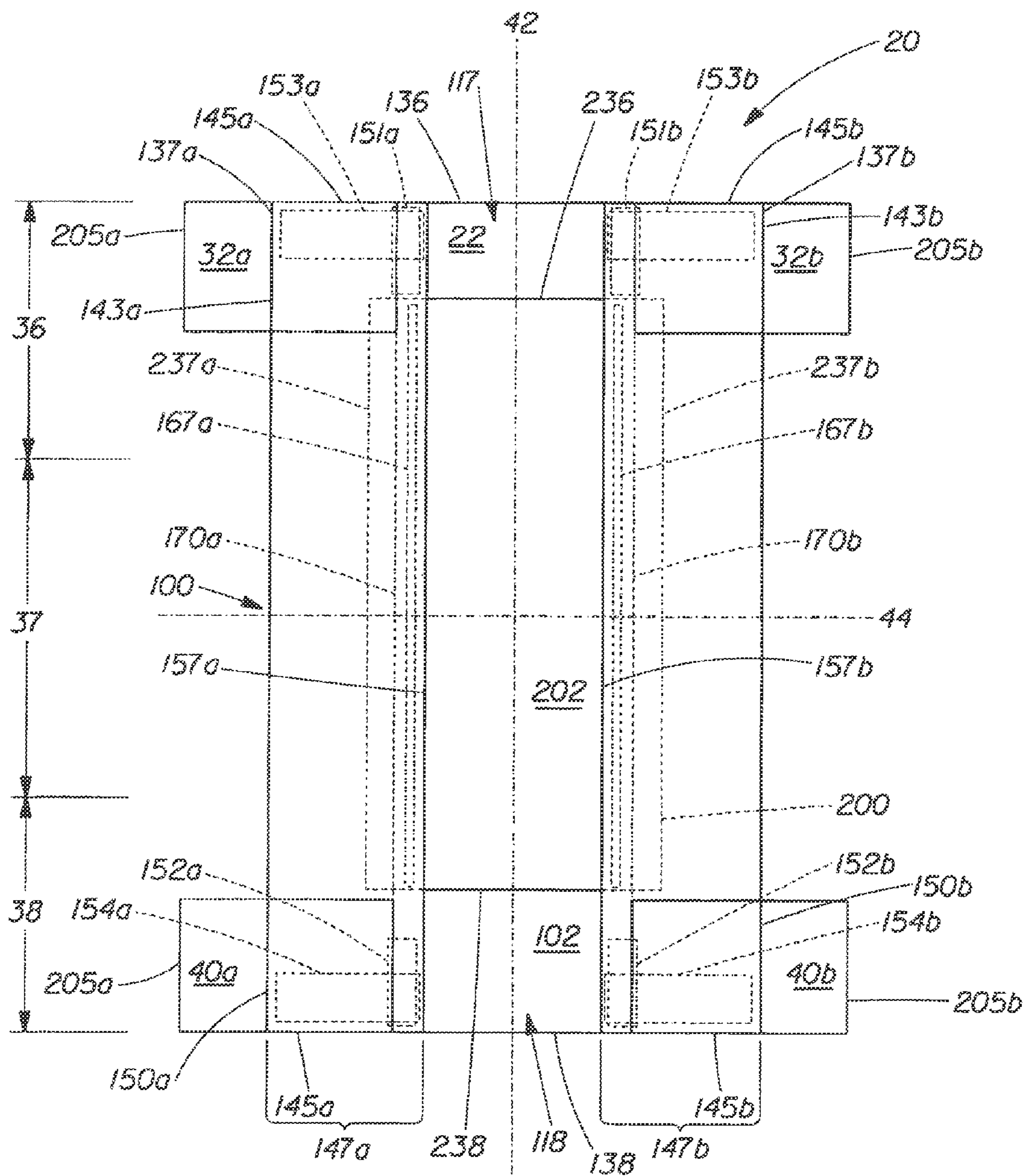
Fig. 19B
