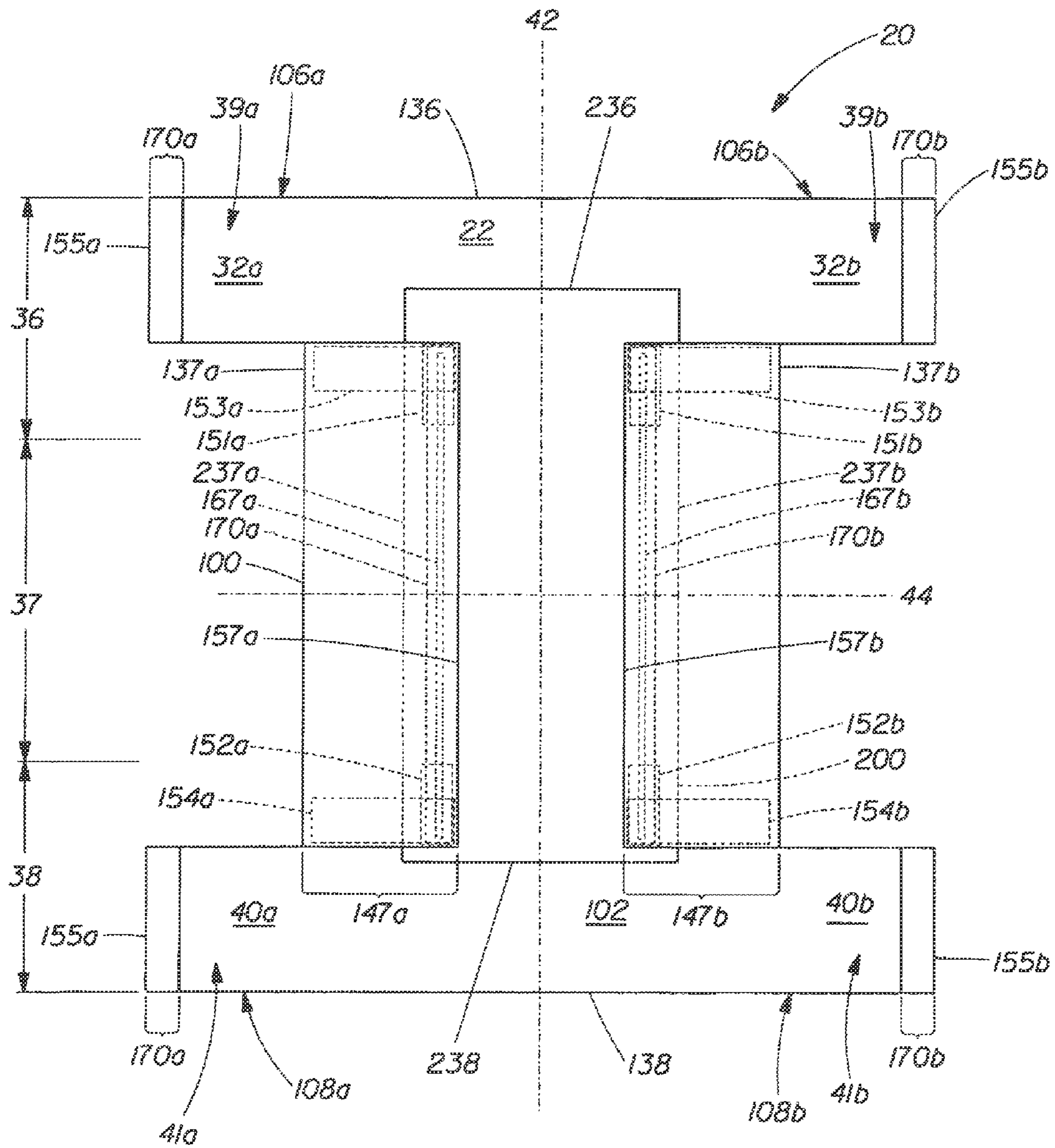
Fig. 19A
