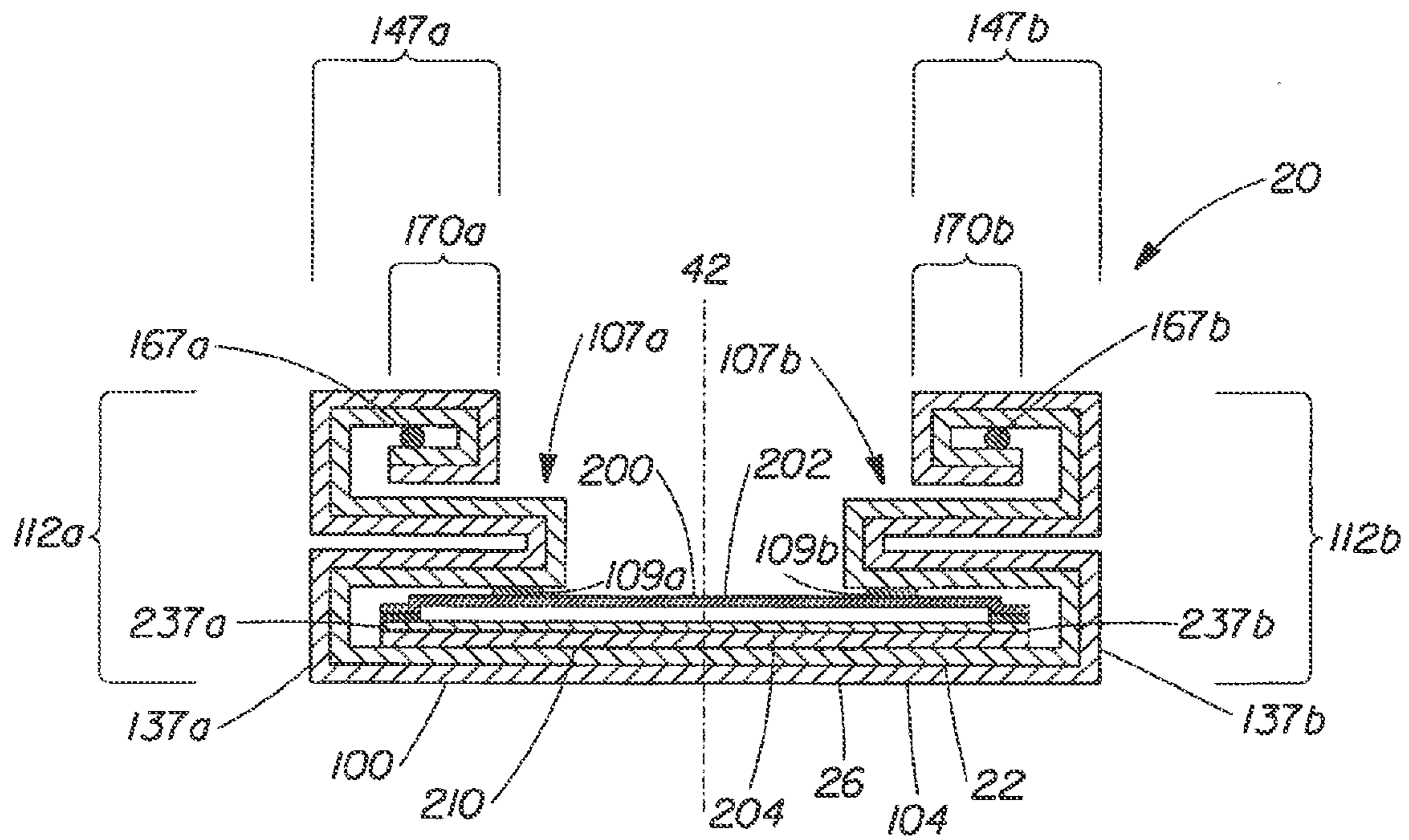
Fig. 21
