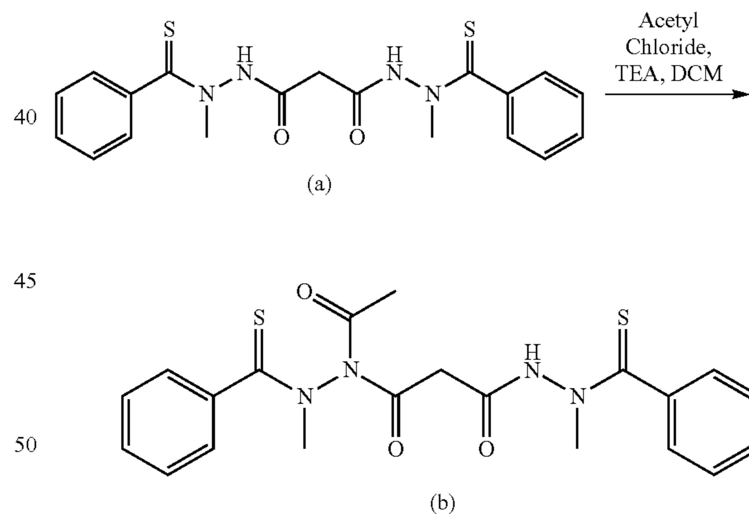
Scheme I:
