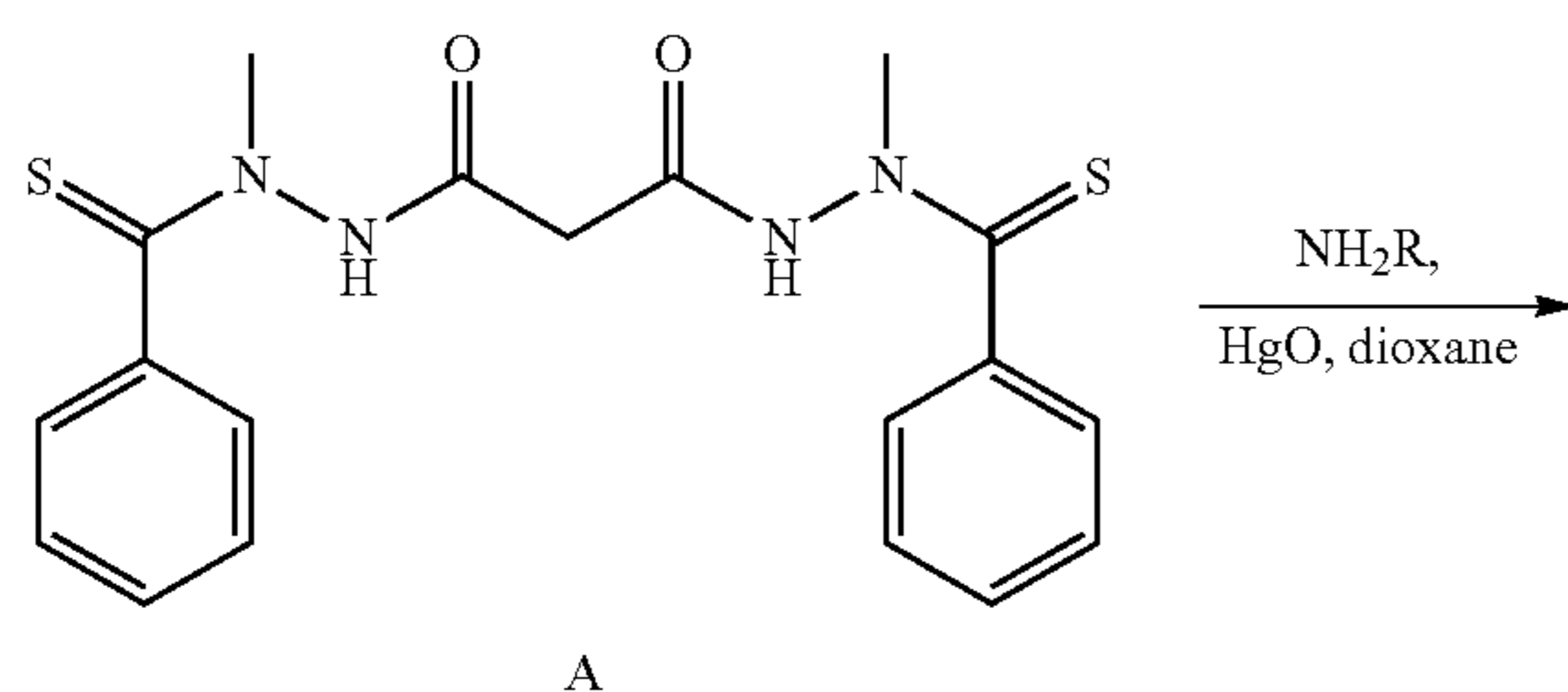
Scheme VI:
