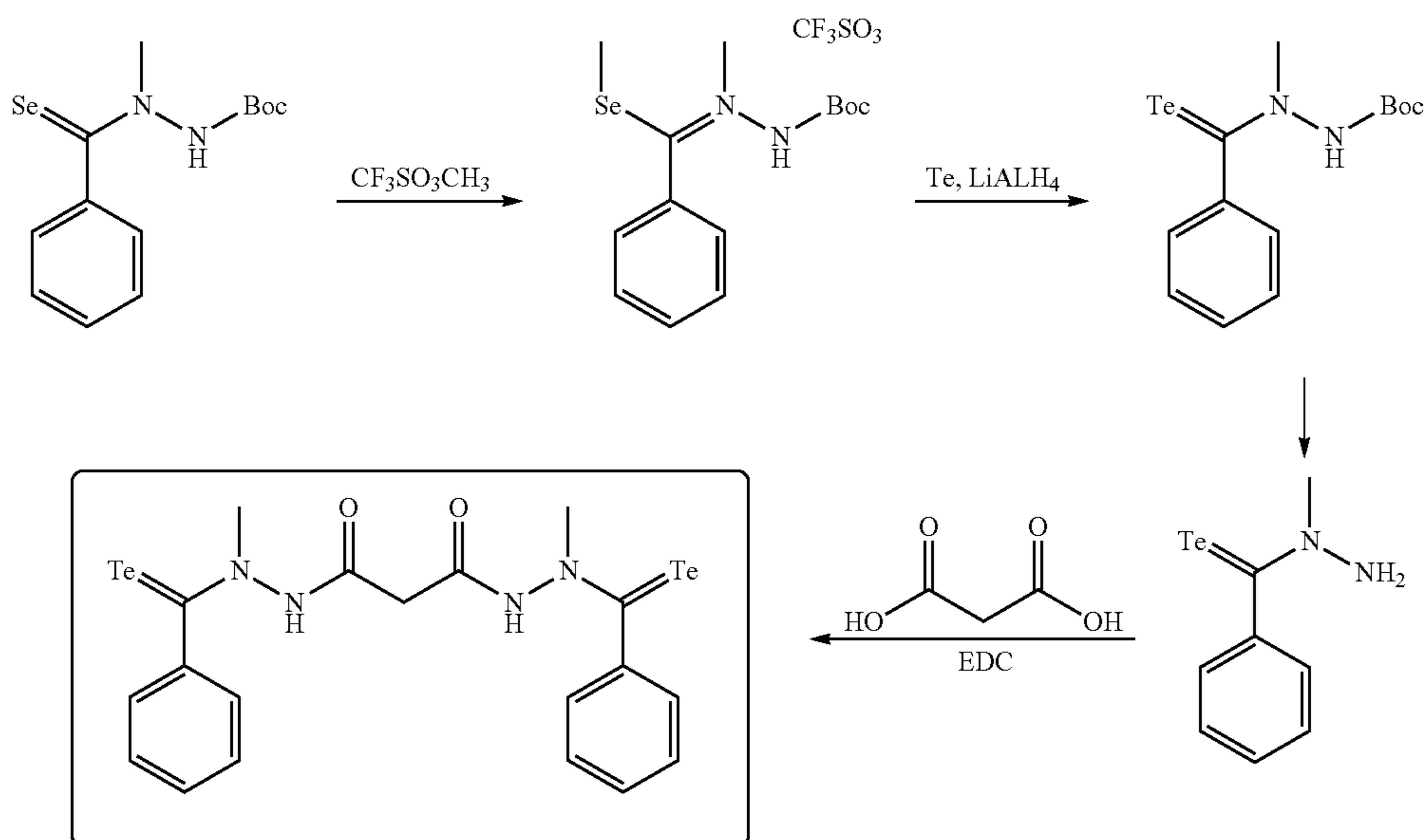
Scheme IV:
