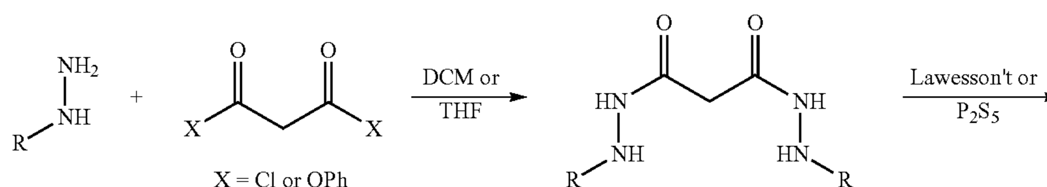
Scheme II:
