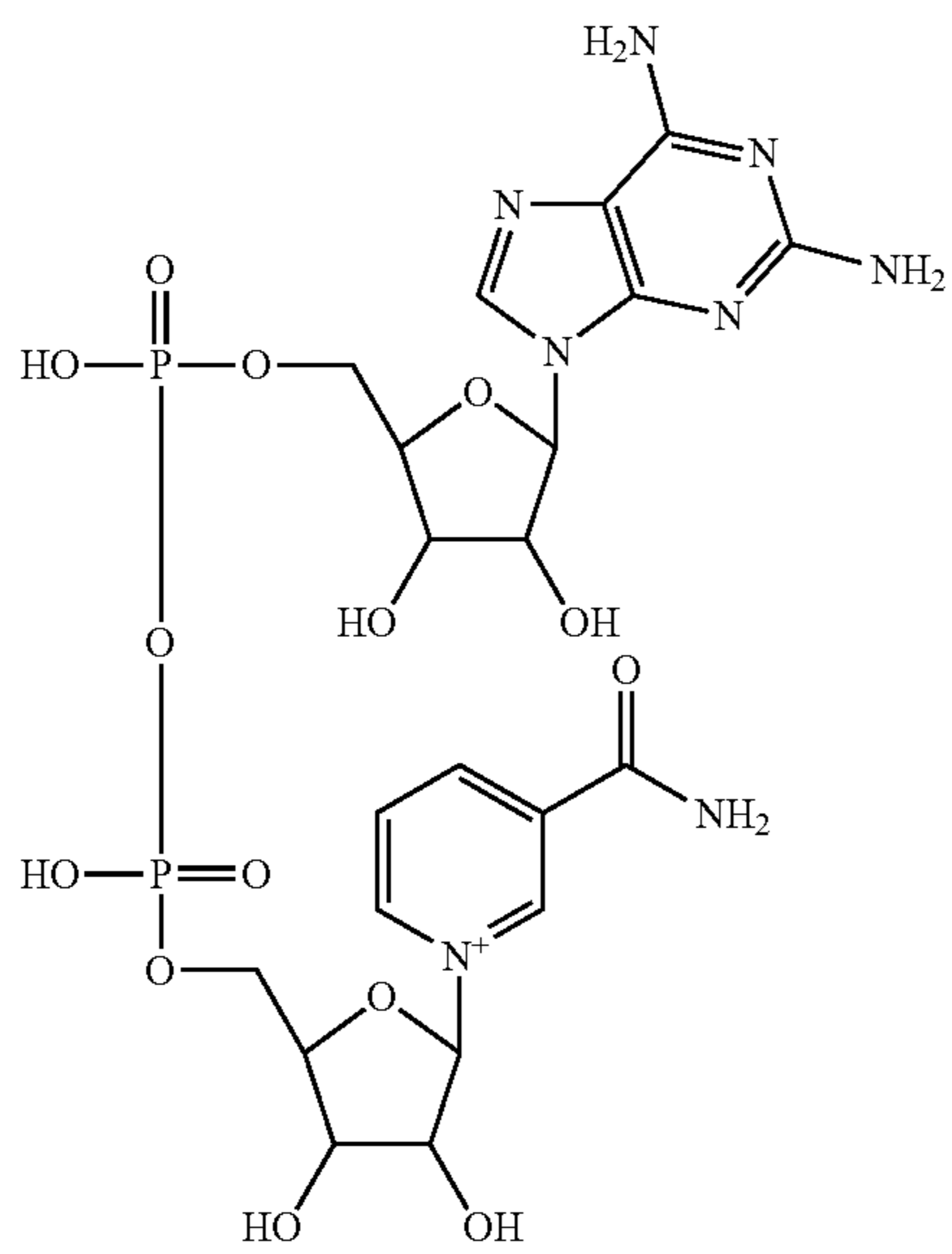
2-amino-NAD +
