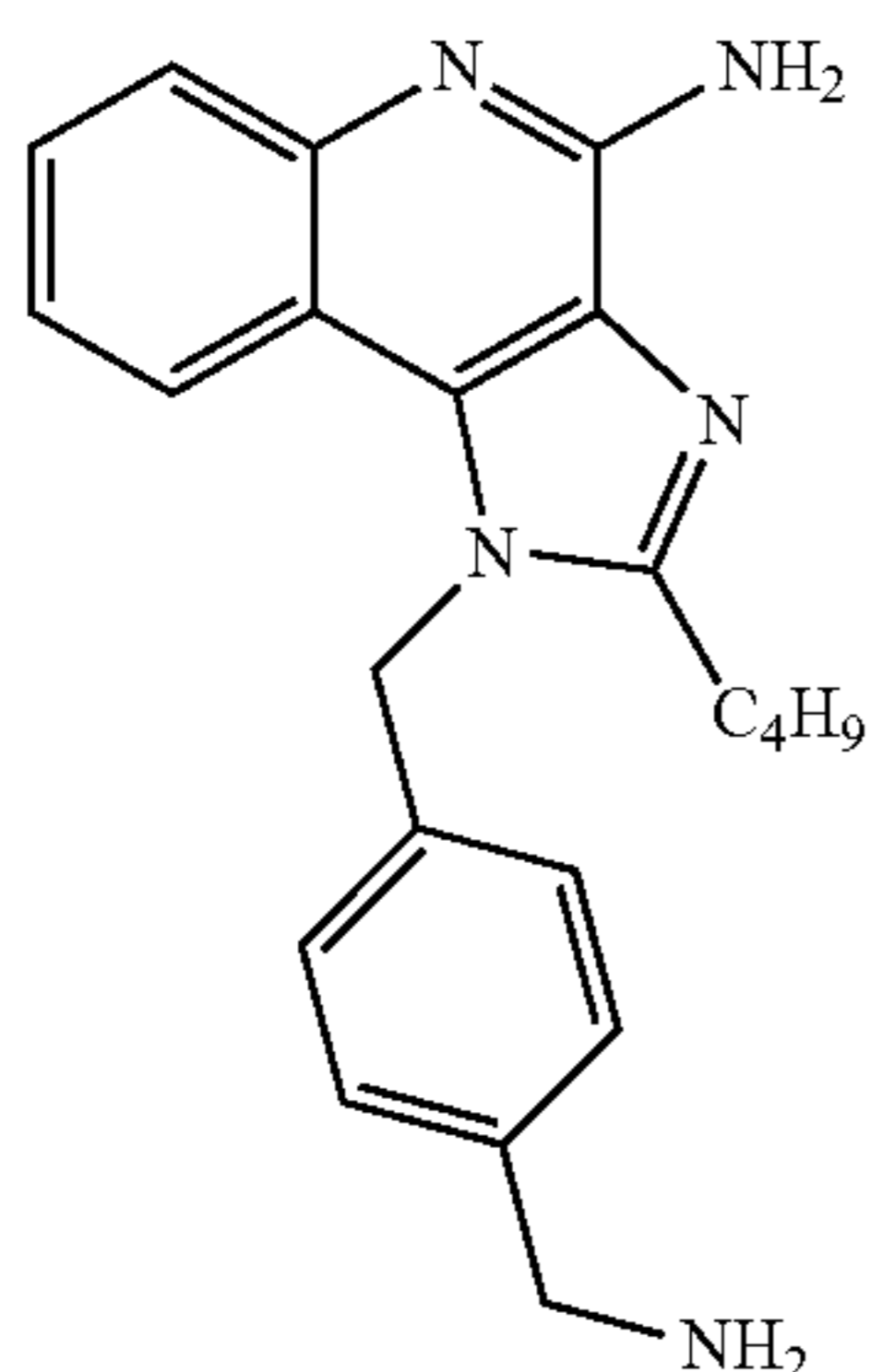
7d: 1-(4-(Aminomethyl)benzyl)-2-butyl-1H-imidazo [4,5-c]quinolin-4-amine
