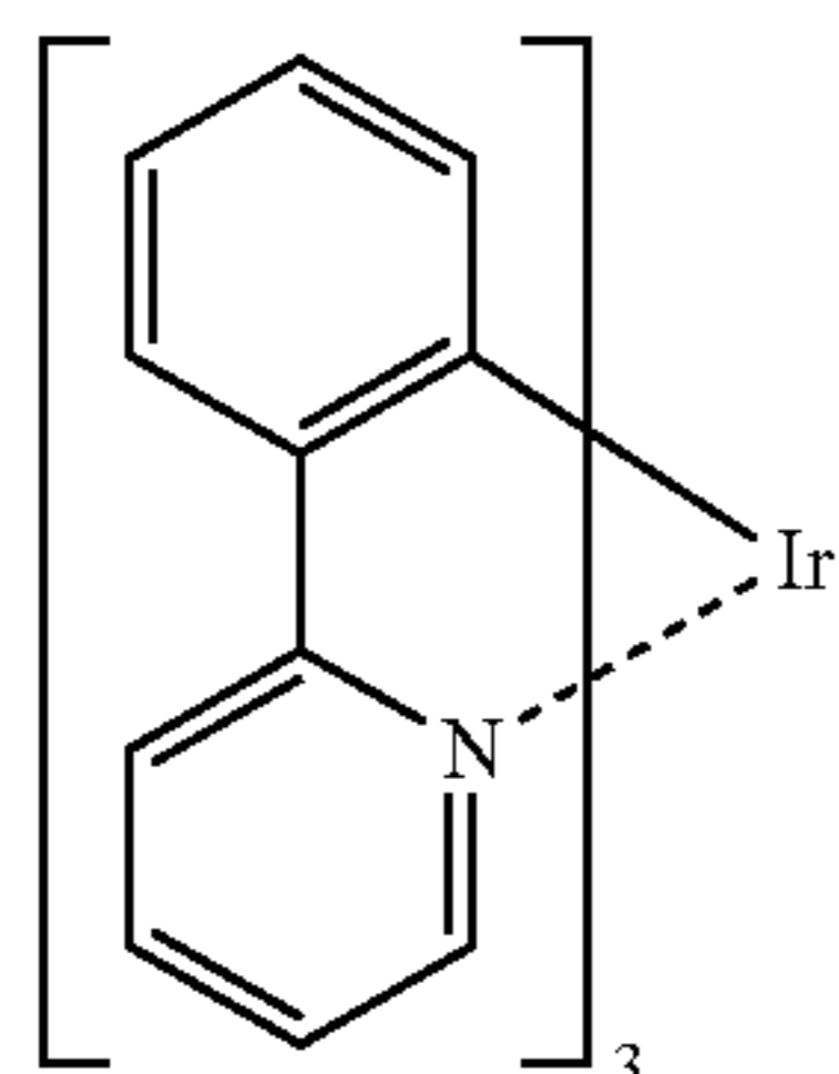
Ir(ppy) 3
