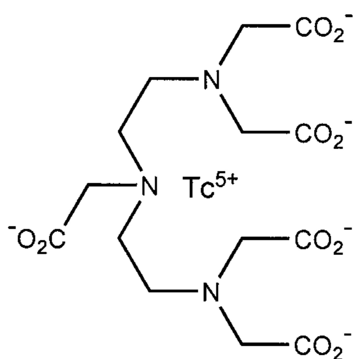
99m Tc-DTPA (3)
