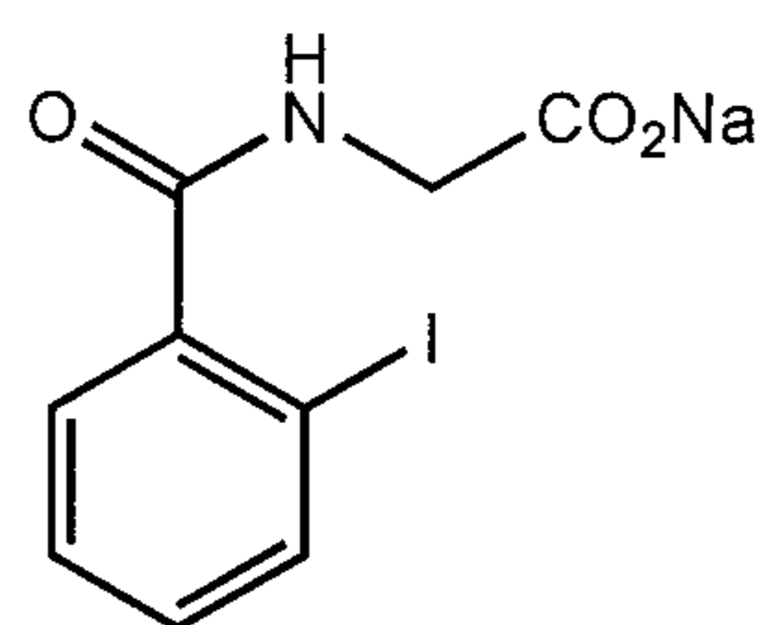
o-Iodohippurate (2)
