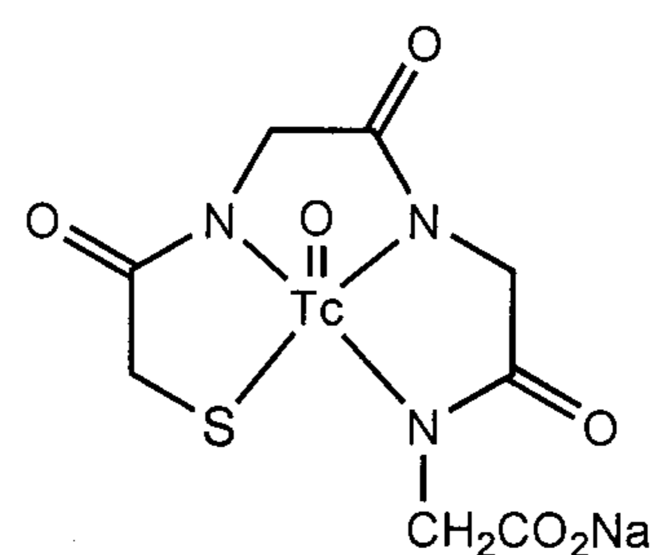
99m Tc-MAG3 (4)
