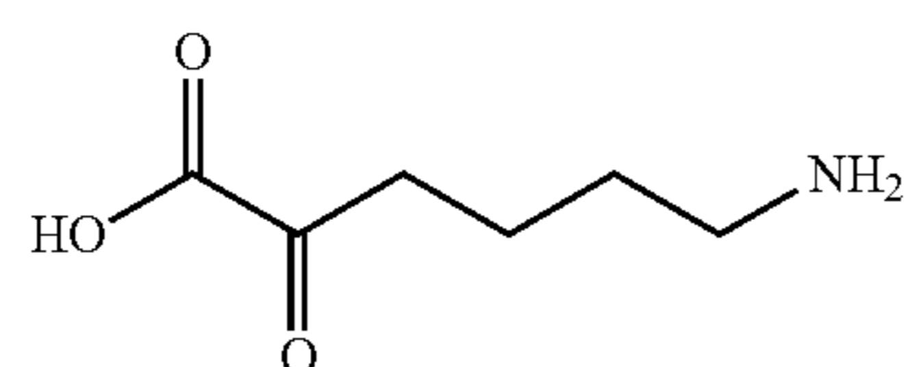
6-amino-2-oxohexanoic
