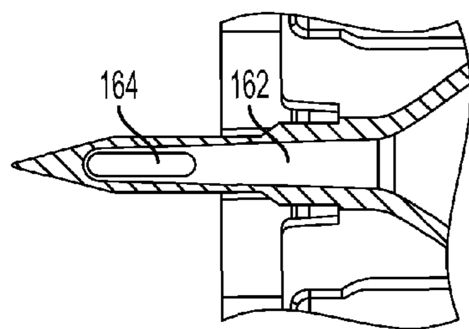
SECTION E - E FIG. 4E
