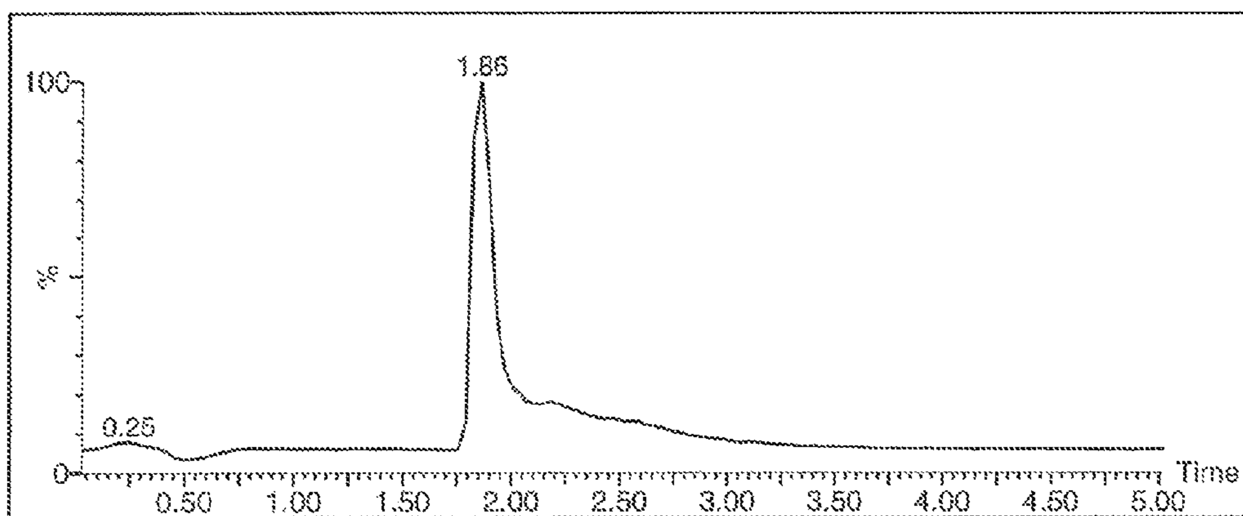
LC Trace - MOM-protected S-equol
