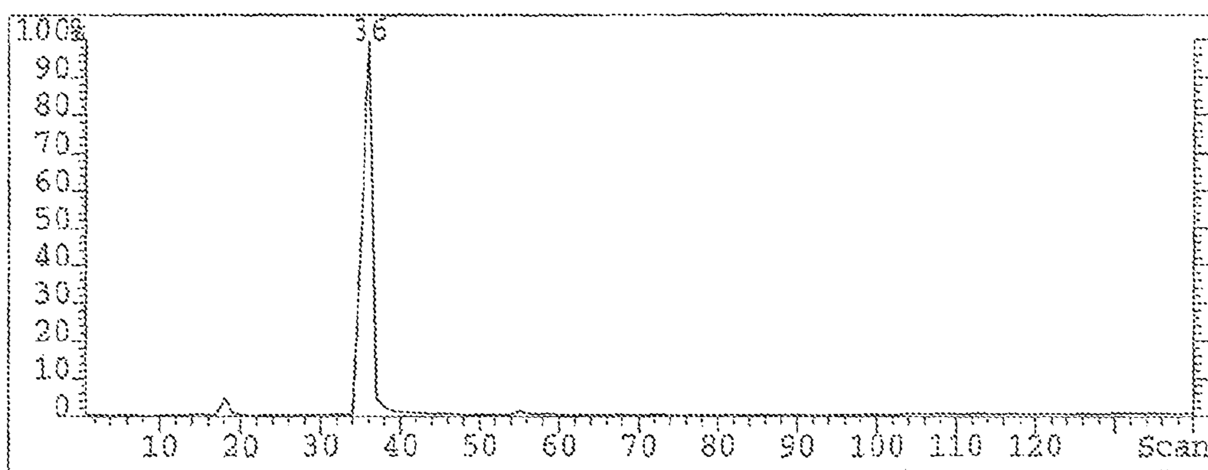
GC Trace - MOM-protected S-equol
