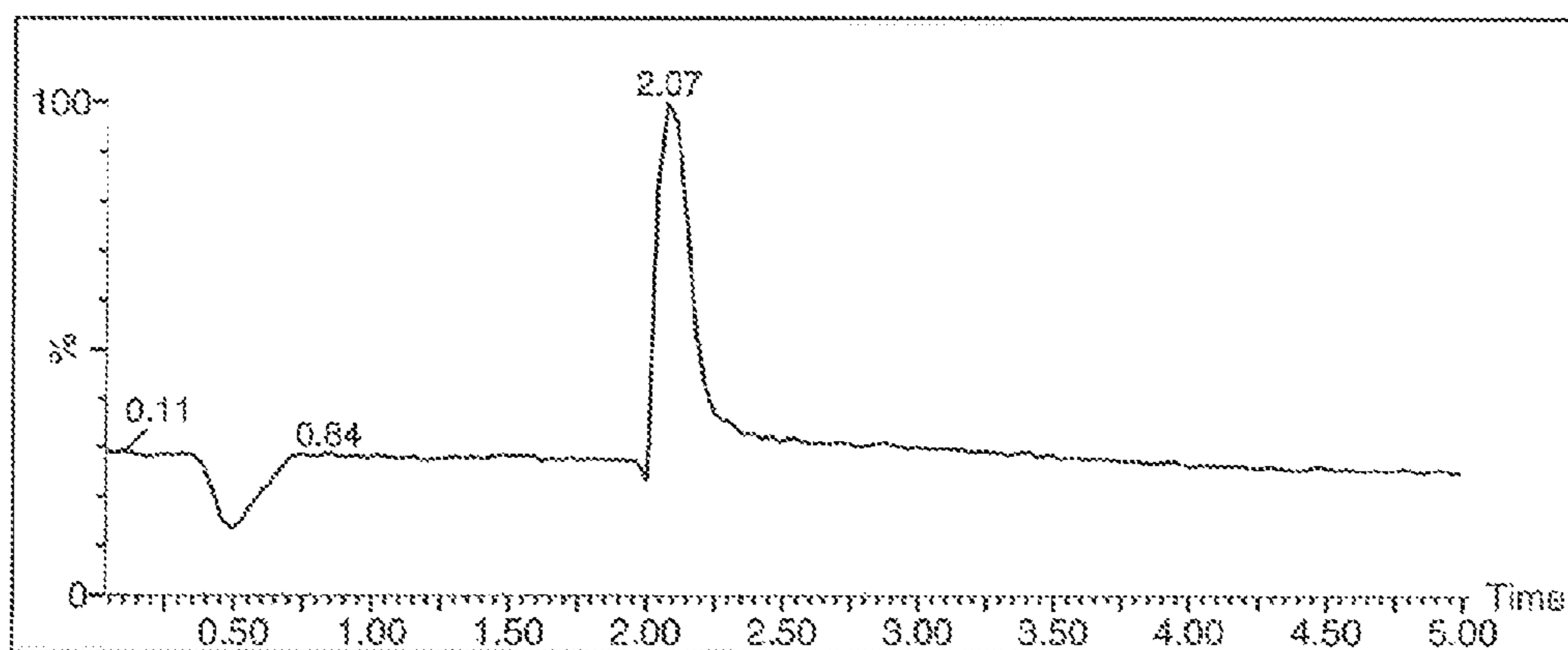
LC Trace - R-Equol
