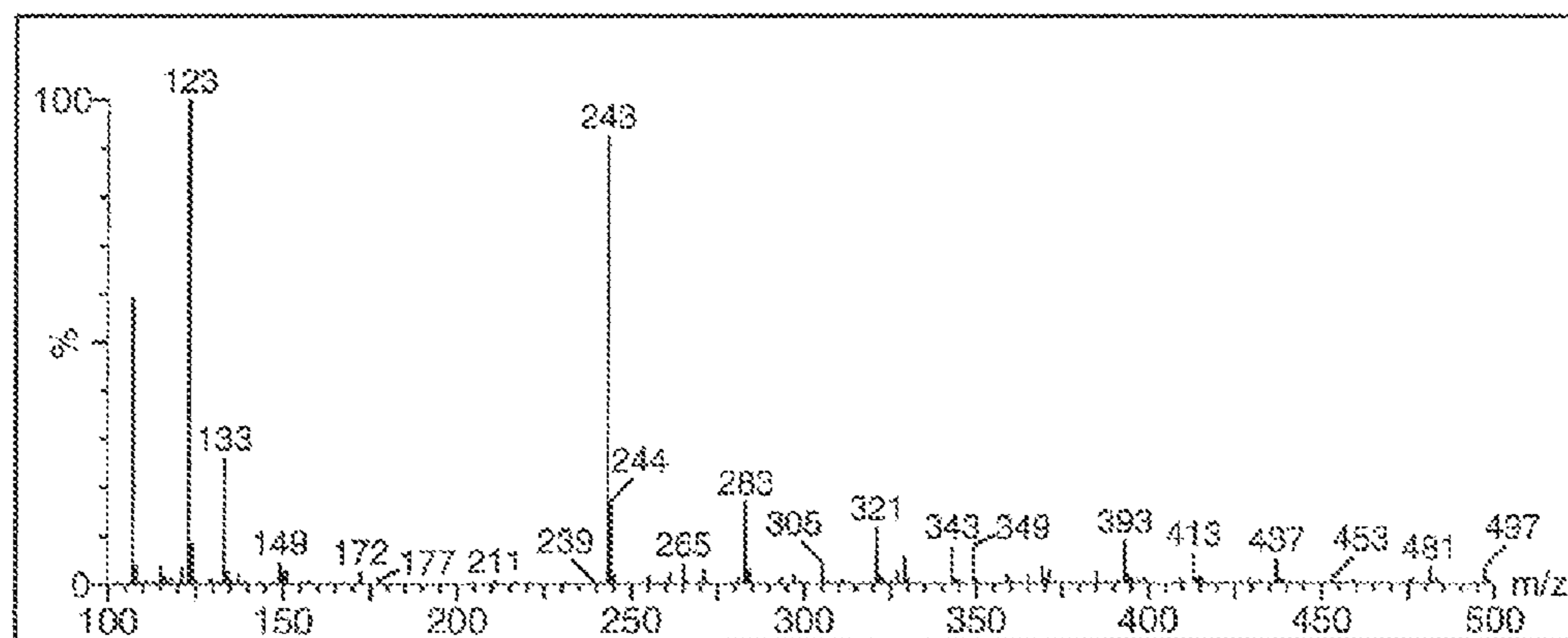
Spectrum - R-Equol
