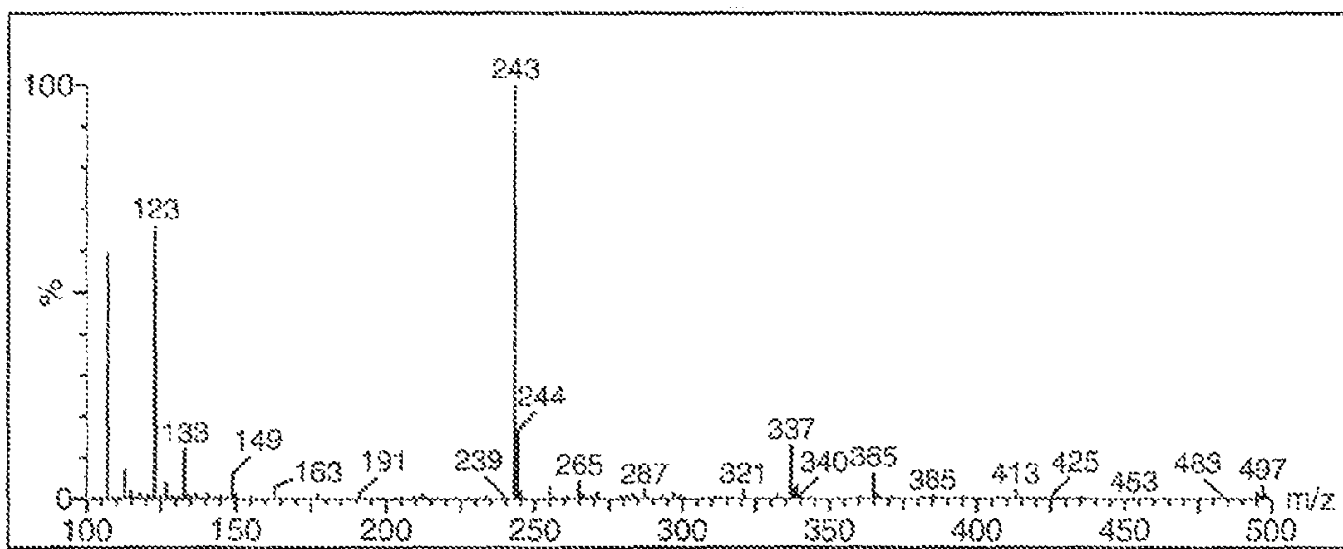
Spectrum - S-Equol
