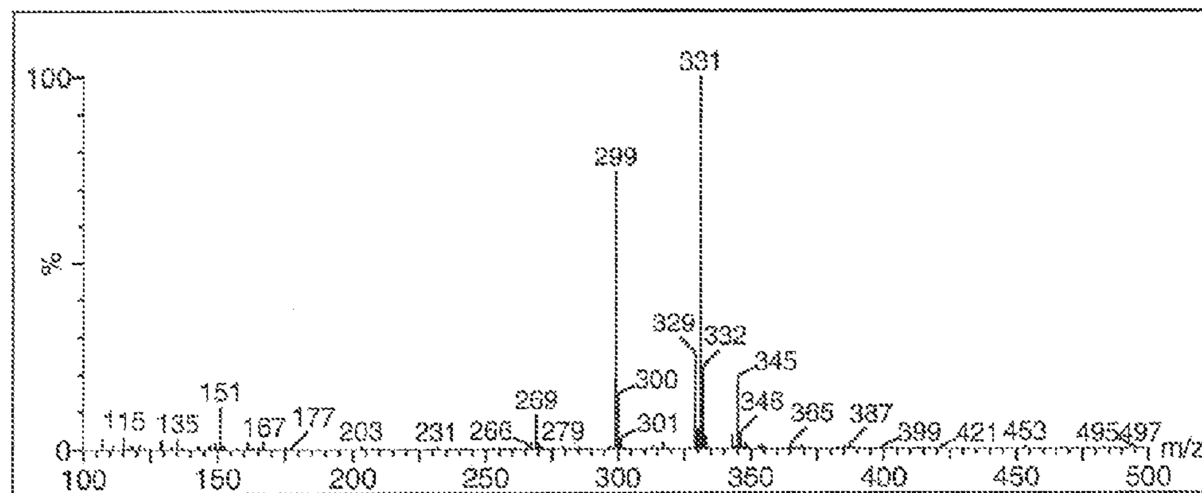
Spectrum - MOM-protected R-equol
