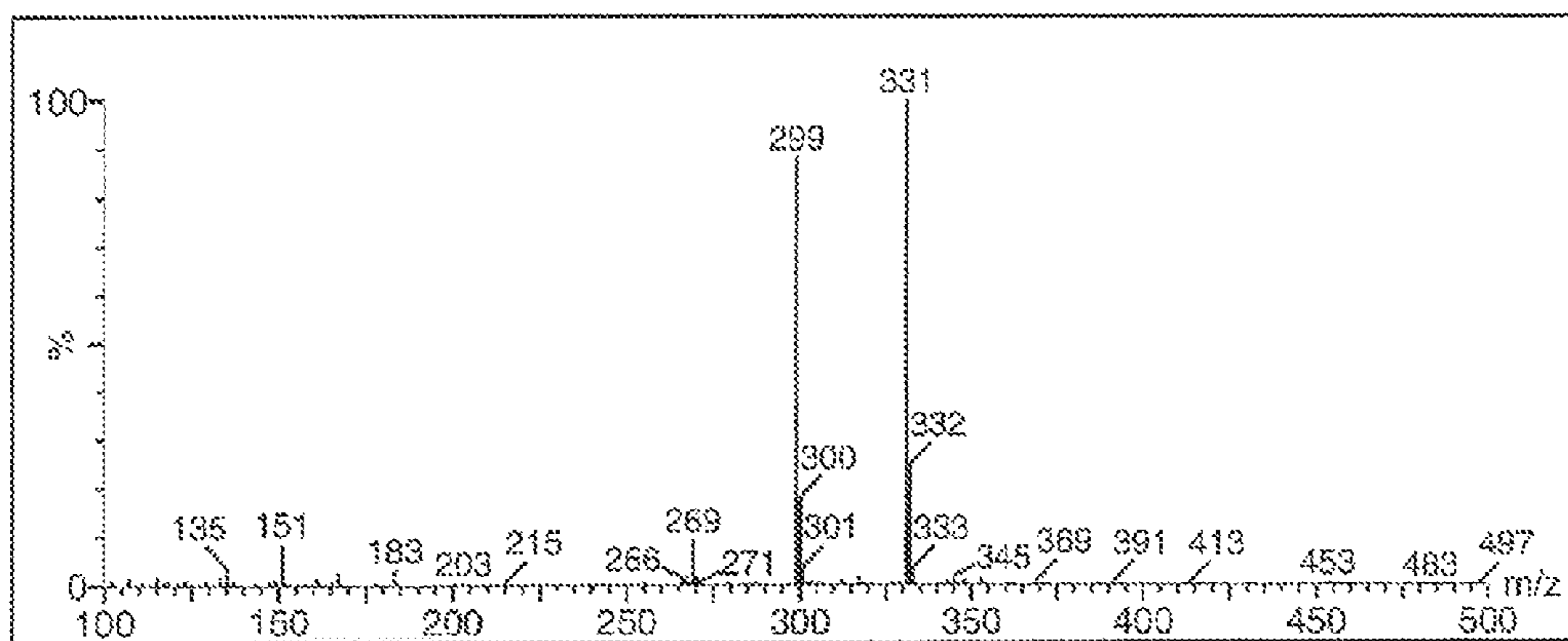
Spectrum - MOM-protected S-equol
