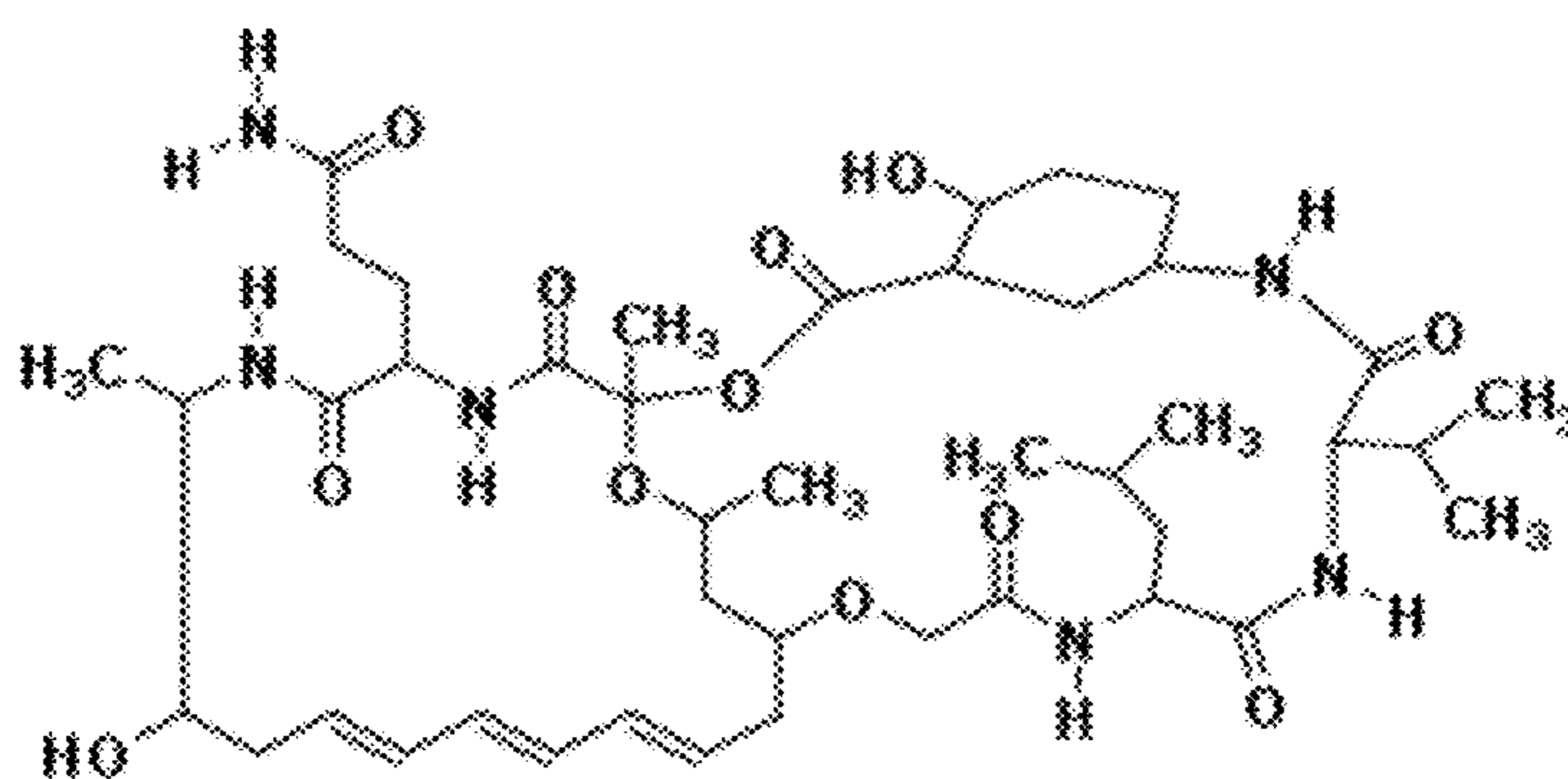
Chromamide A (1)
