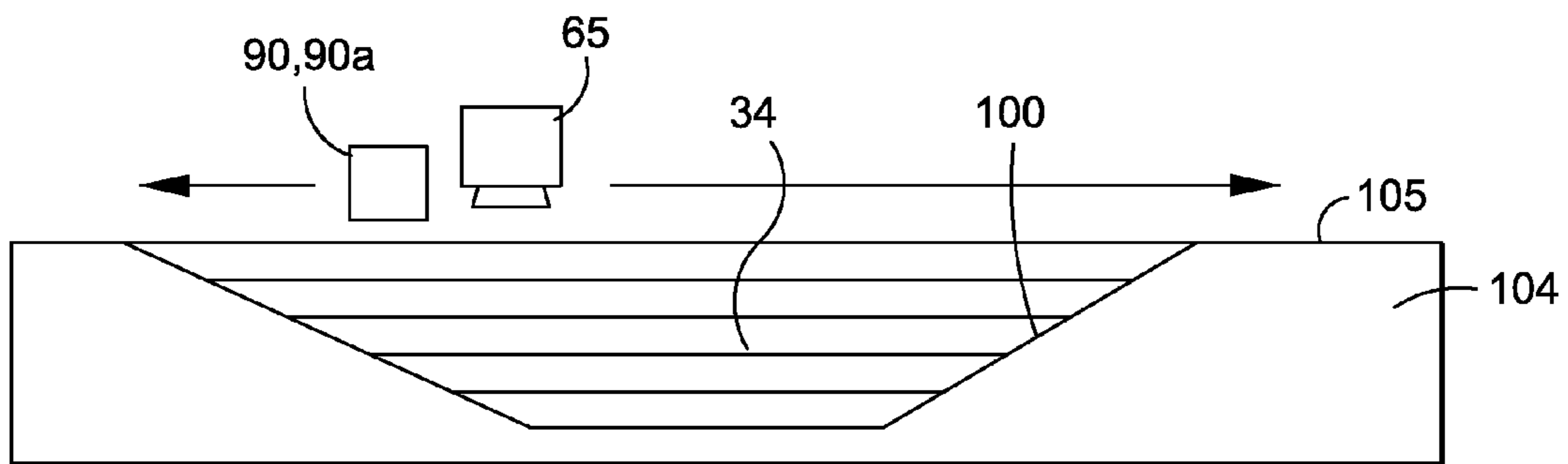
FIG. 8M
