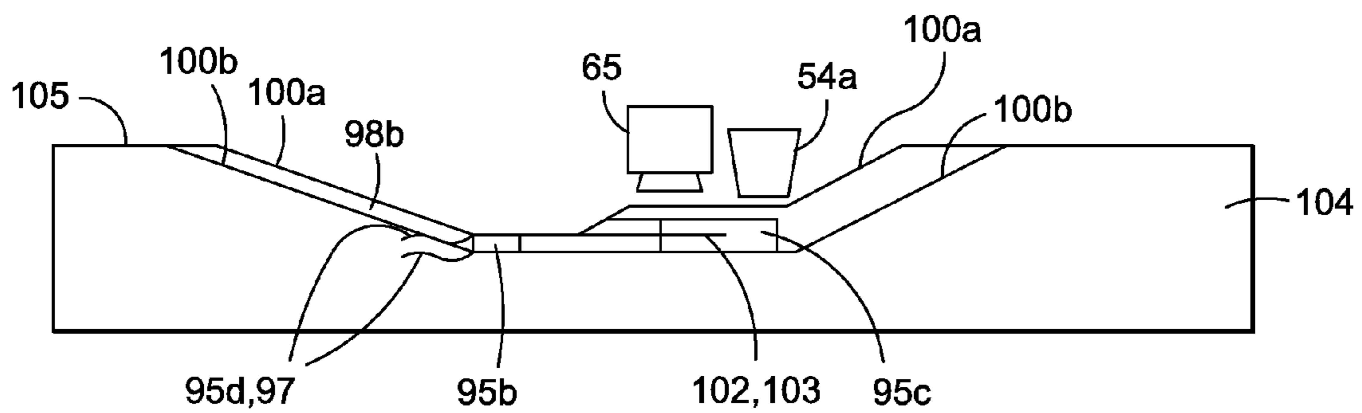
FIG. 8F
