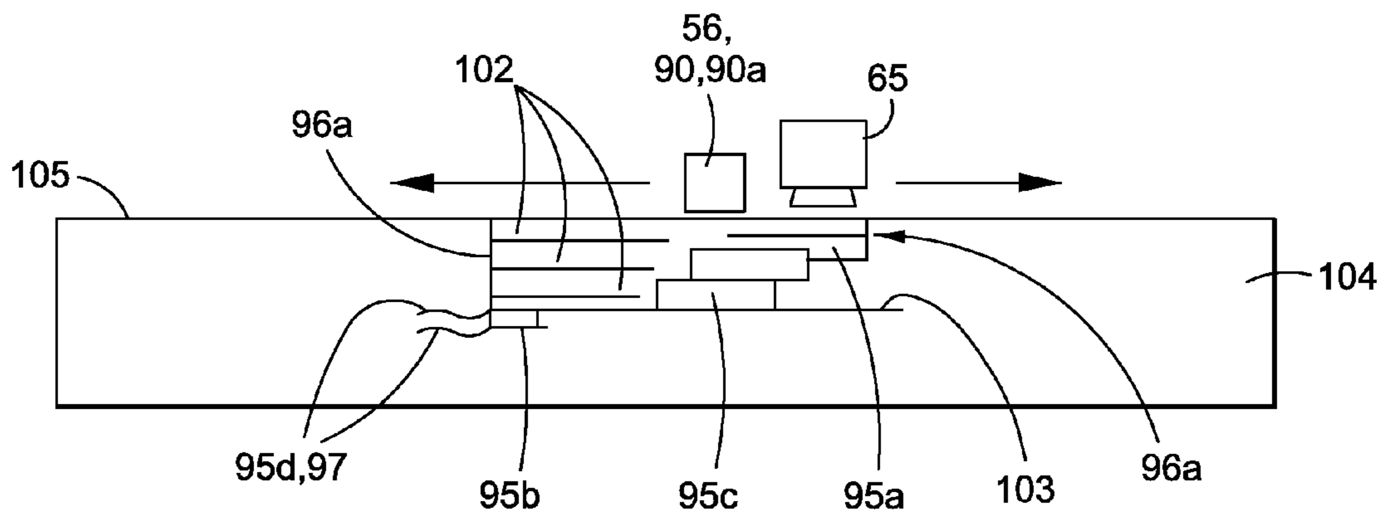
FIG. 8B
