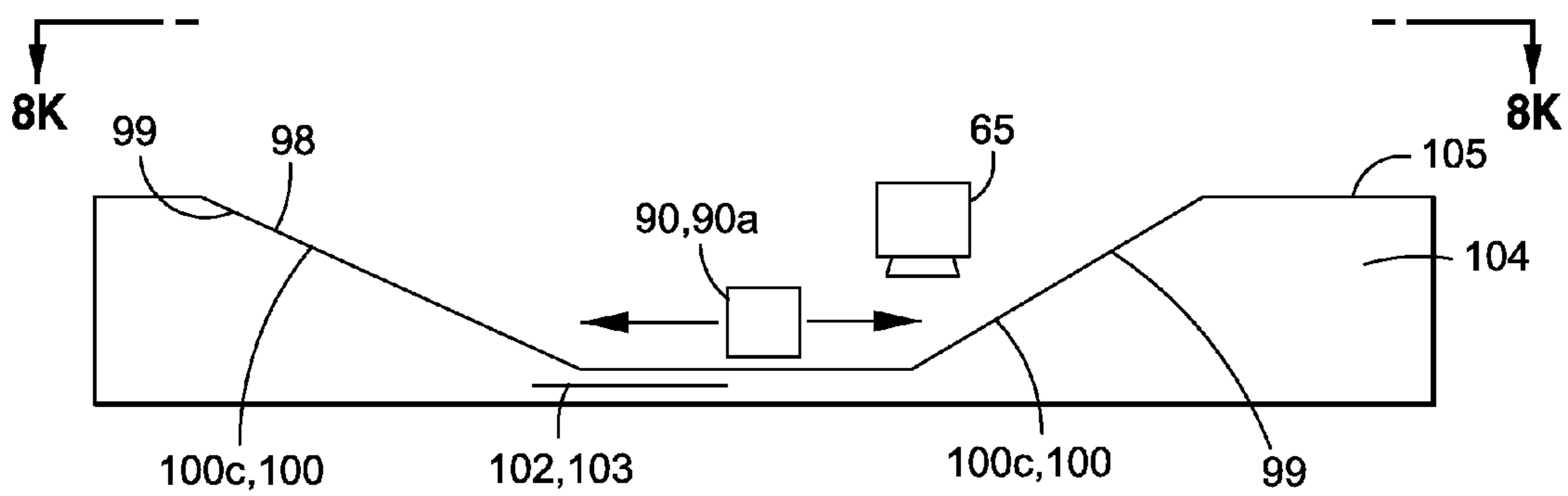
FIG. 8J
