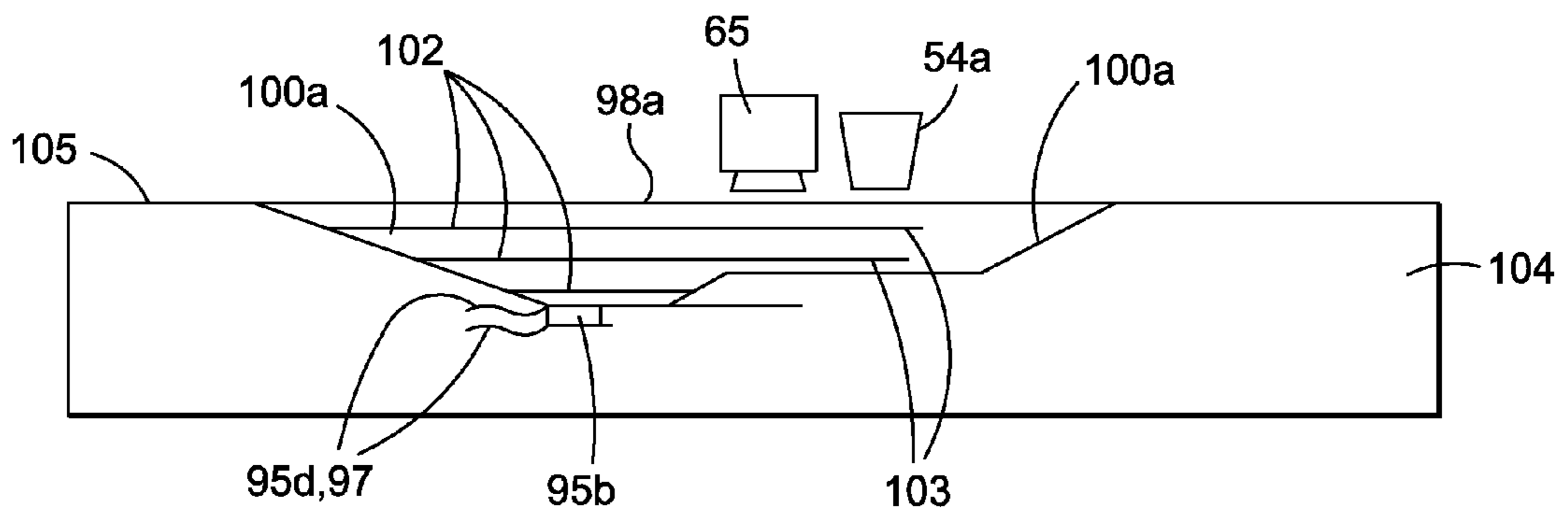
FIG. 8C
