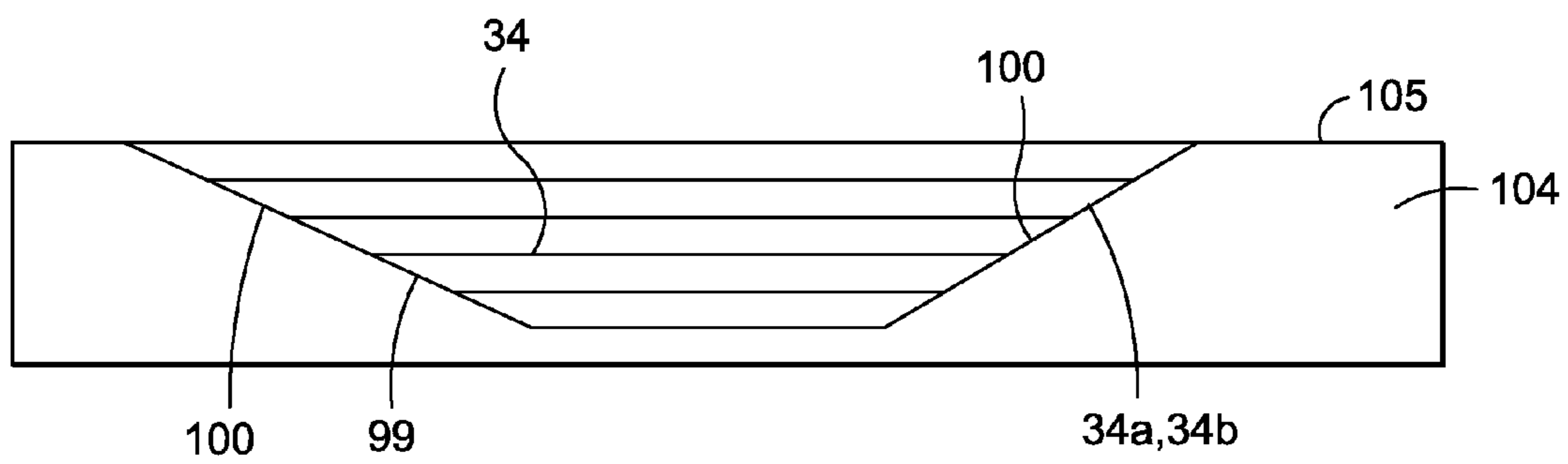
FIG. 8L
