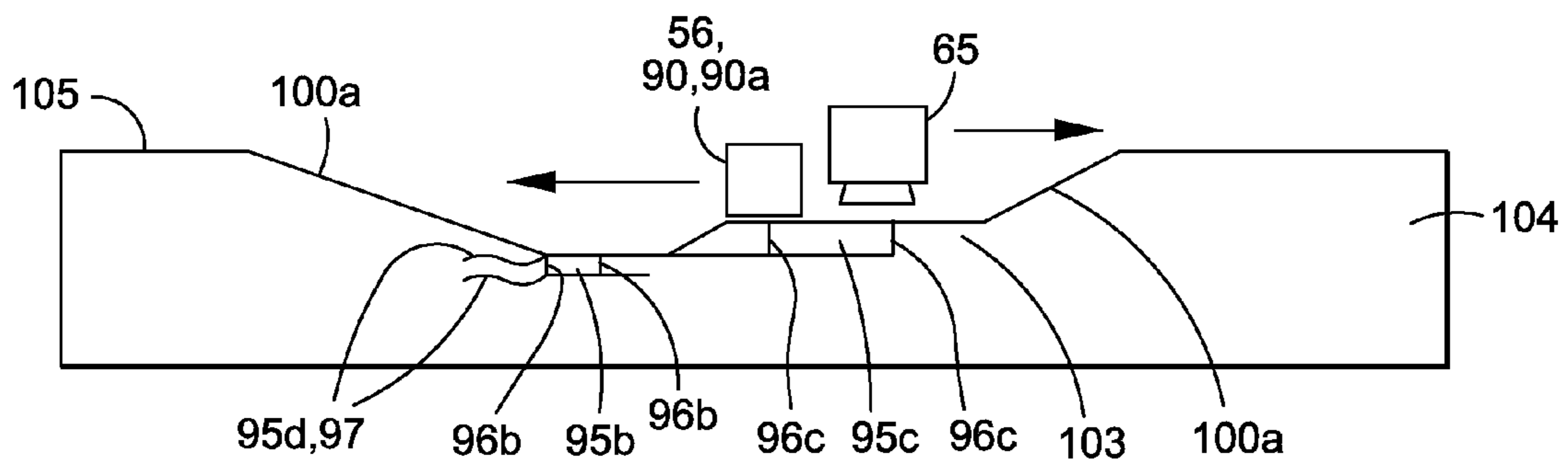
FIG. 8E
