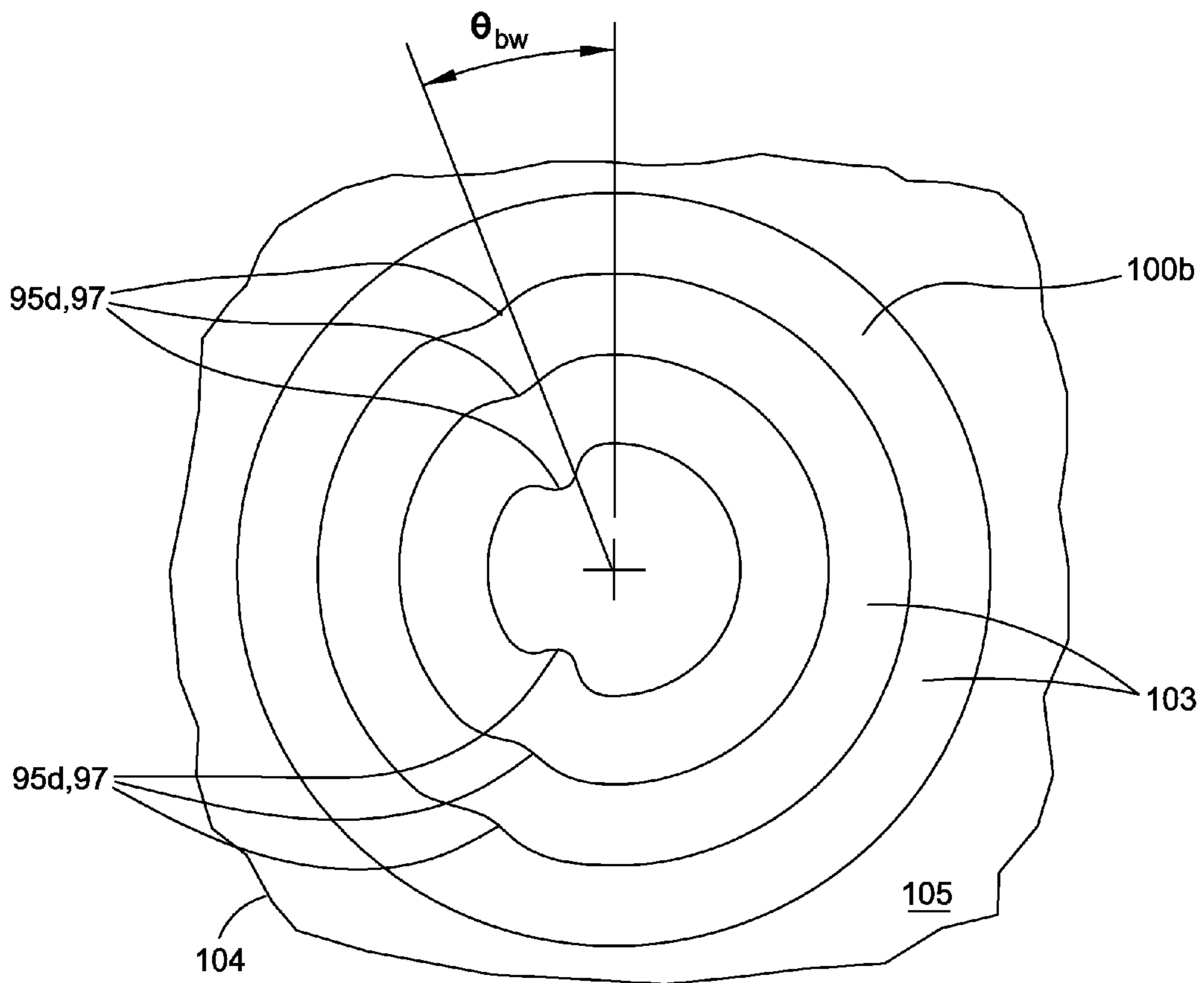
FIG. 8H
