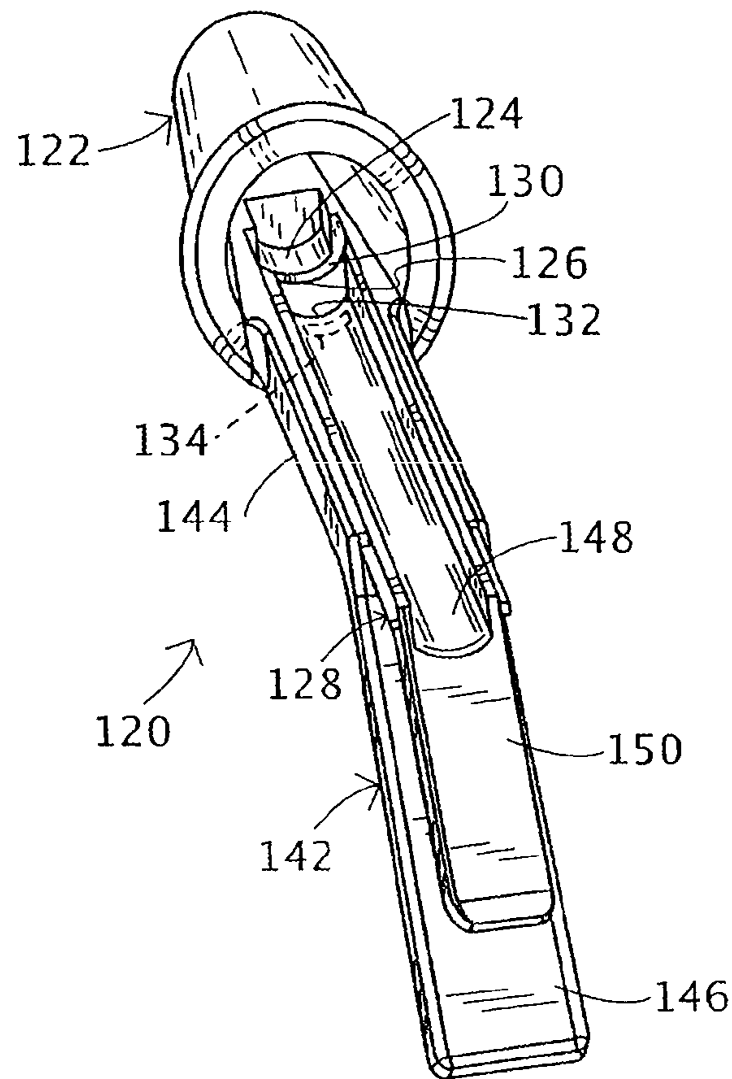
FIG. 15
