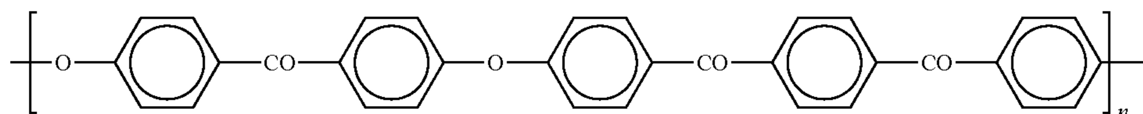
PEKEKK
