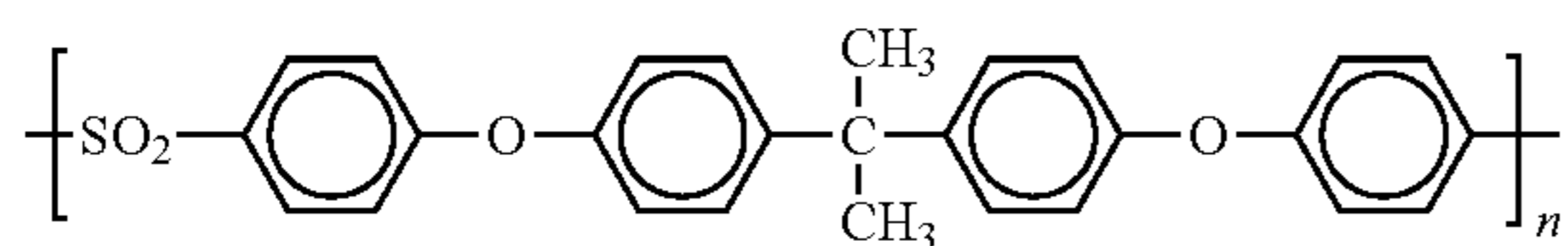
®Udel
