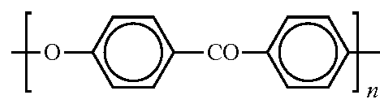
PEK
