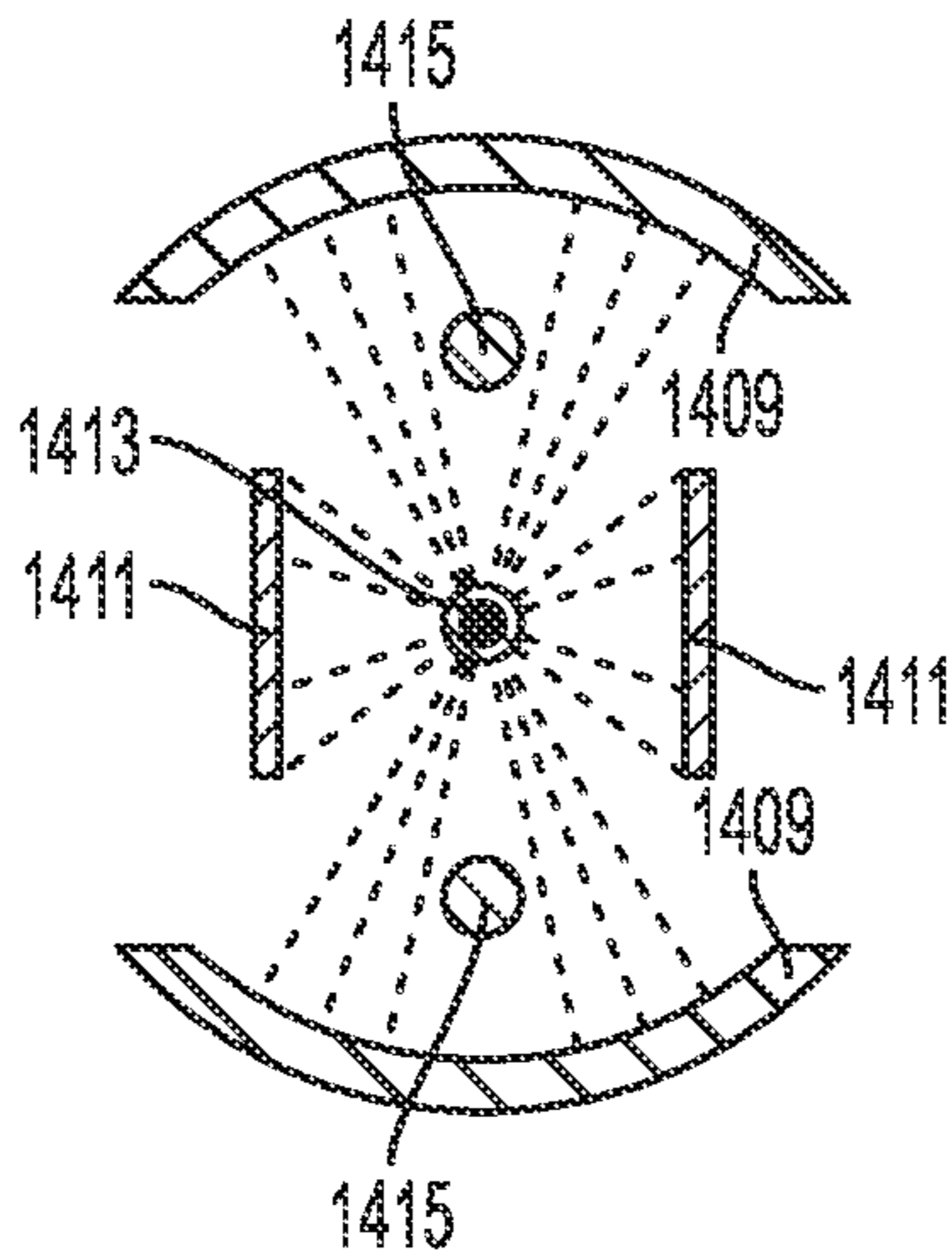
FIG. 14B
