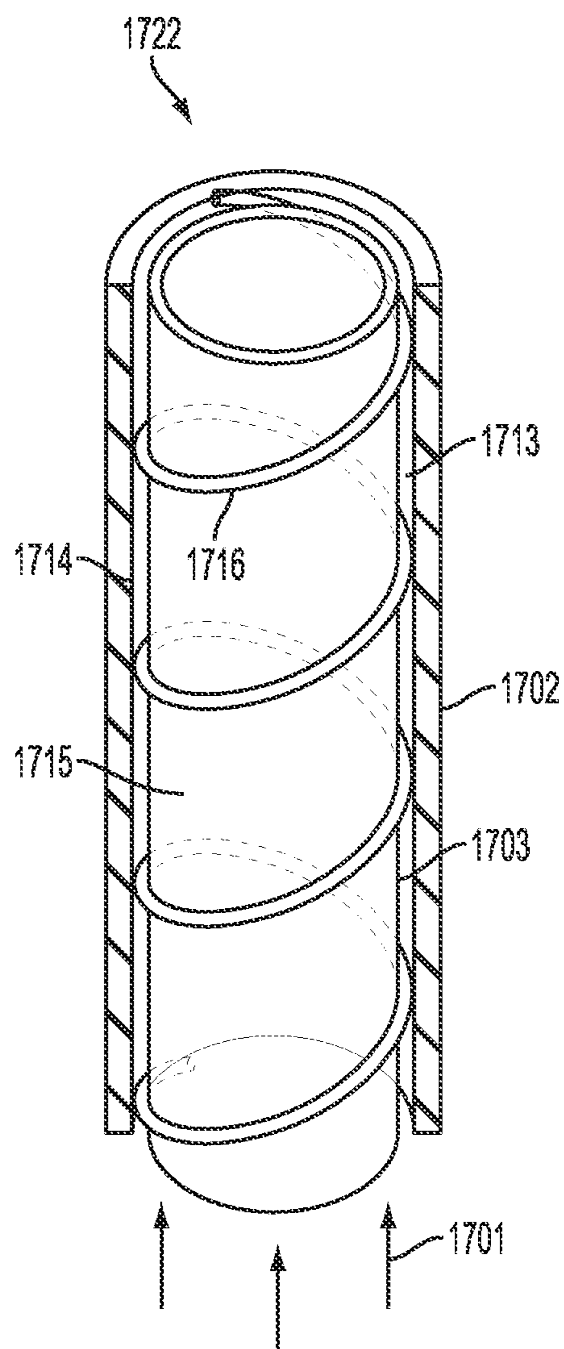
FIG. 17
