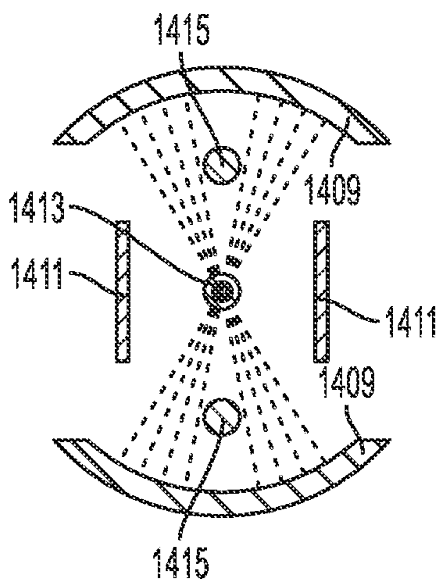
FIG. 14C
