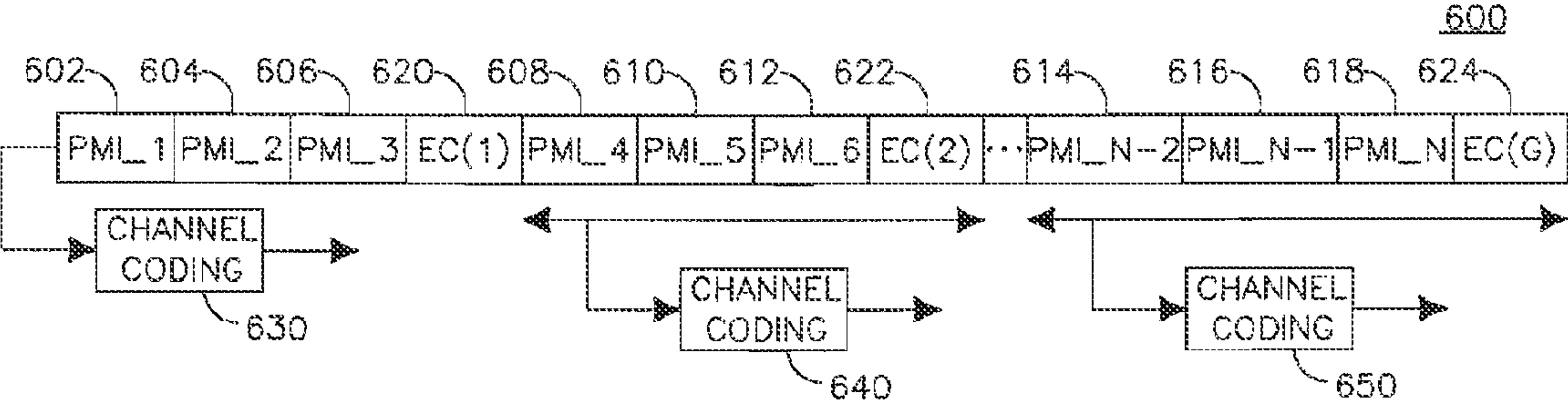
FIG. 6
