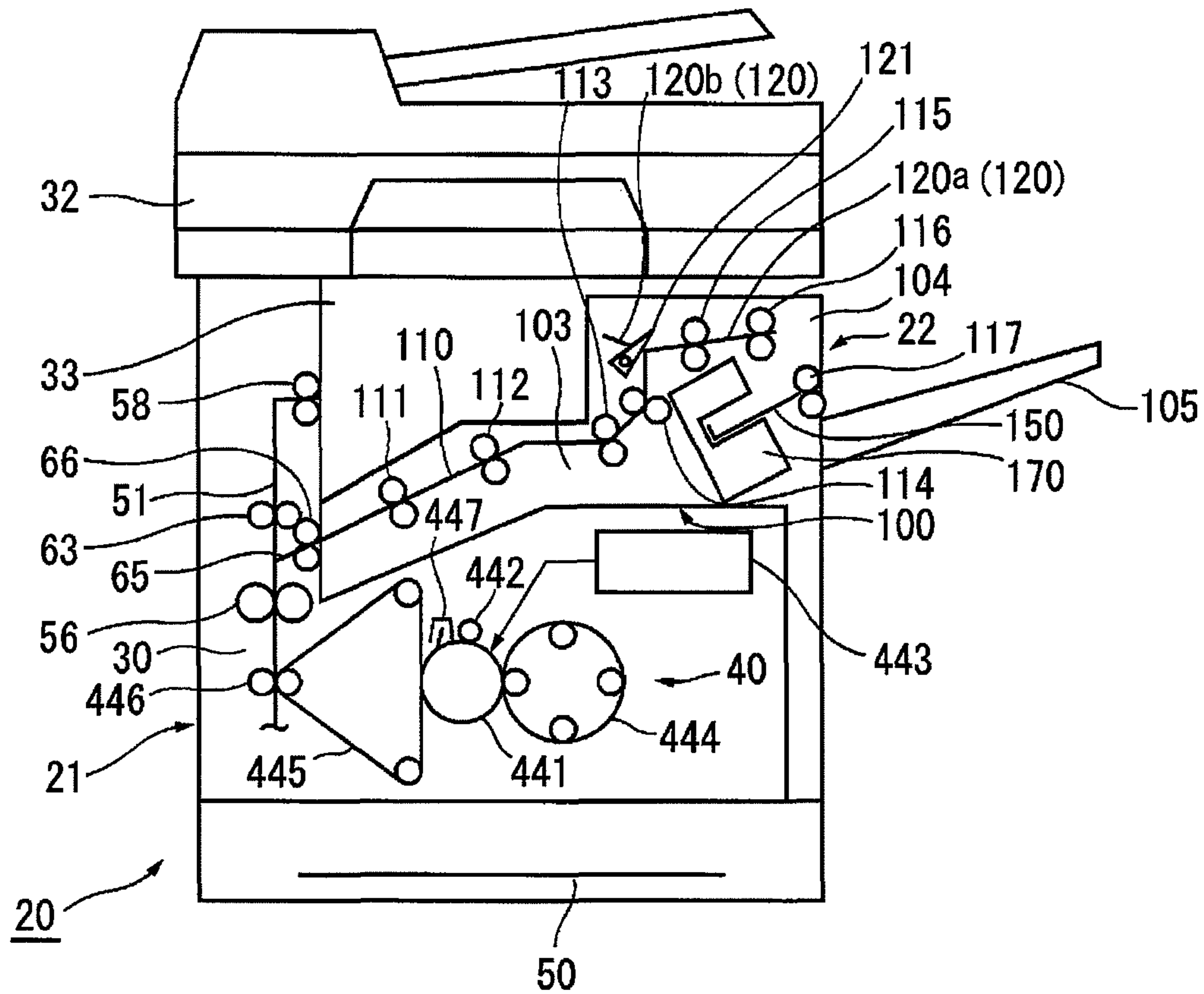
FIG. 18C
