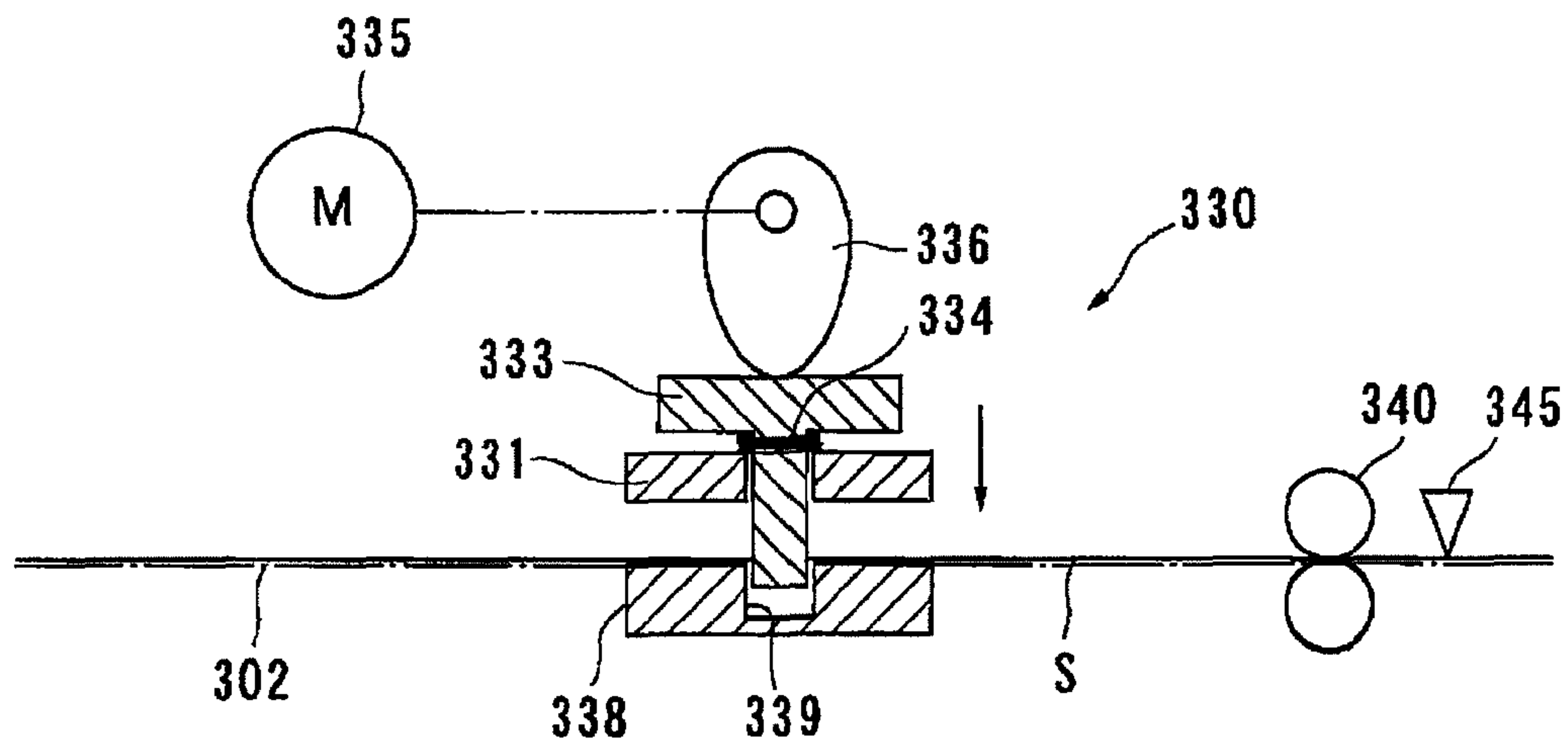
FIG. 10B
