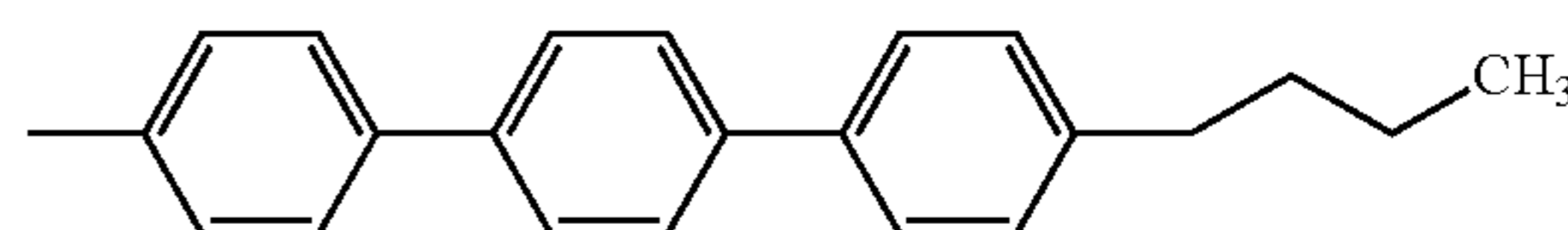
4-butyl-[1,1';4',1'']terphenyl-4-yl
