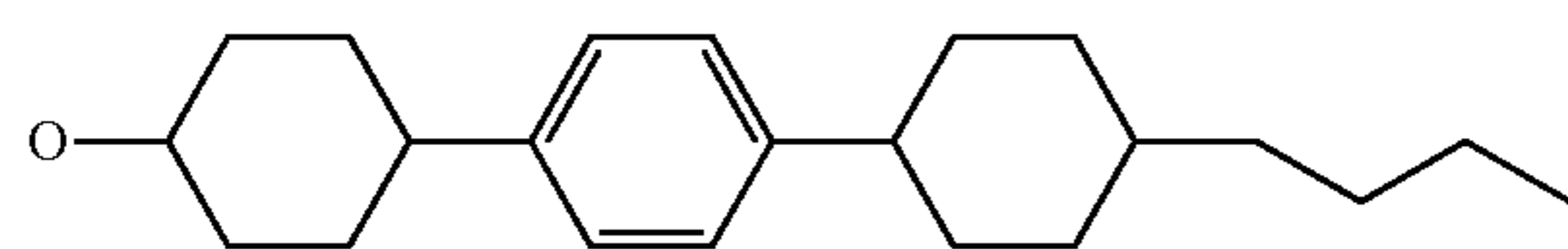
4-[4-(4-butyl-cyclohexyl)-phenyl]-cyclohexyloxy
