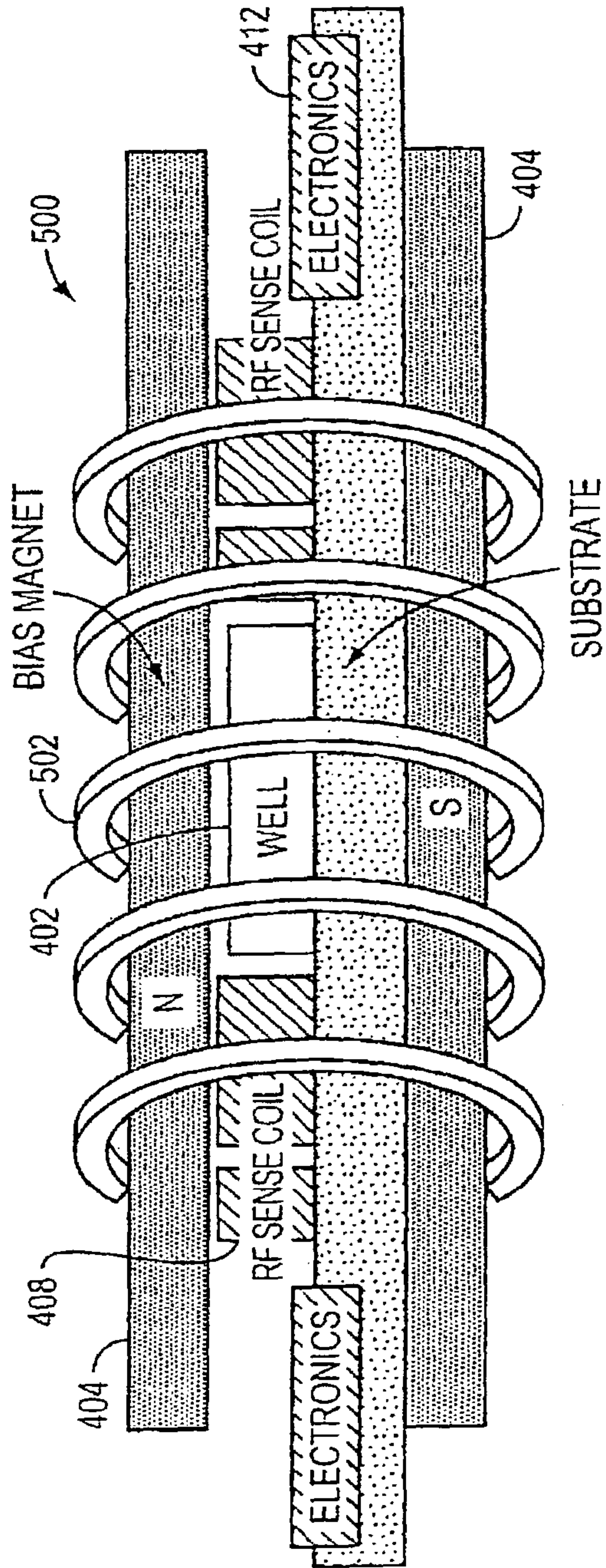
FIG. 5A
