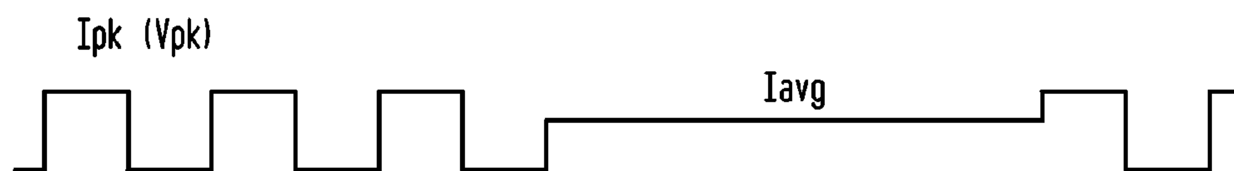
FIG. 9 FORWARD BIASING (V OR I)
