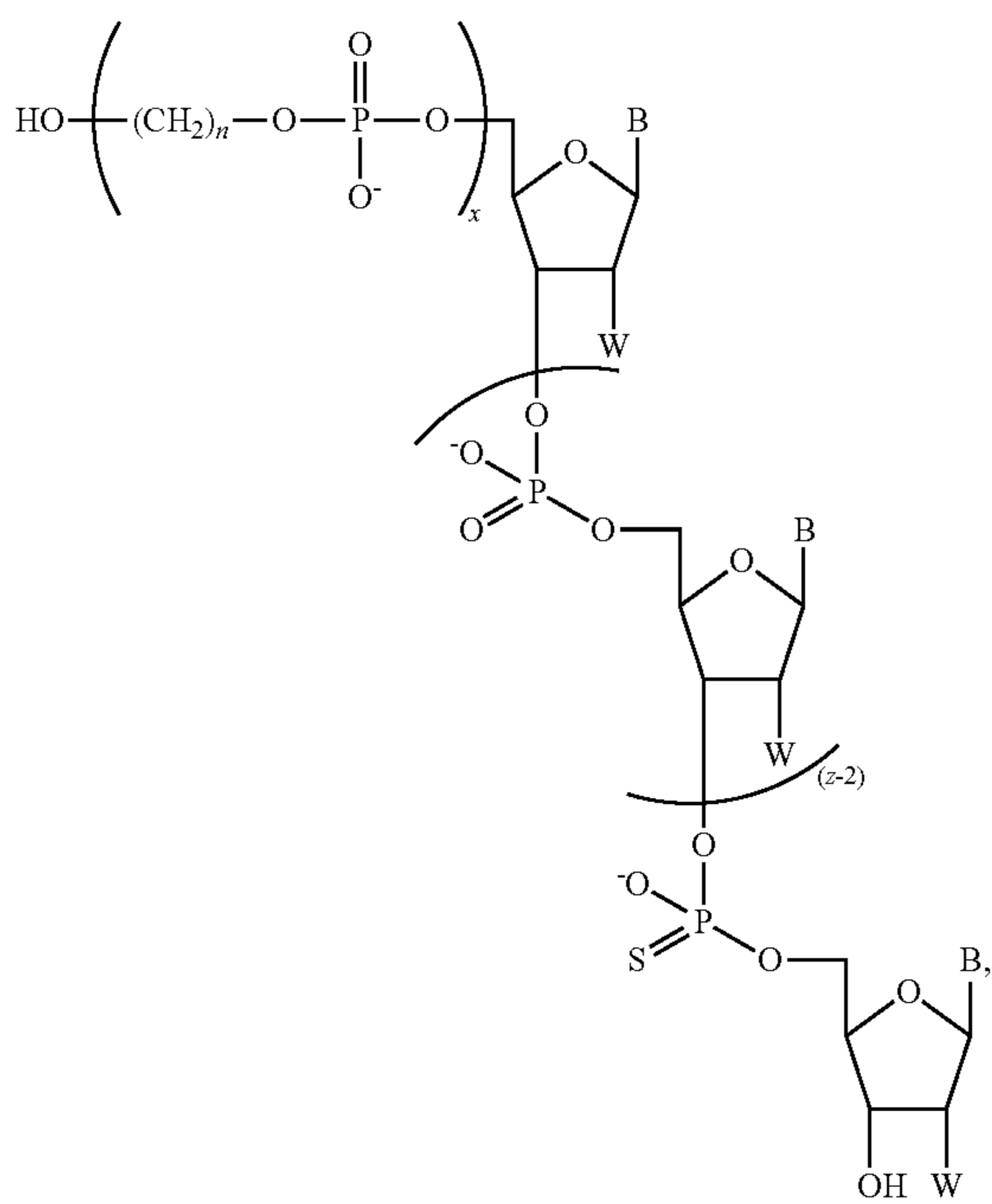
Formula I-A
