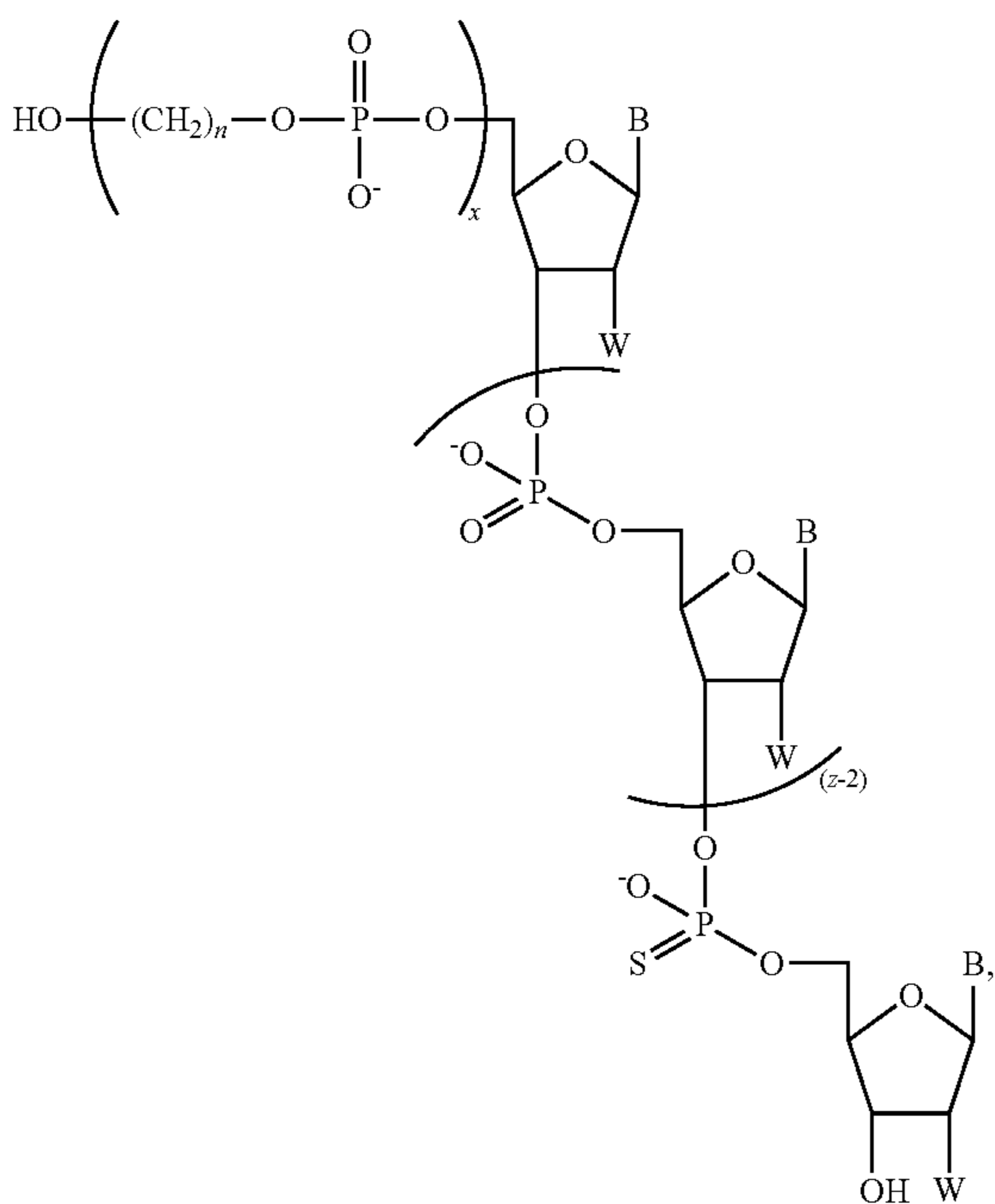
Formula I-A
