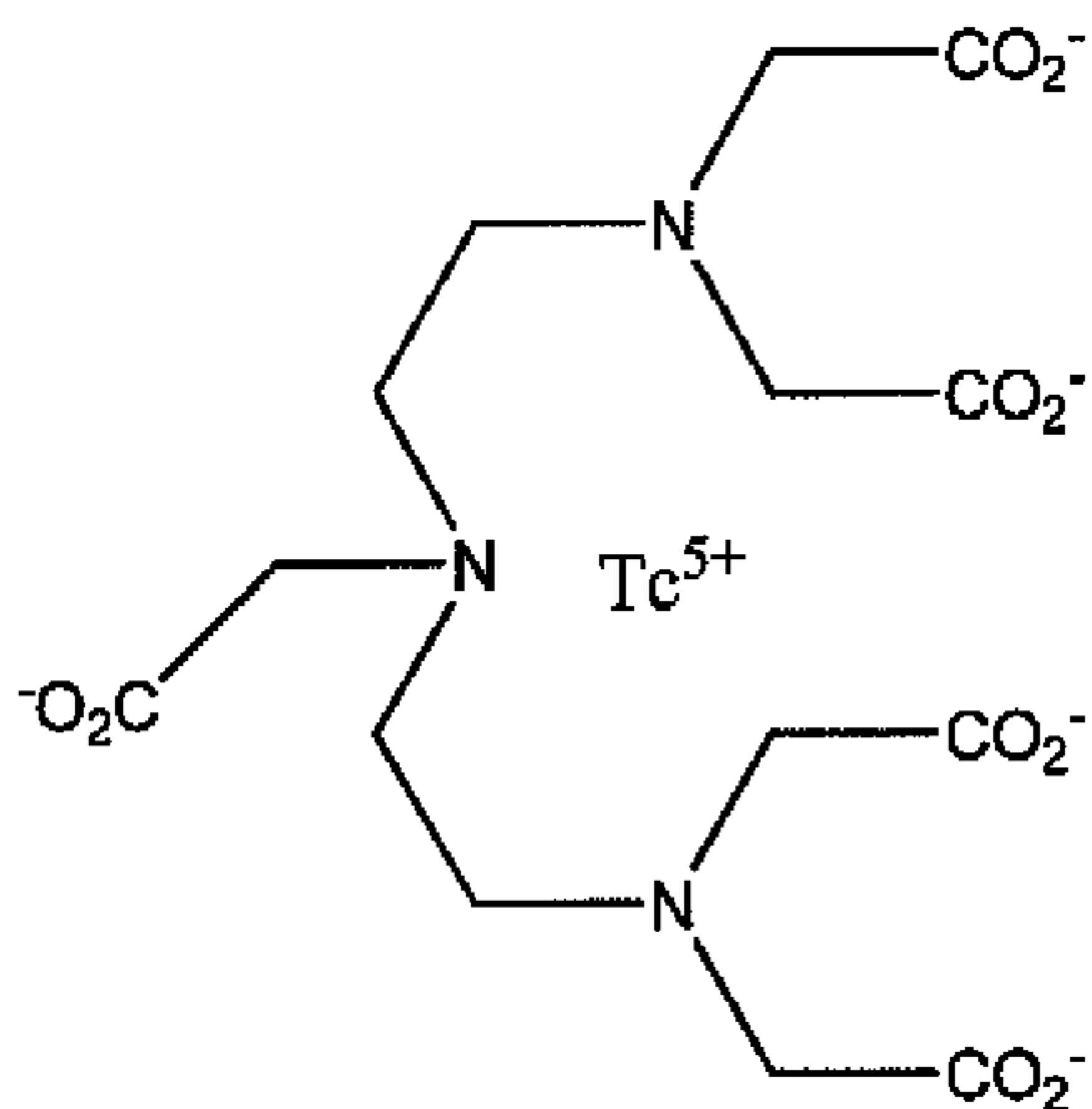
99m Tc-DTPA MW: 487
