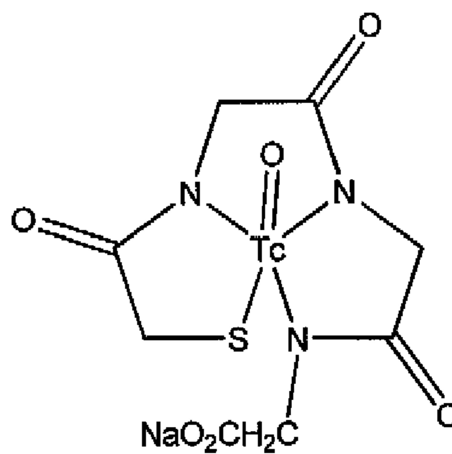
99m Tc-MAG3 MW: 364
