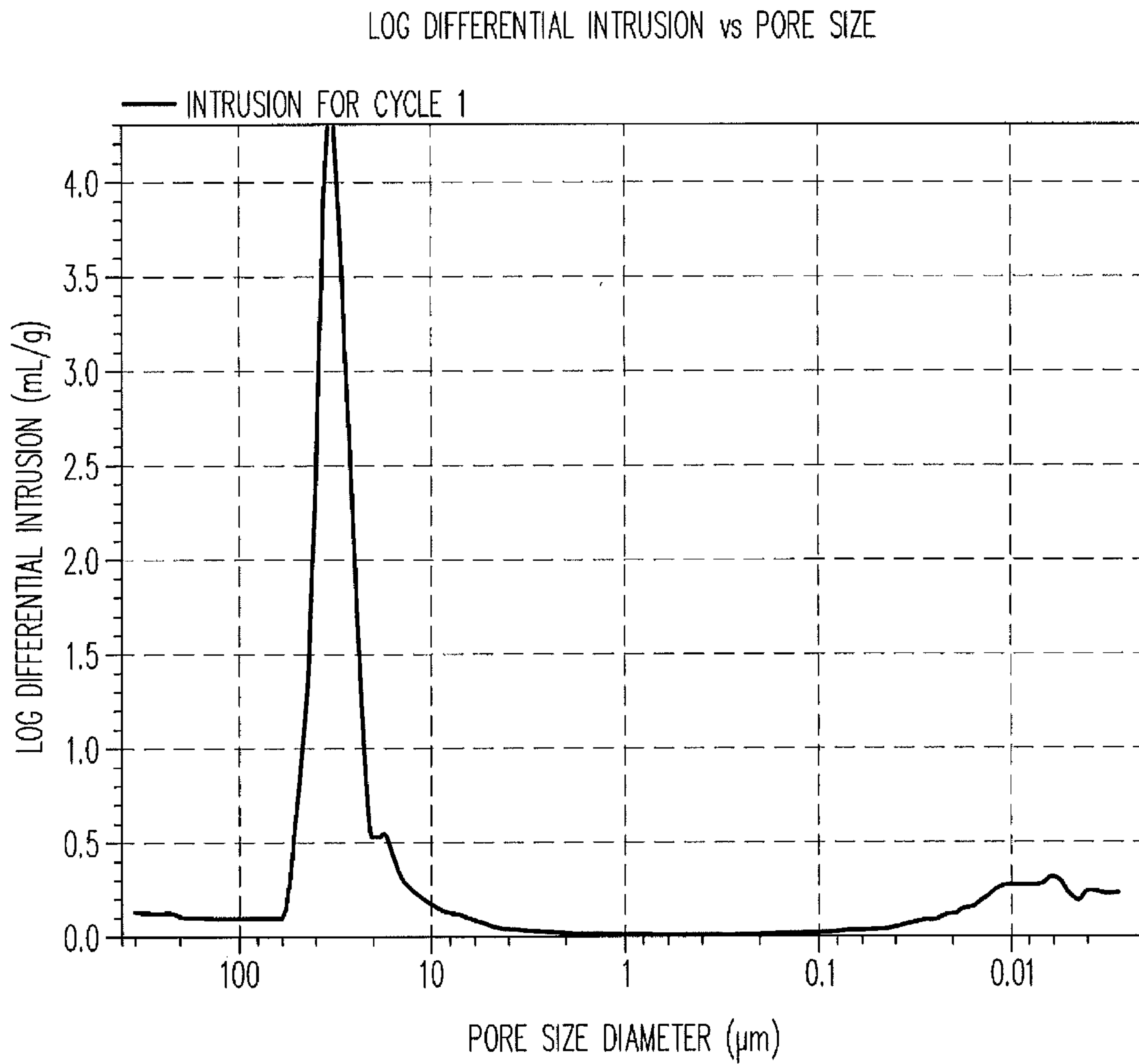
FIG. 21
