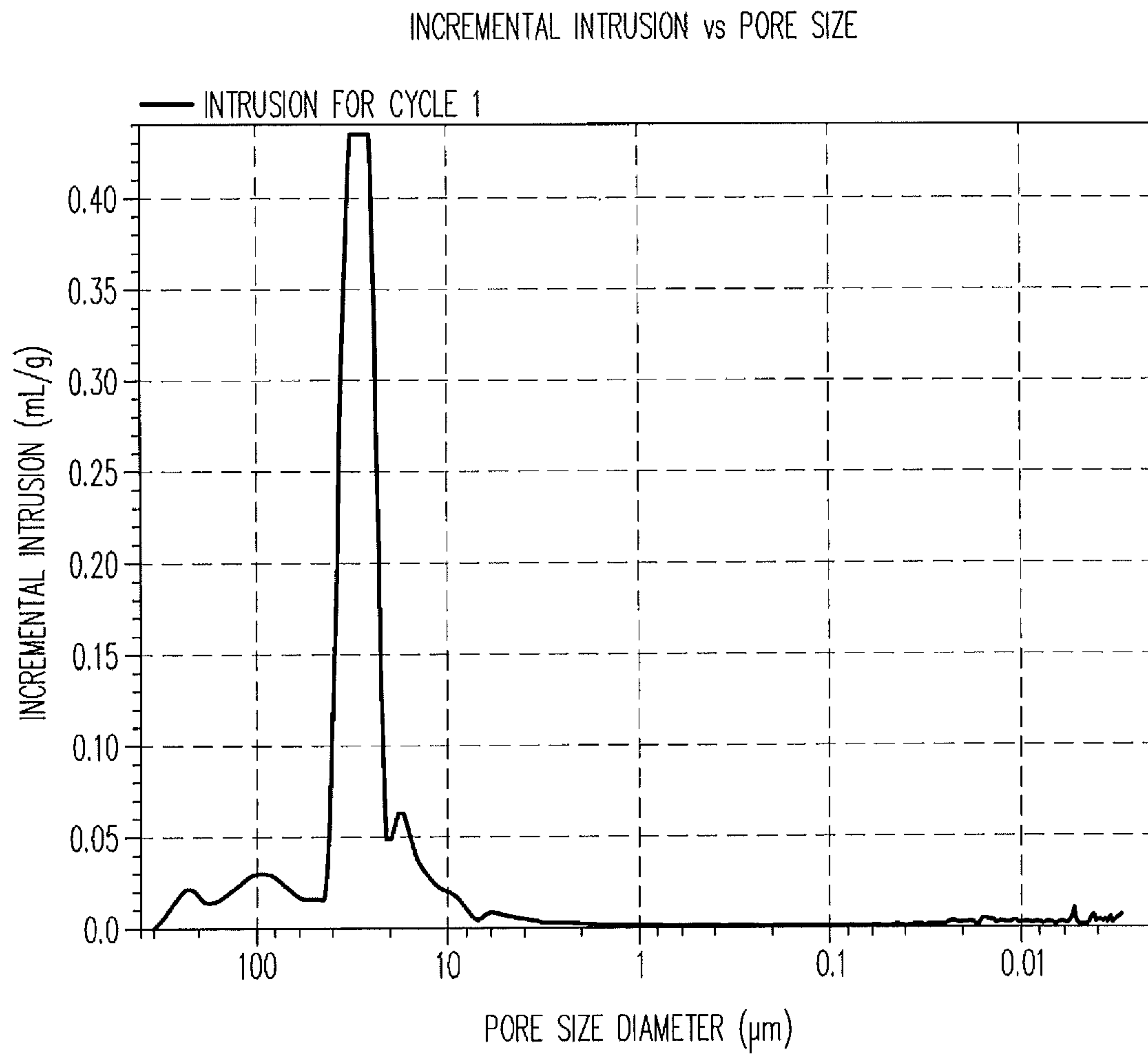
FIG. 18
