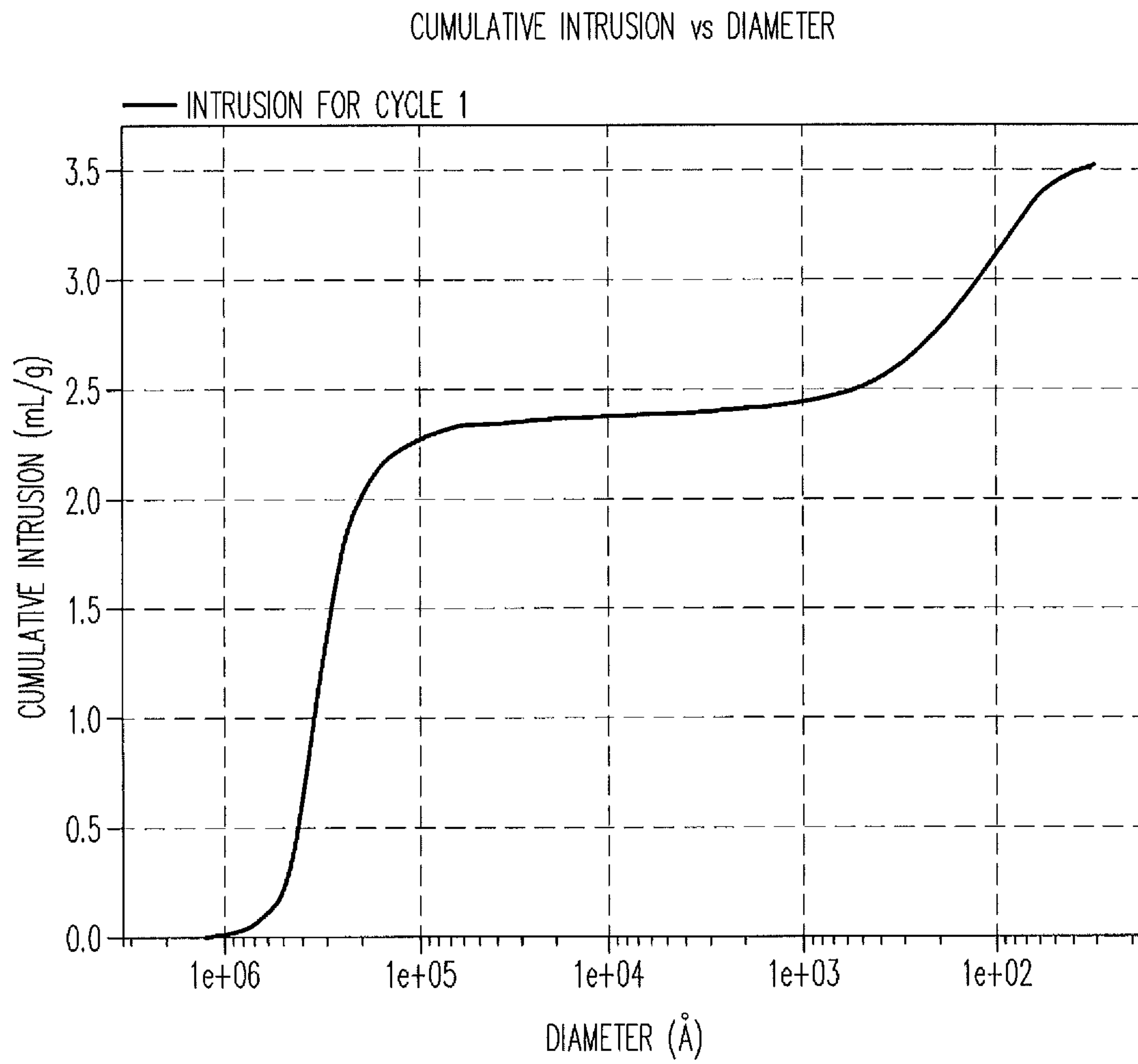
FIG. 4
