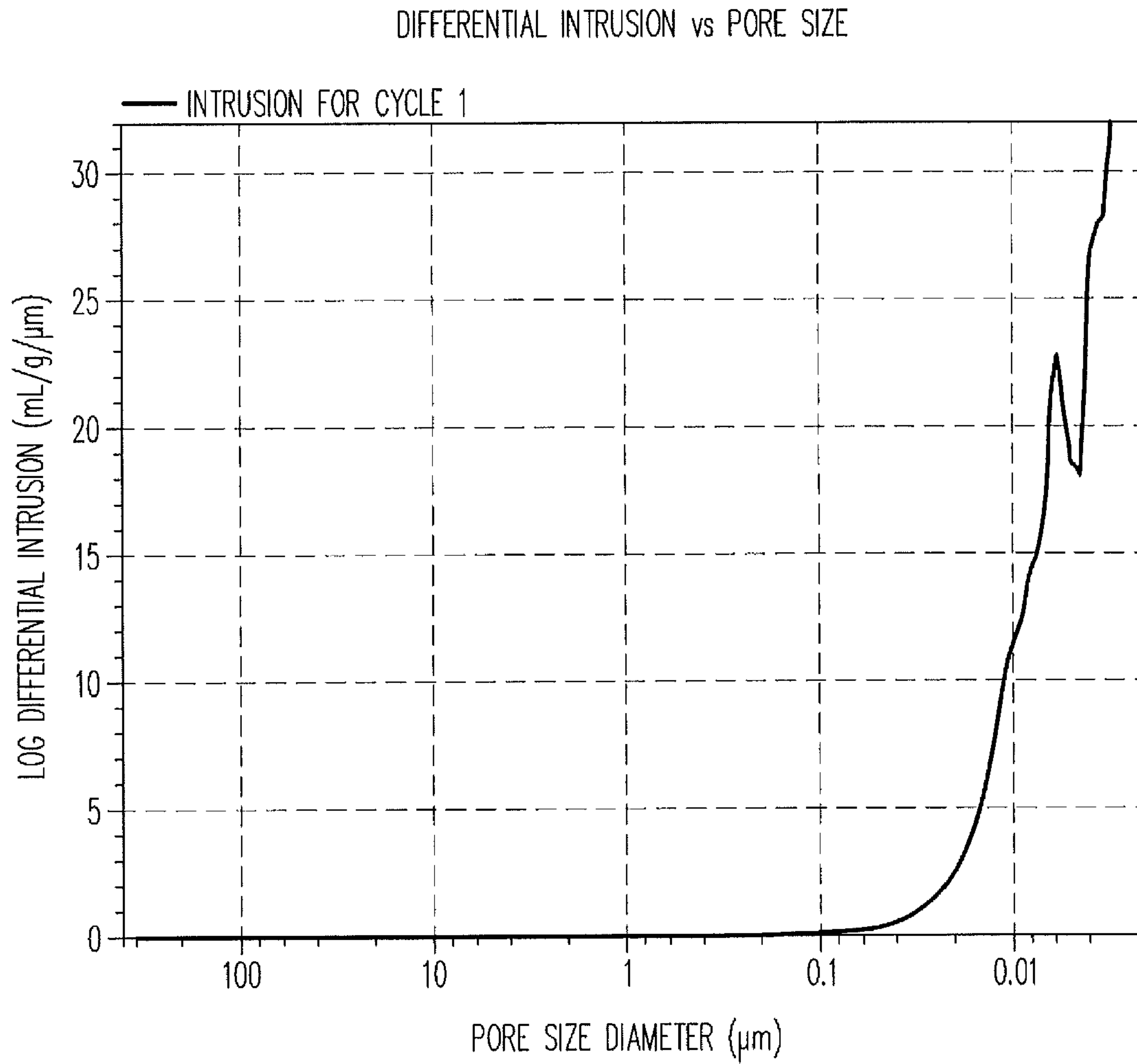
FIG. 20
