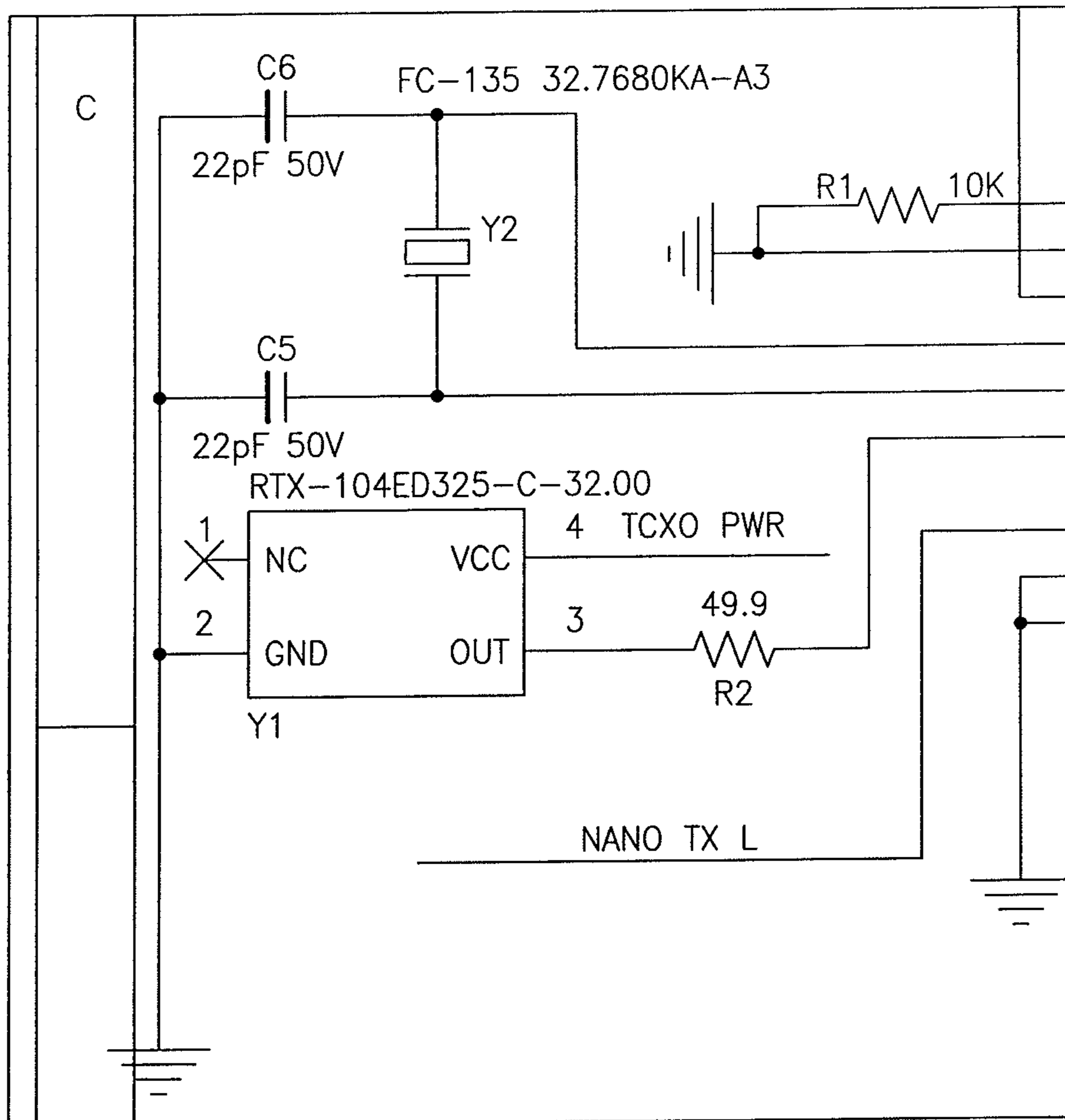
TCXO
