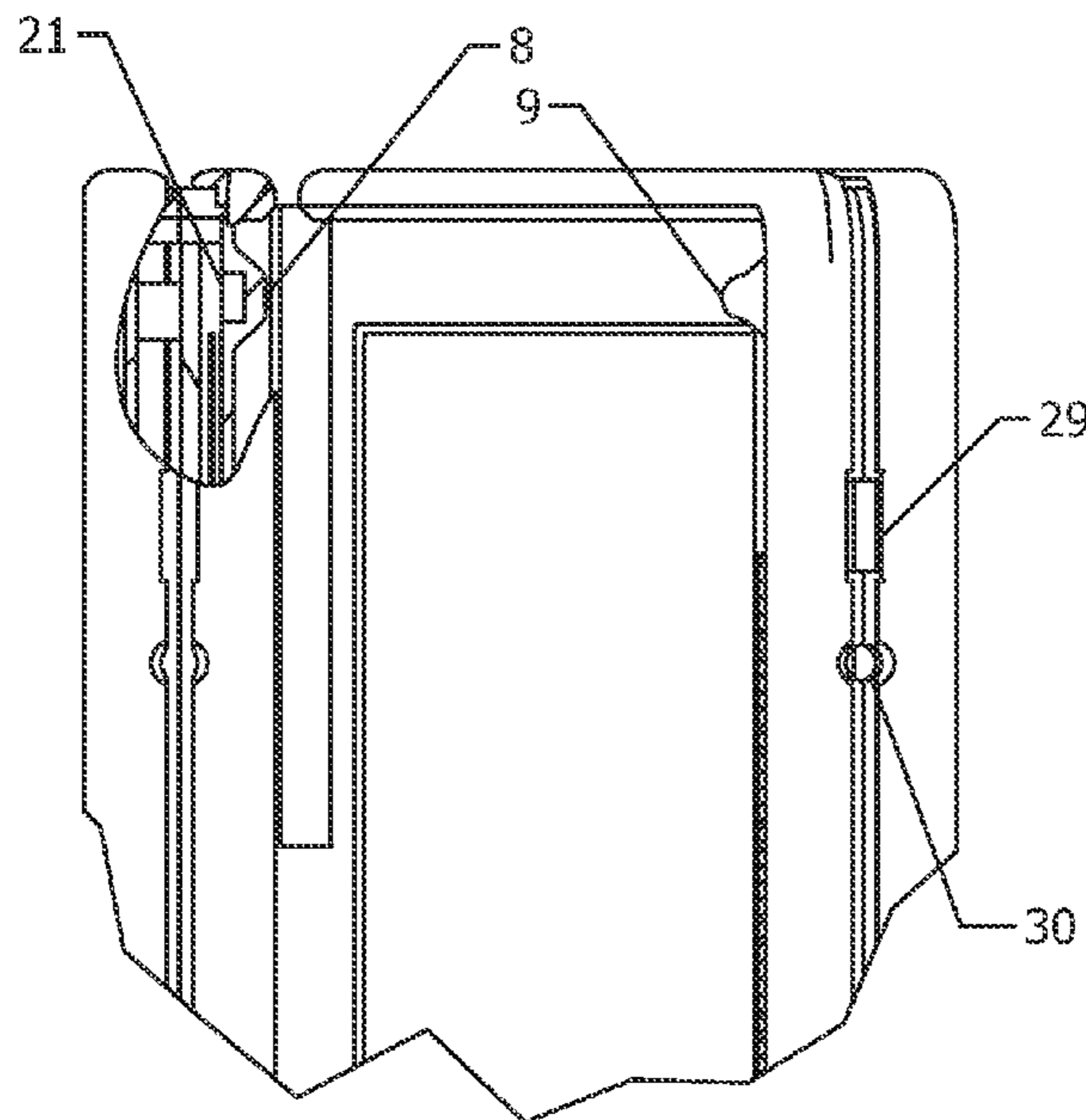
DETAIL 8A SCALE 1 : 1
