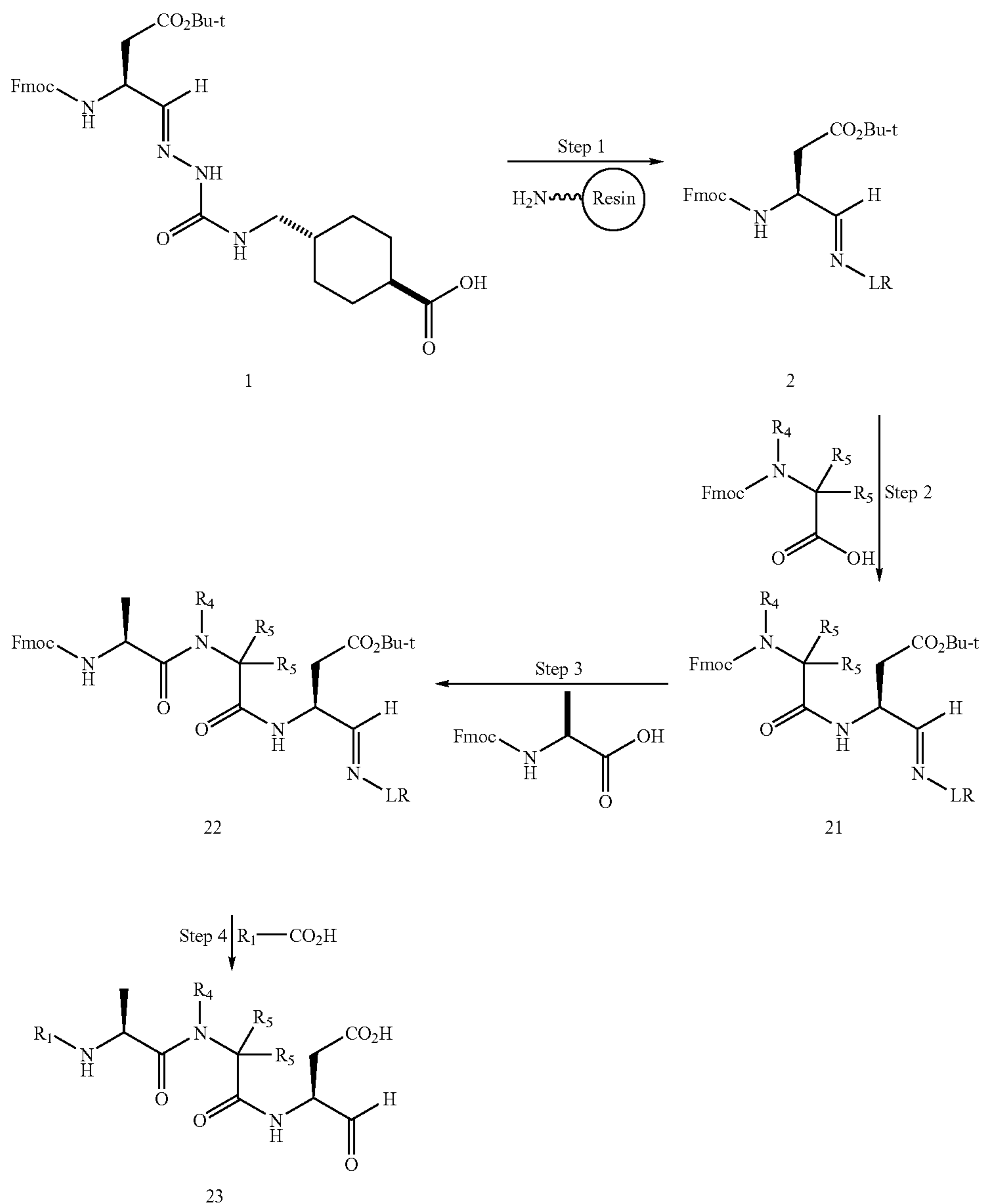
Scheme VI
