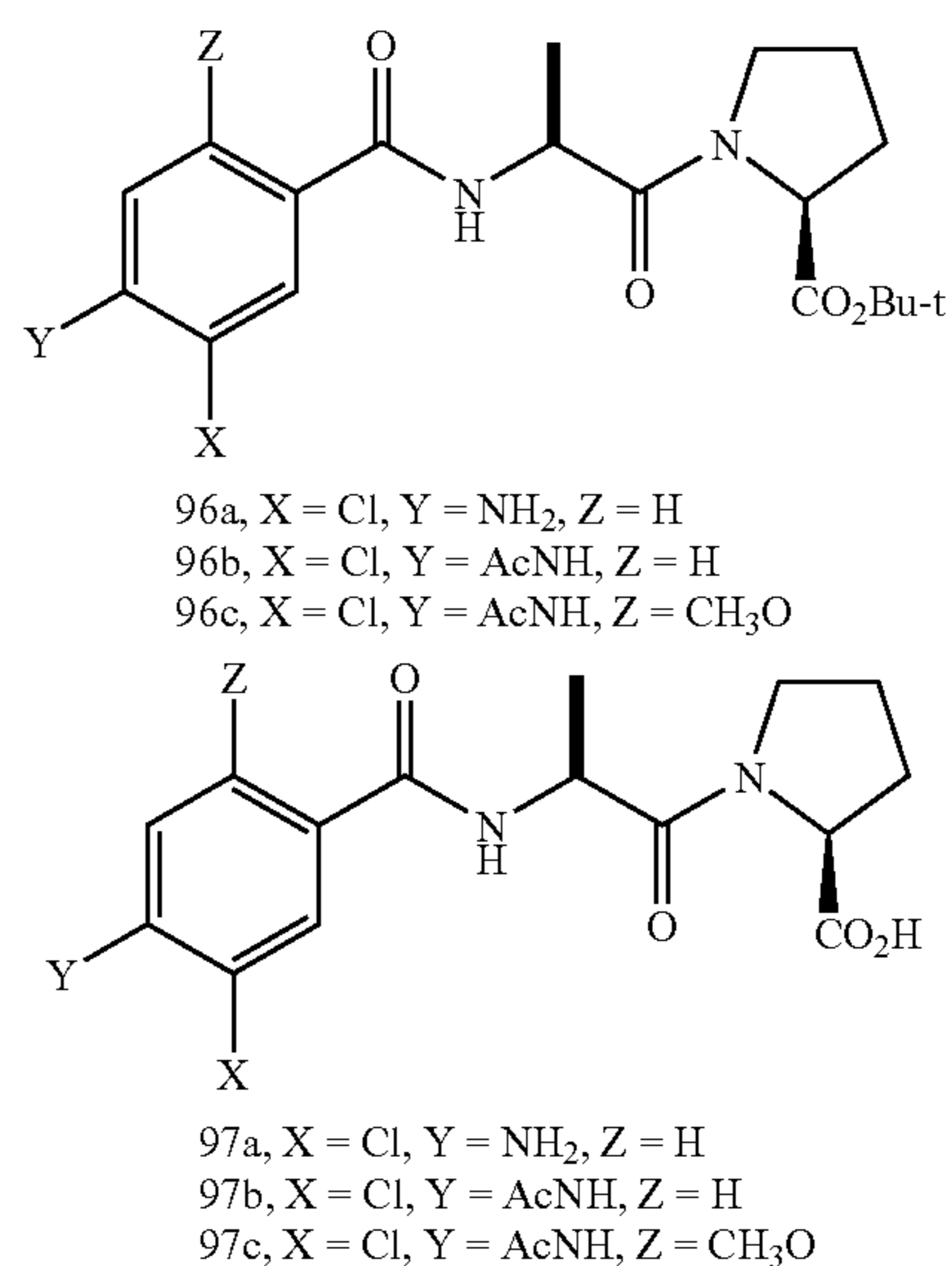
1-[2-(4-Amino-3-chloro-benzoylamino)-propionyl]-pyrrolidine-2-carboxylic acid tert-butyl ester (96a)
