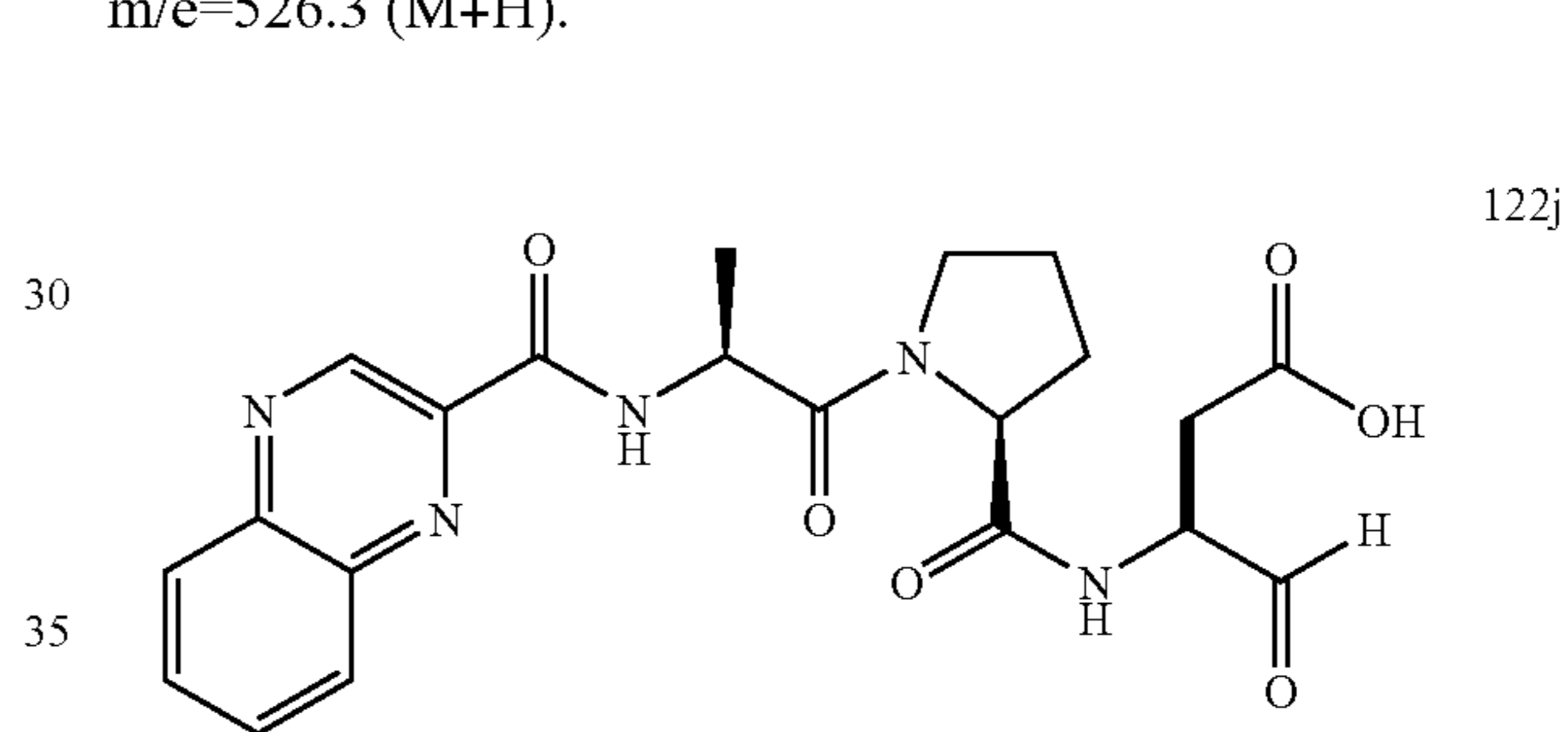
4-Oxo-3-[(1-{2-[(quinoxaline-2-carbonyl)-amino]-propionyl]-pyrrolidine-2-carbonyl}-amino]-butyrinic acid (122j)
