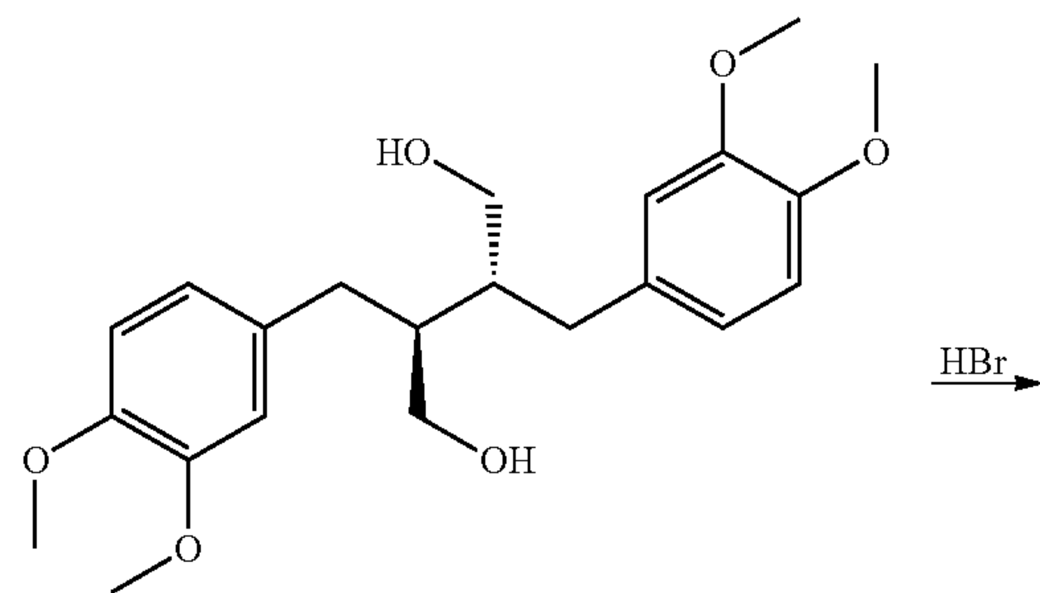
2,3-bis(hydroxymethyl)-1,4-bis-(3,4-dimethoxyphenyl)-butane
