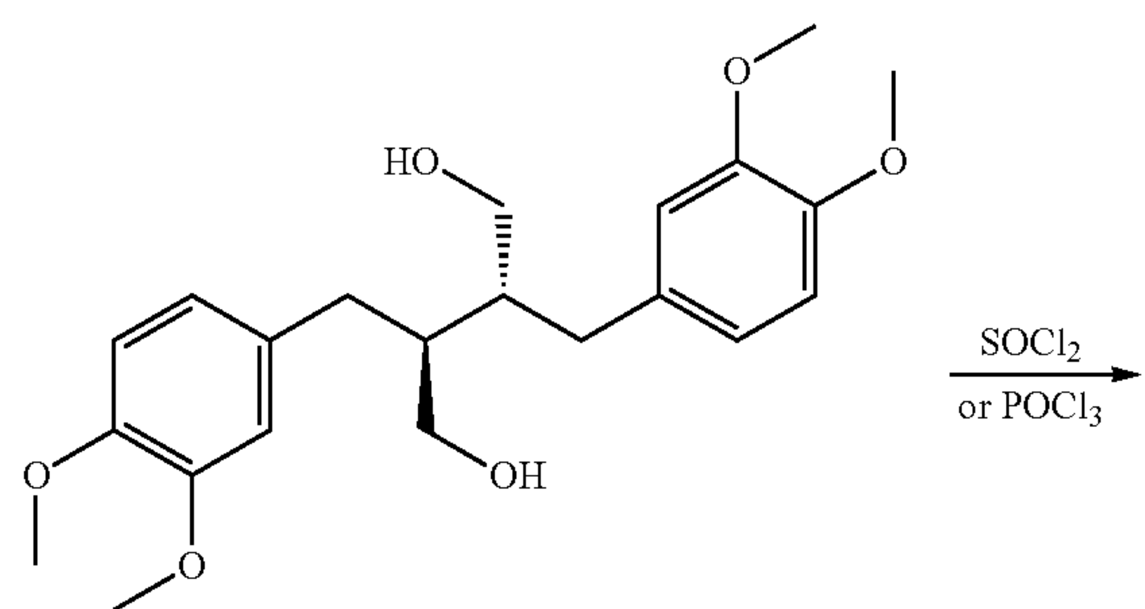
2,3-bis(hydroxymethyl)-1,4-bis-(3,4-dimethoxyphenyl)-butane
