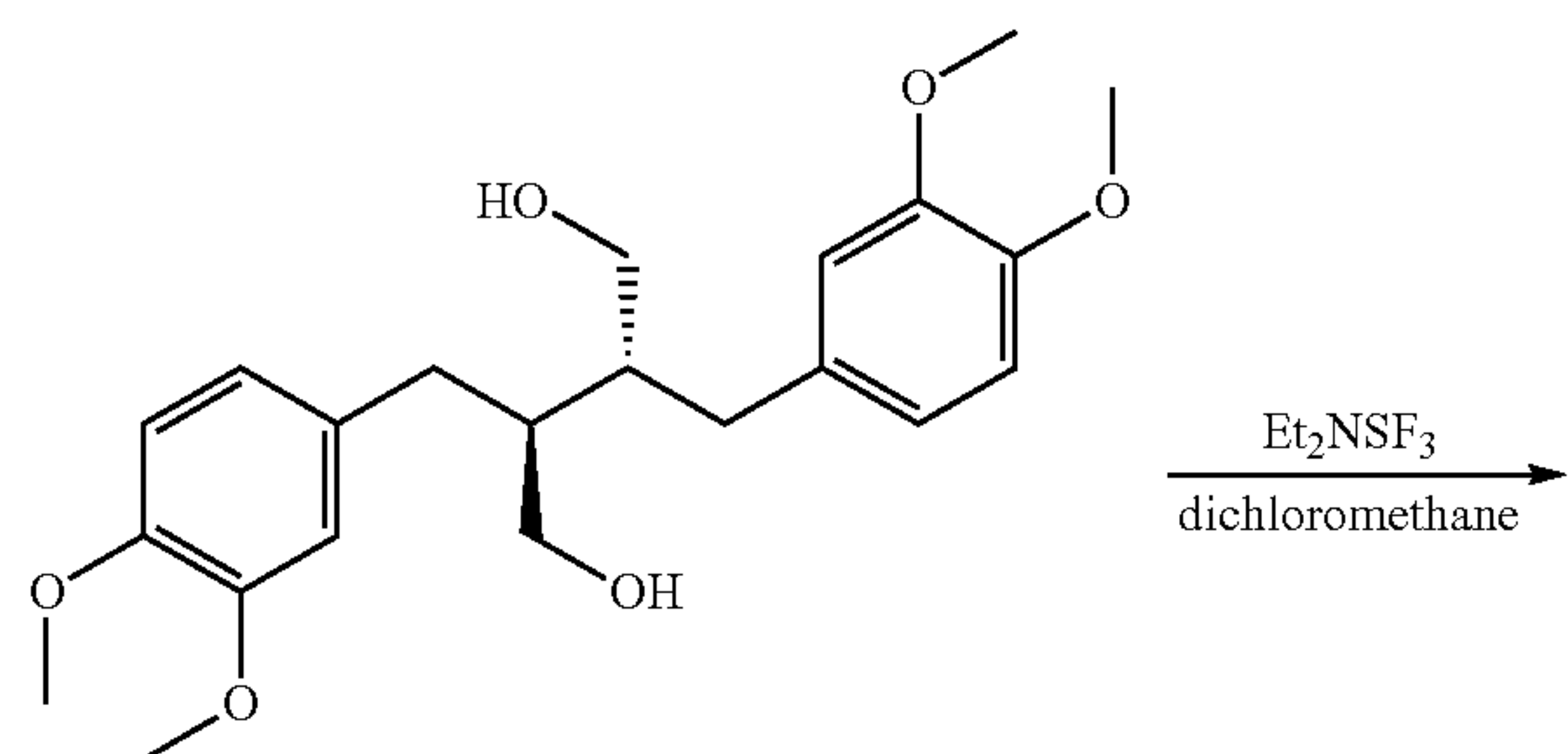
2,3-bis(hydroxymethyl)-1,4-bis-(3,4-dimethoxyphenyl)-butane
