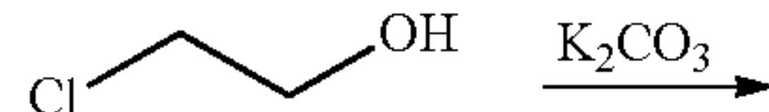
2-chloroethanol
