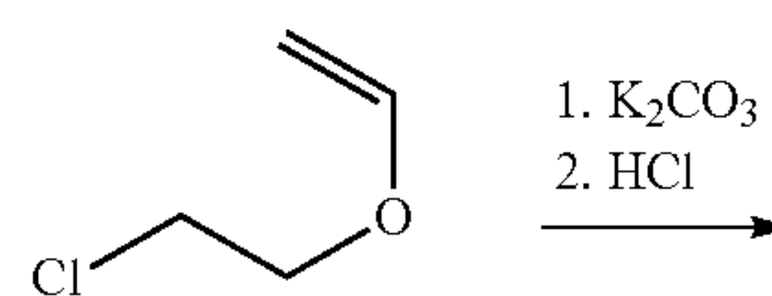
(2-chloroethoxy)ethene
