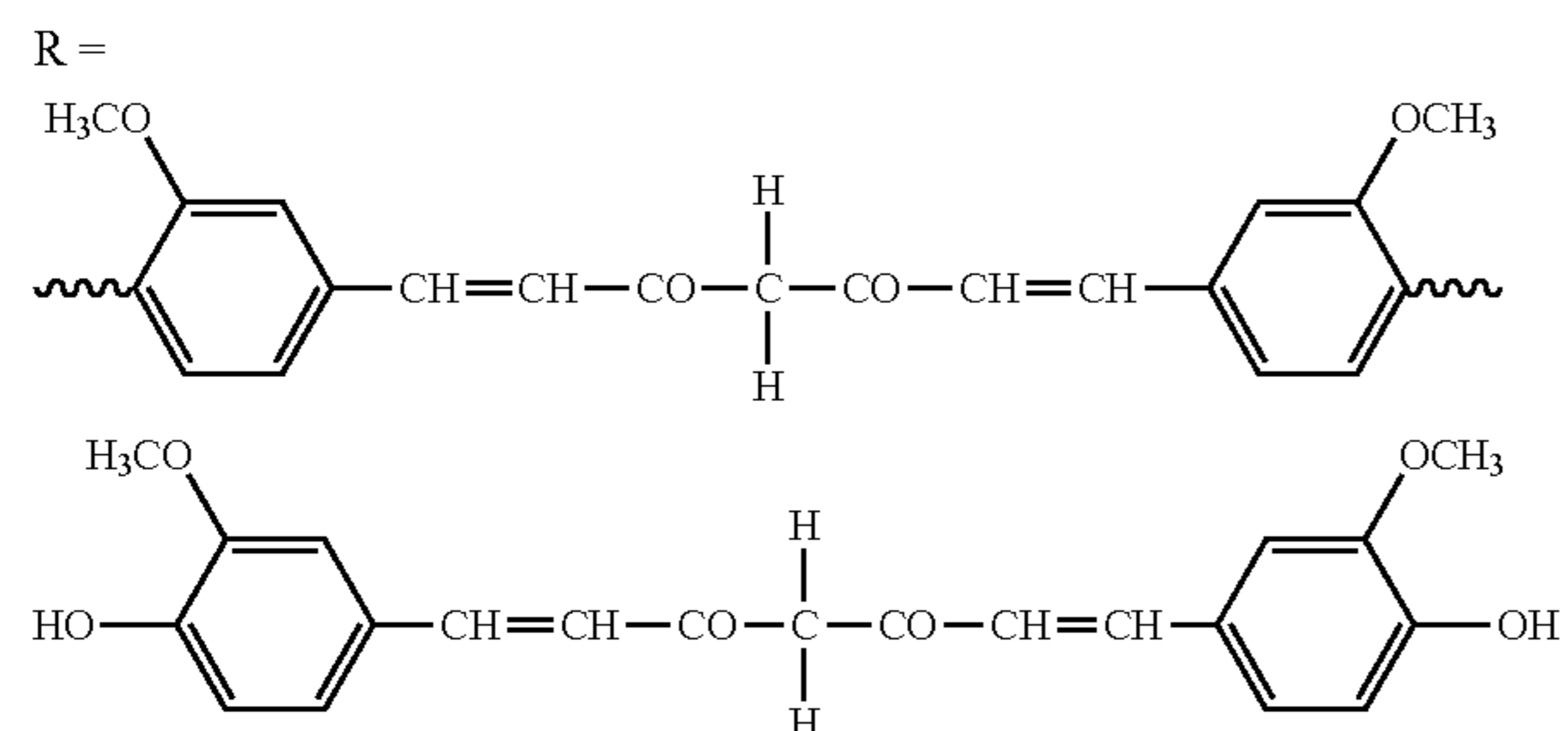
Curcumin
