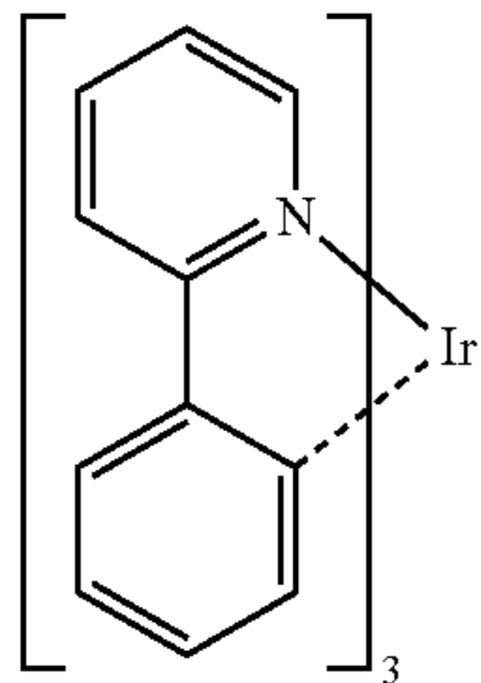
Ir(ppy) 3
