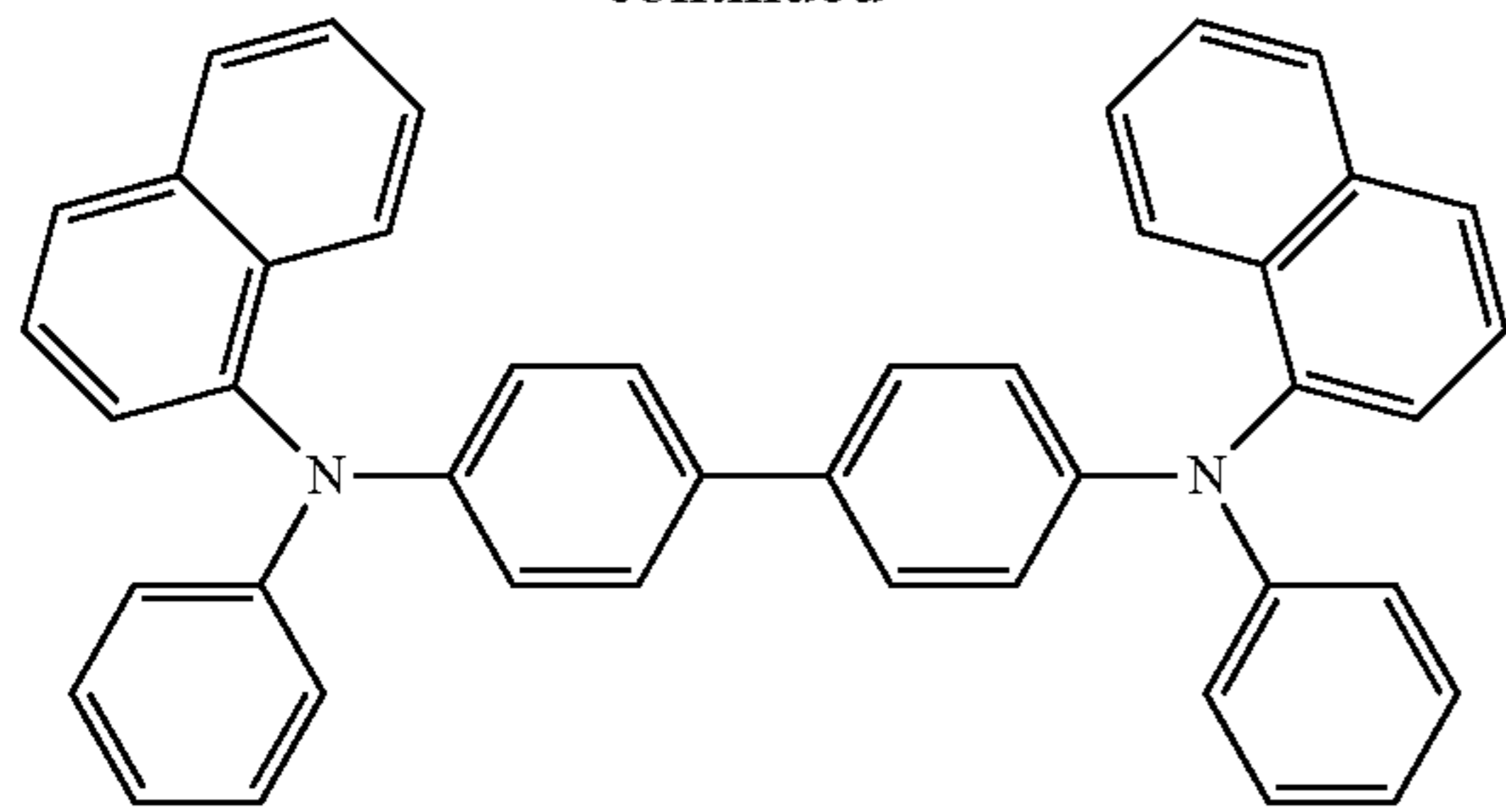
\alpha -NPD
