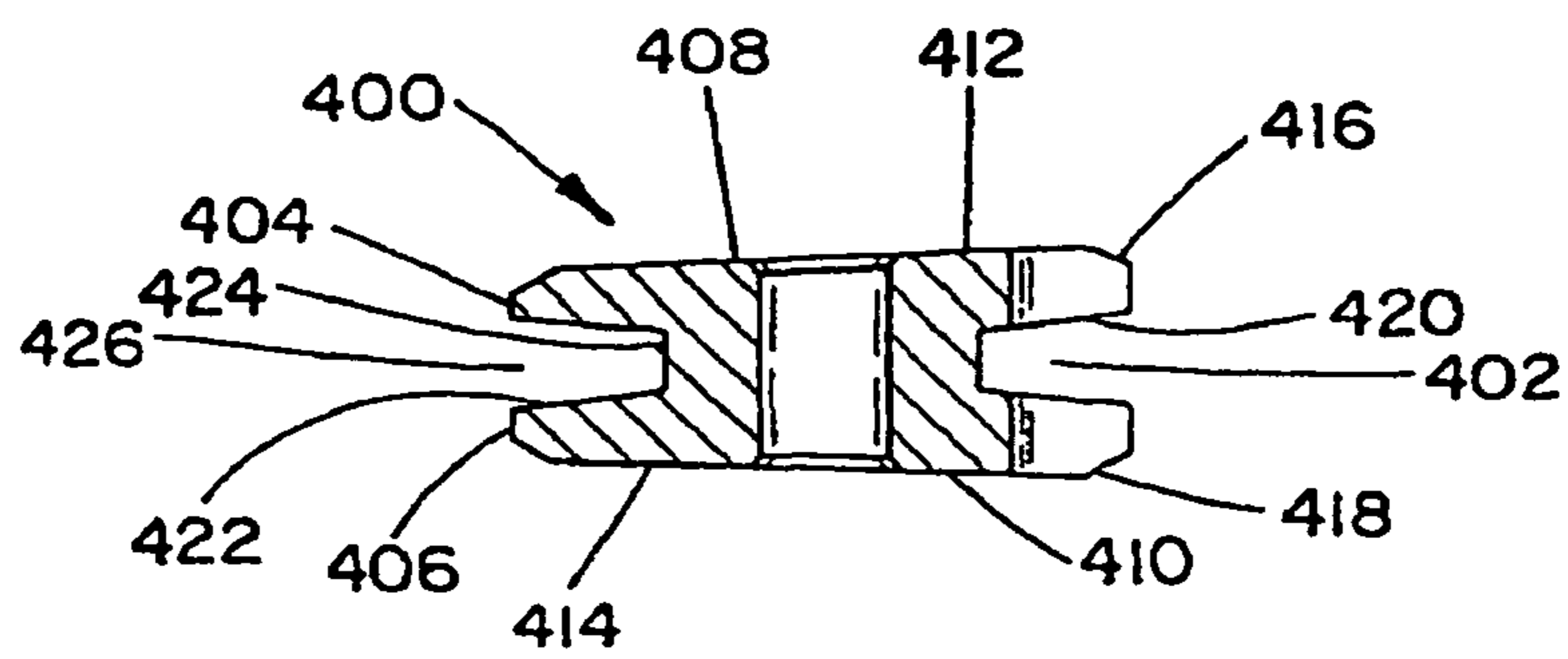
Section A-A
