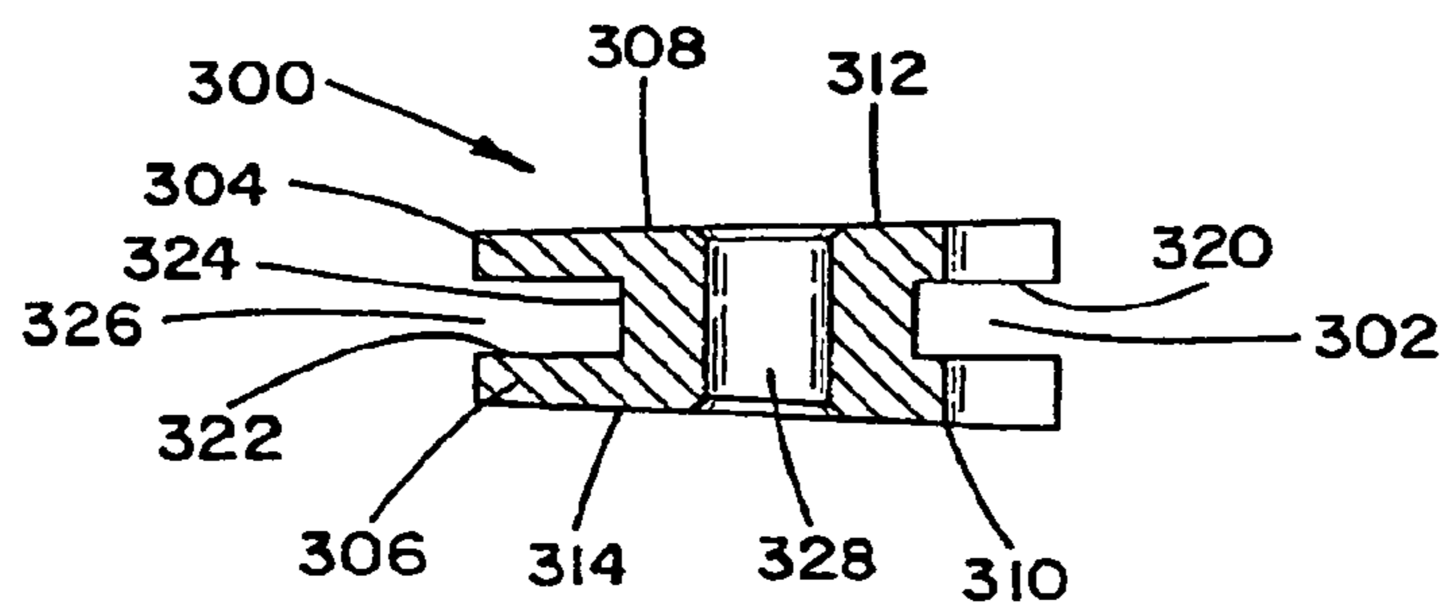
Section A-A
