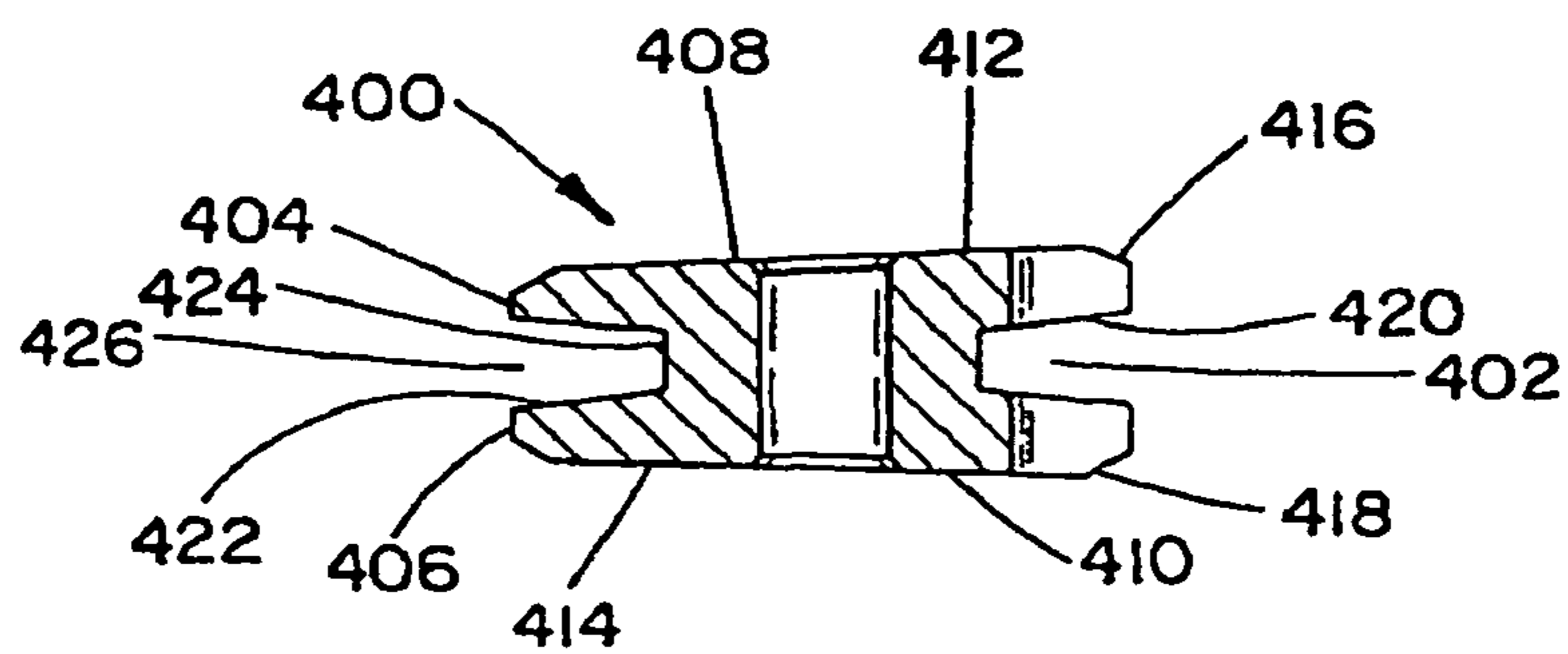
Section A-A
