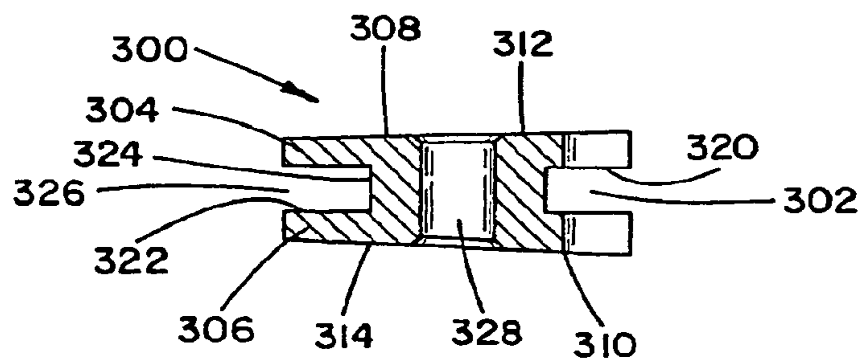
Section A-A
