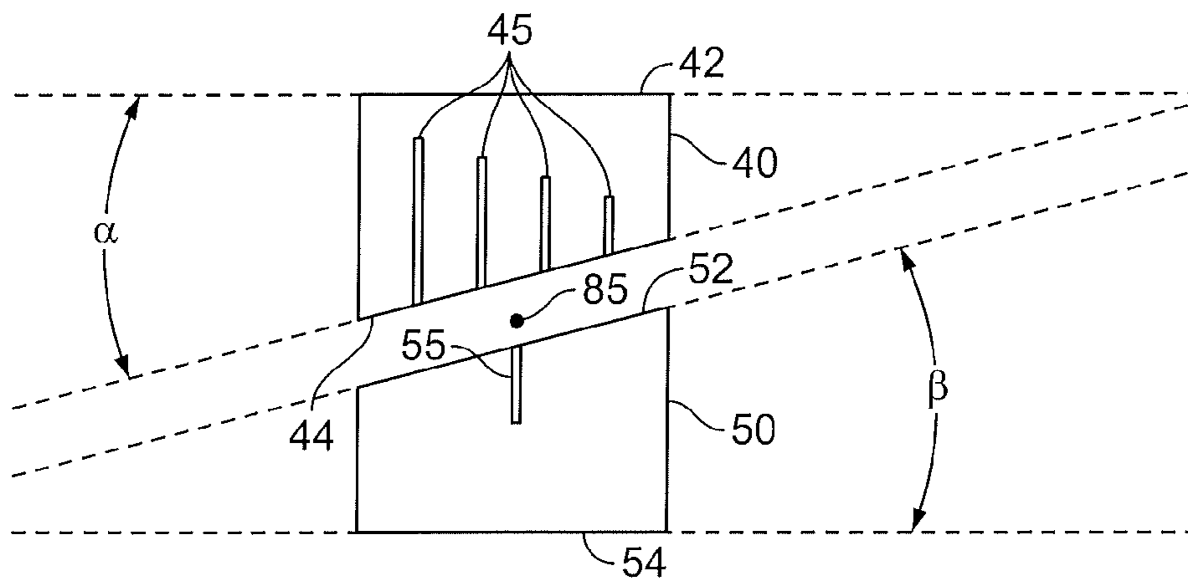
FIG. 7A
