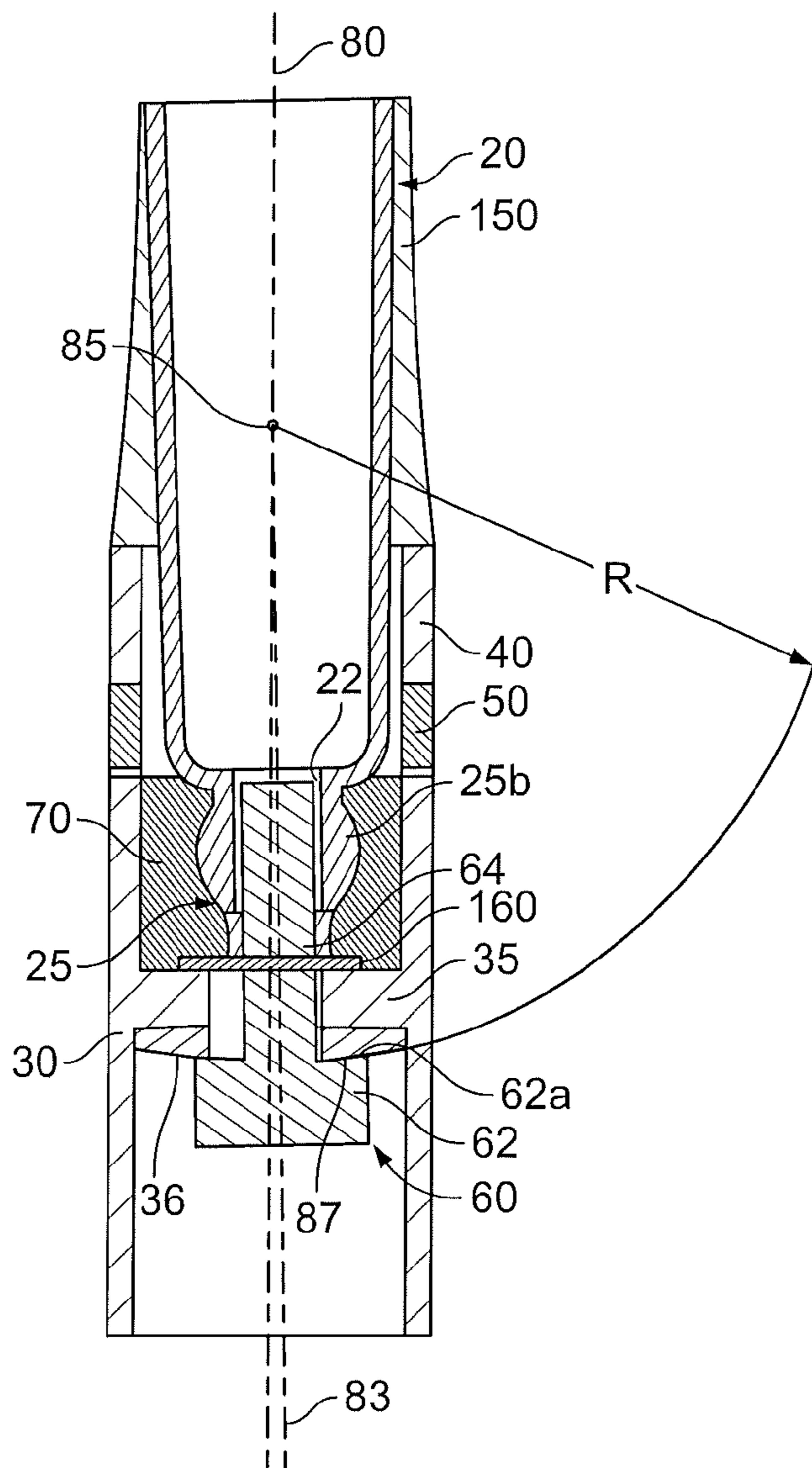
FIG. 8B
