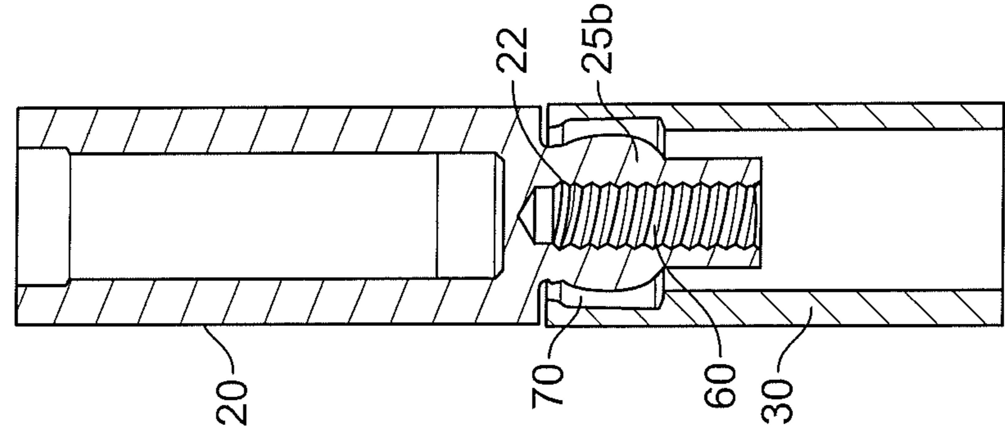
FIG. 4A
