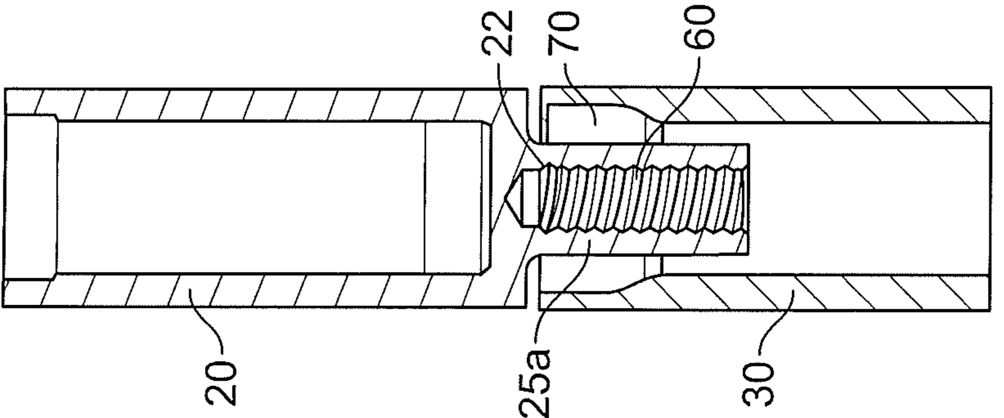
FIG. 4D
