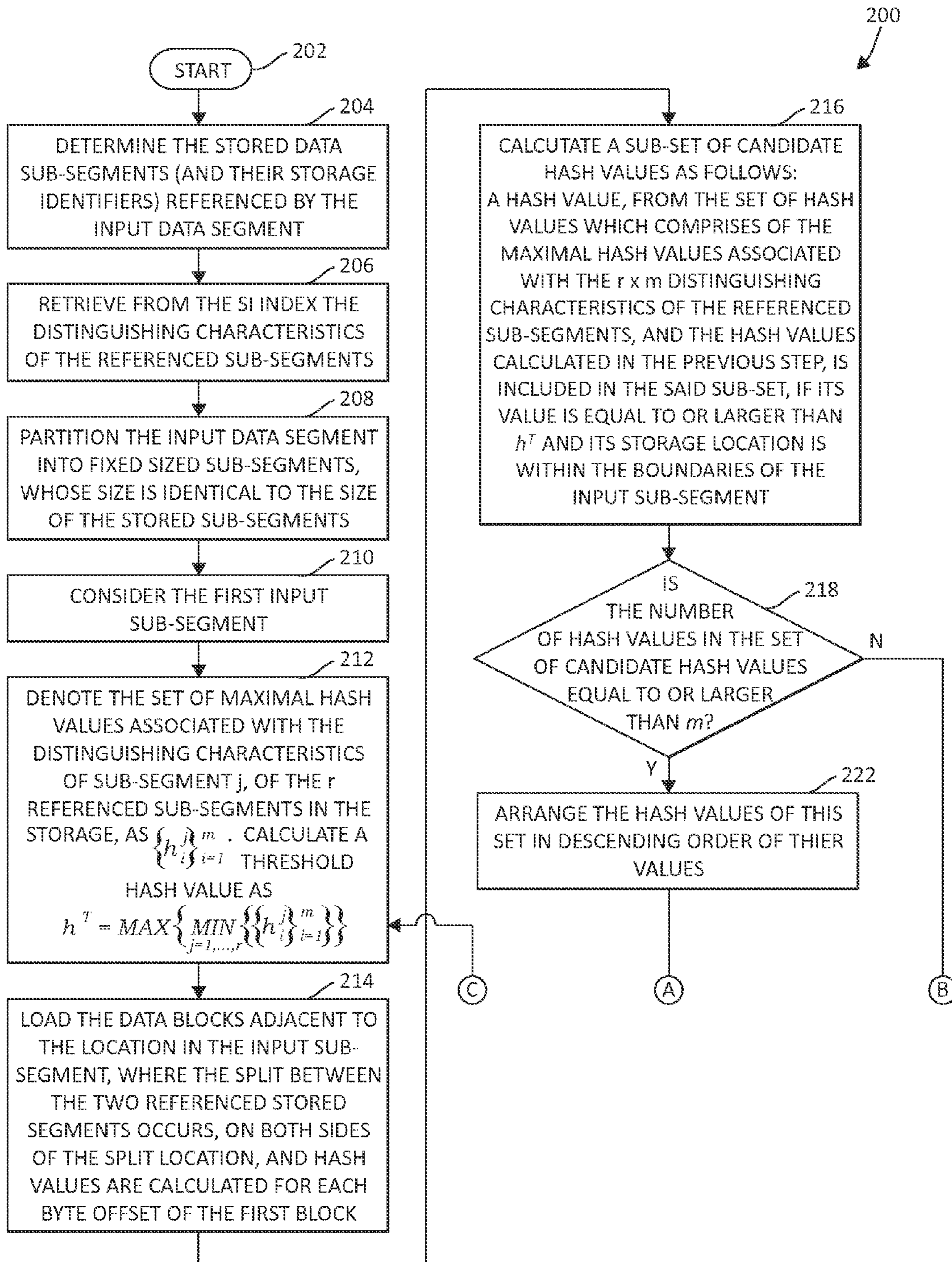
FIG. 10A
