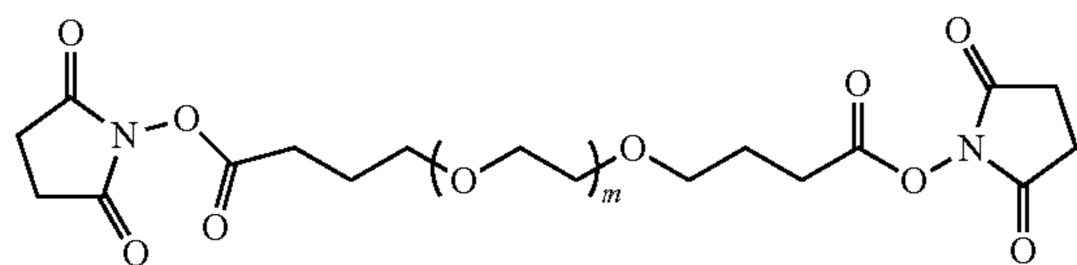
PEG-DiSBA (MW = 3400 Da)
