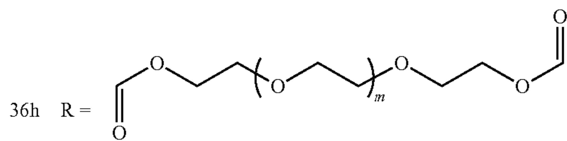
Poly(CDDCys-CB-PEG)
