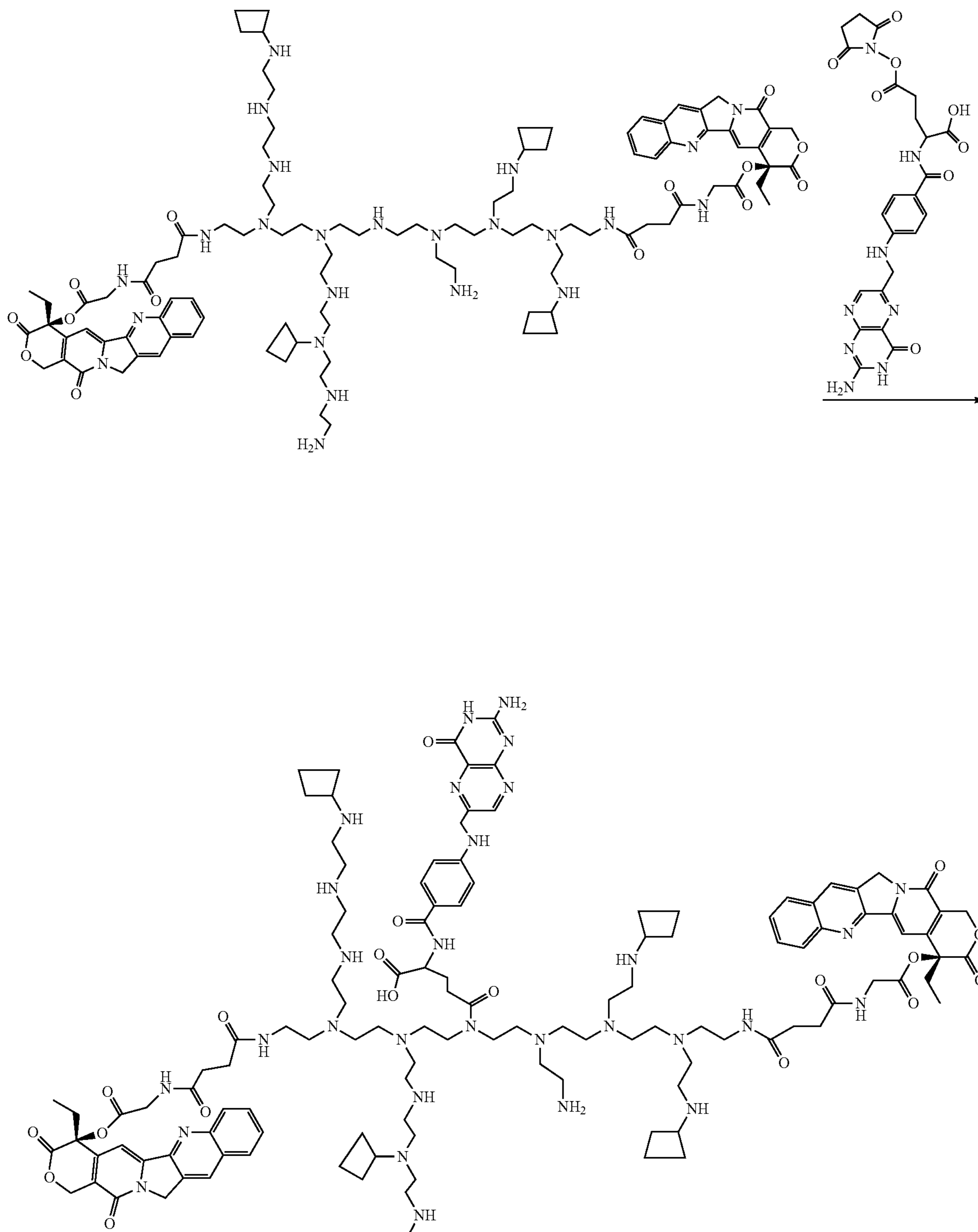
Scheme LI
