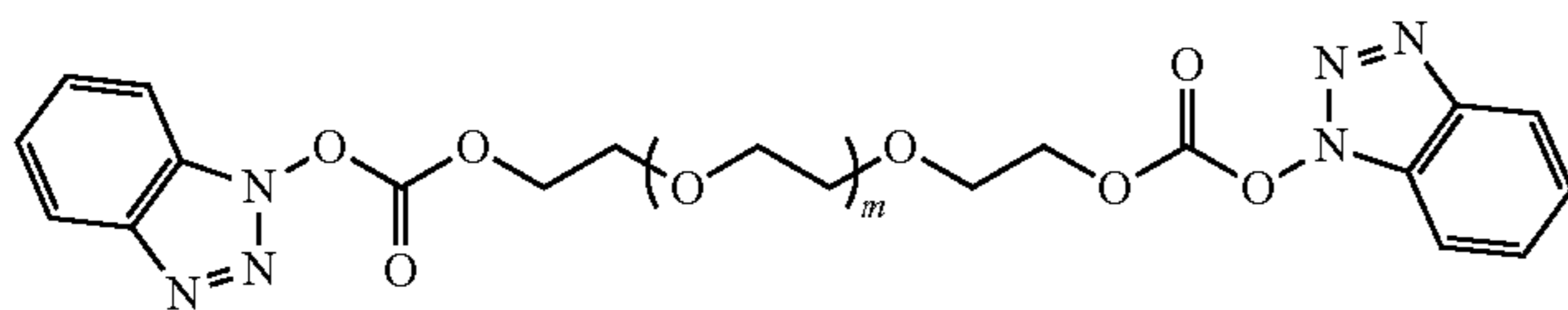
PEG-DiBTC (MW = 3400 Da)
