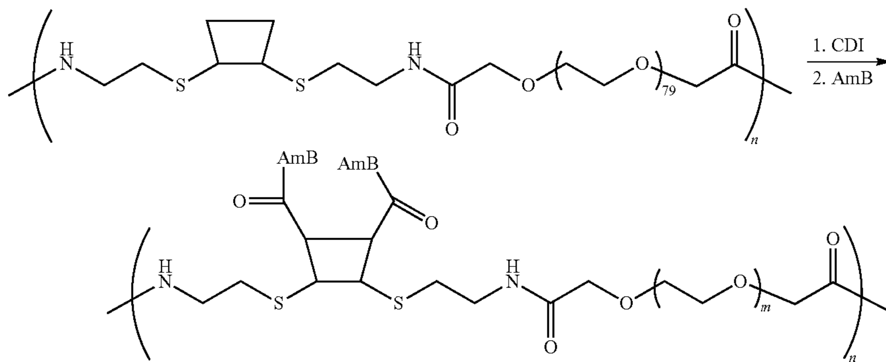
Scheme LII
