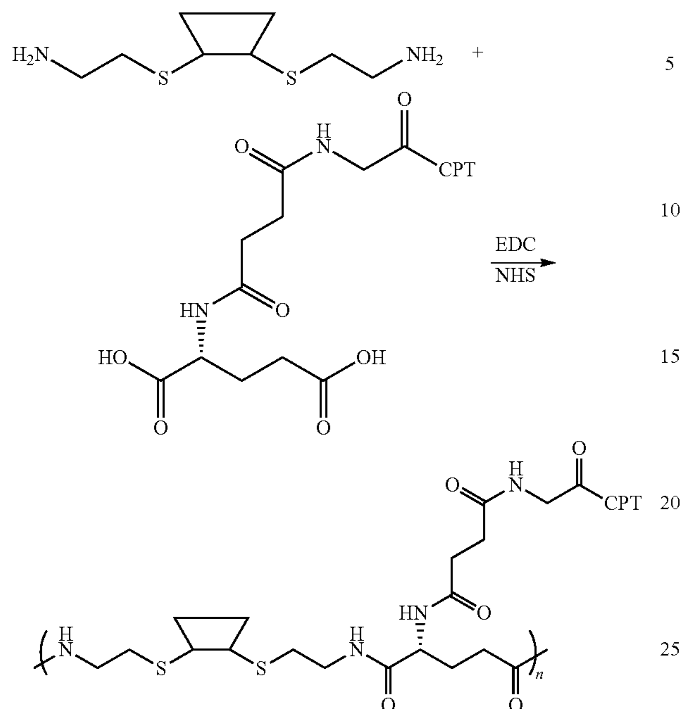
Scheme VI
