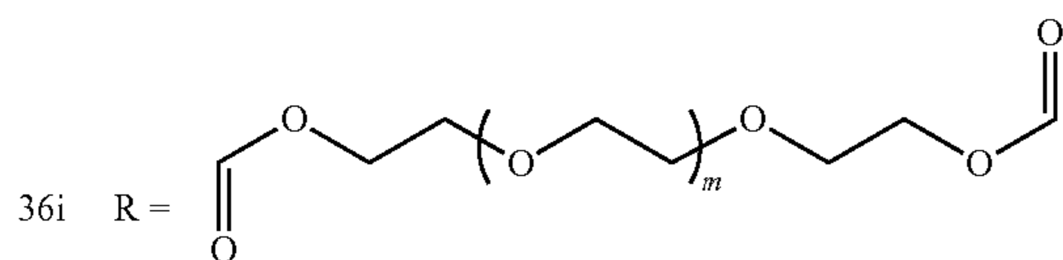
Poly(CDDCys-CB-PEG)
