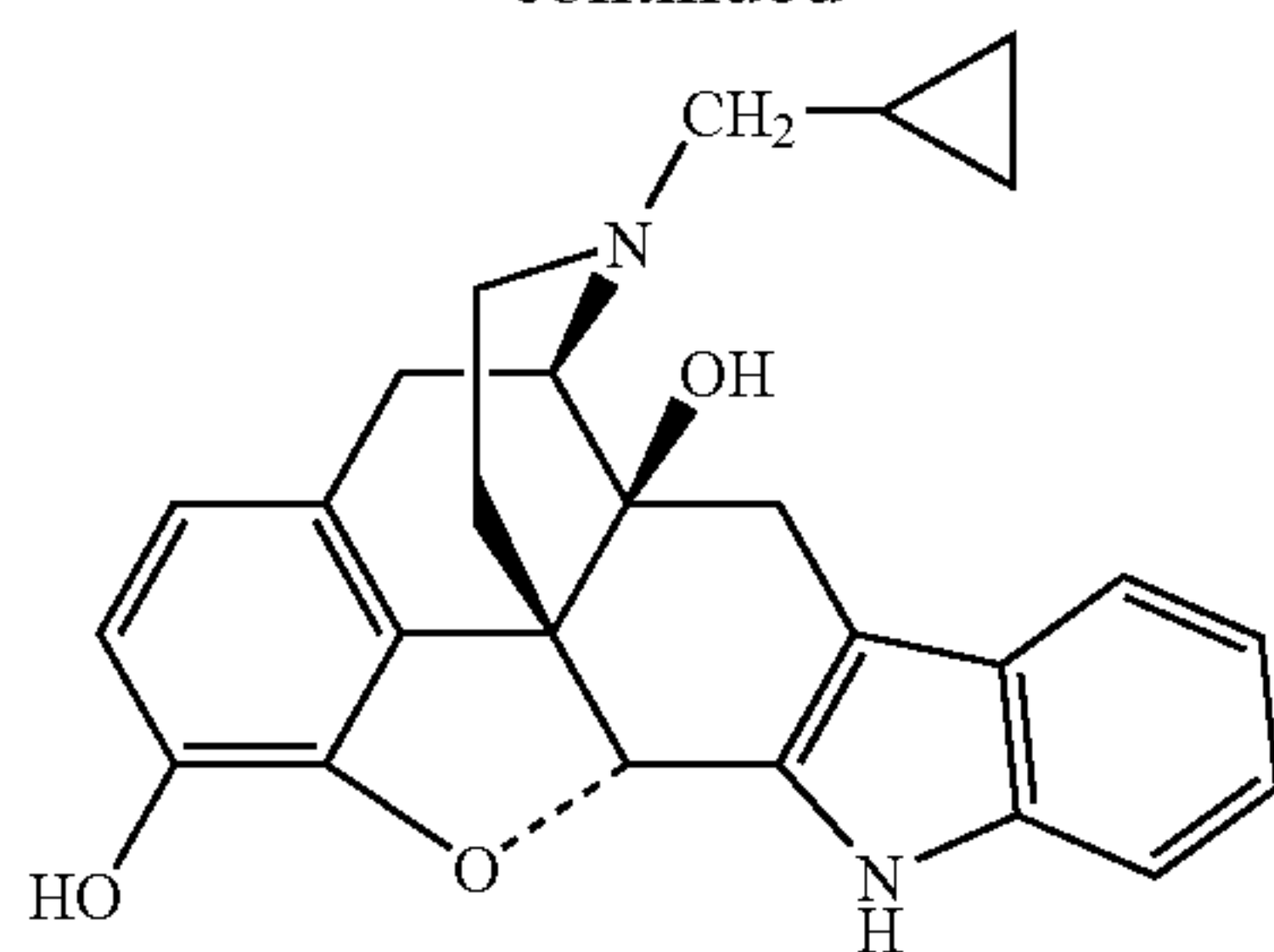
Naltrindole
