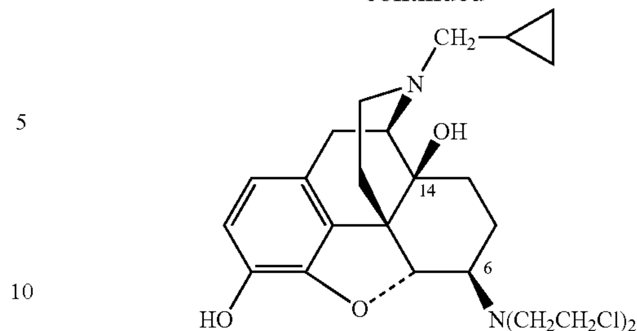
\beta -CNA
