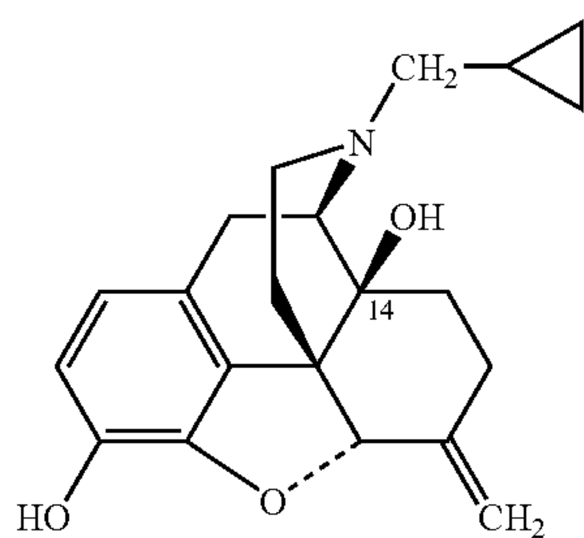
Nalmefene
