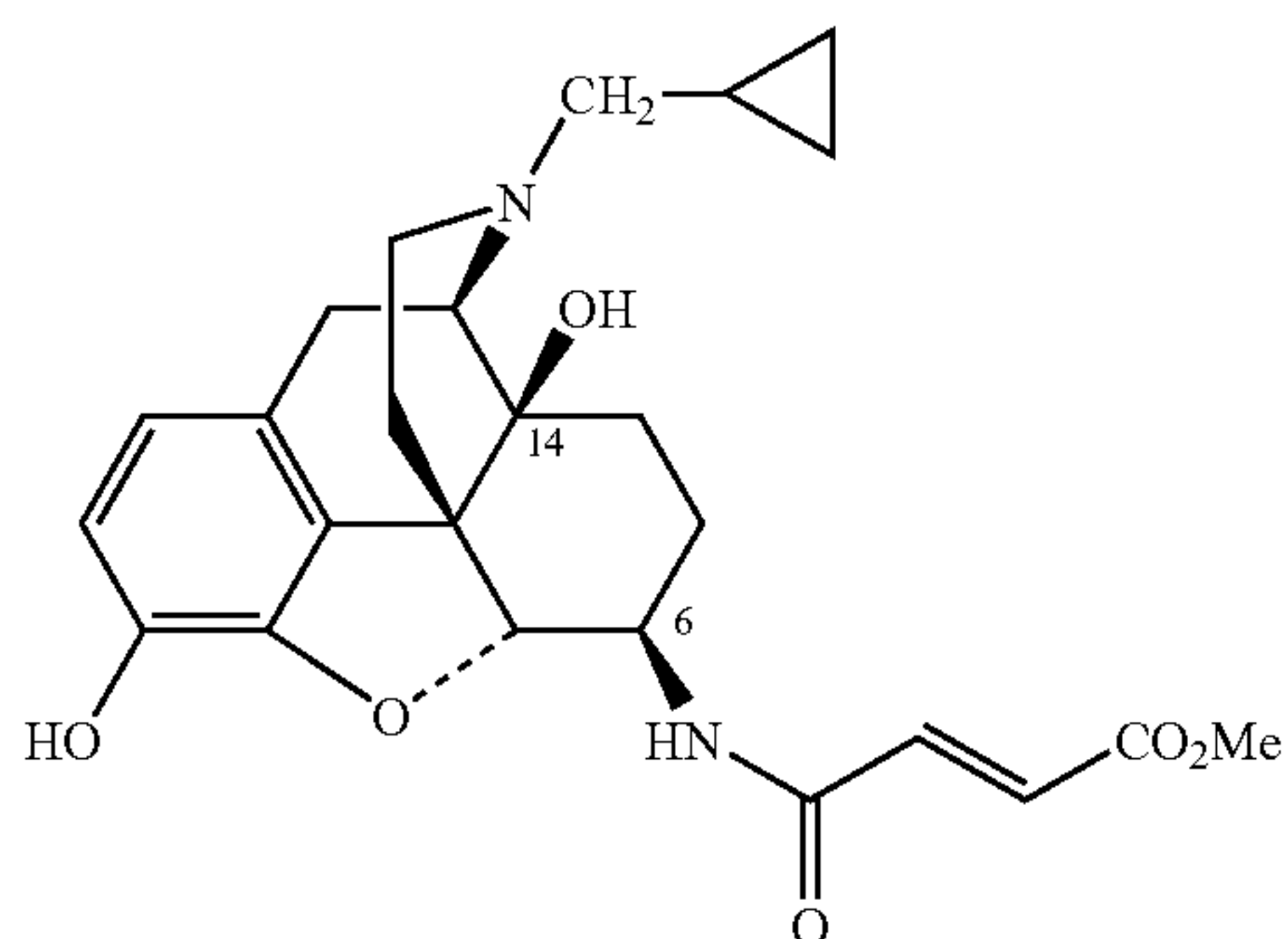
\beta -FNA
