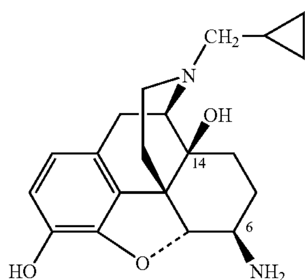
\beta -Naltrexamine
