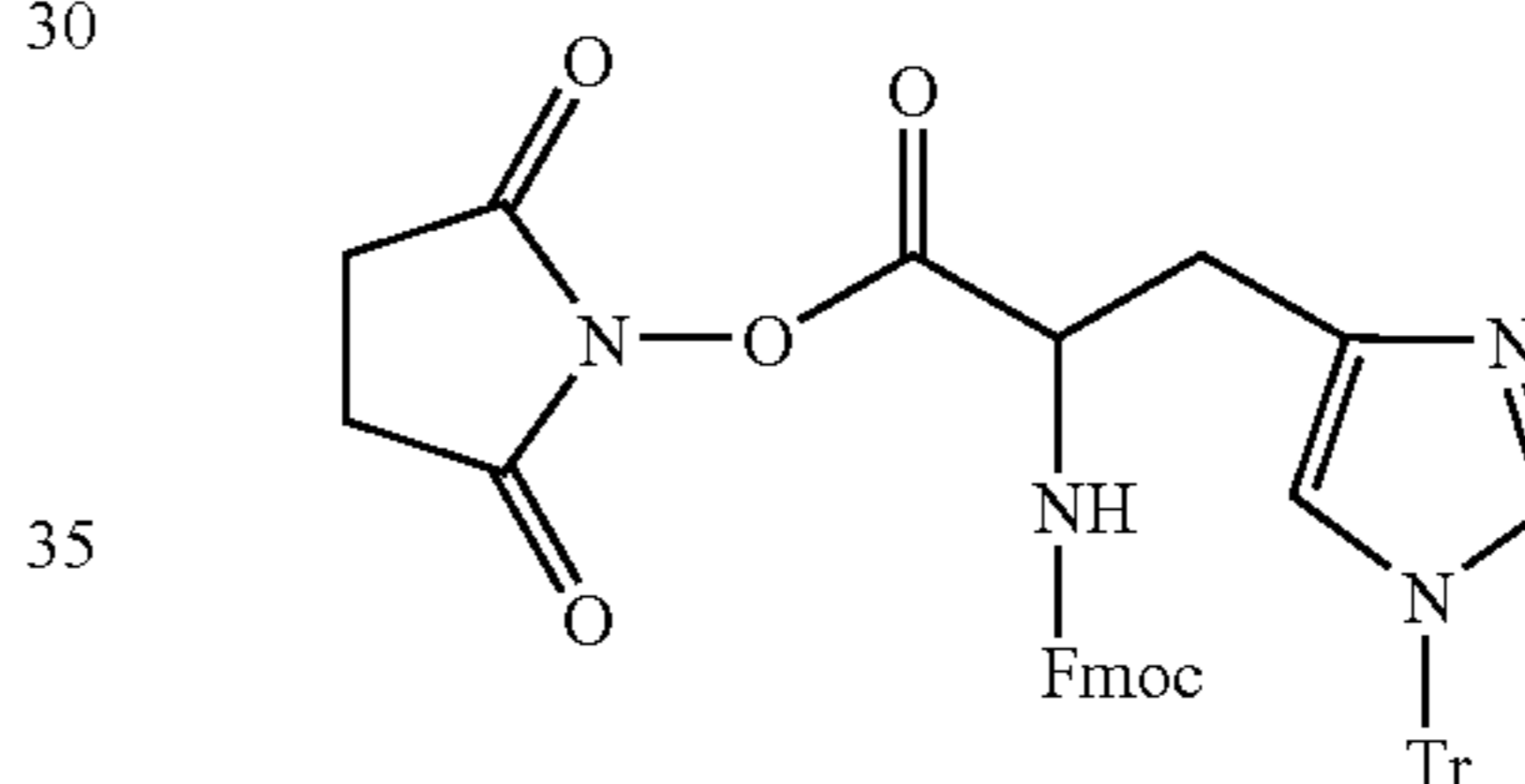
NHS-Histidine
