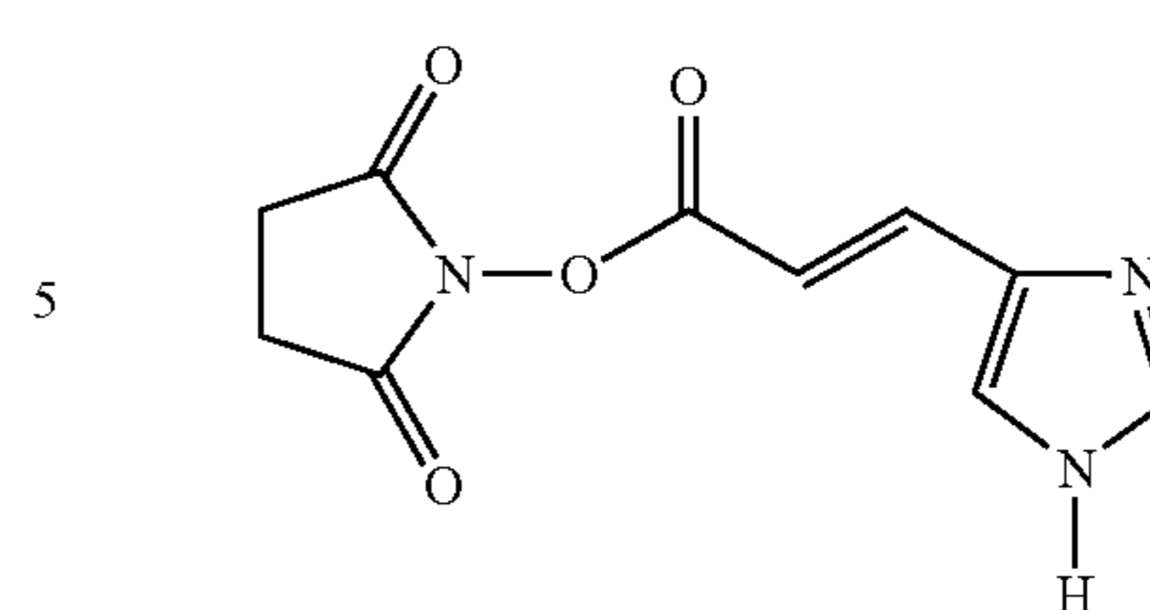
NHS-Urocanic
