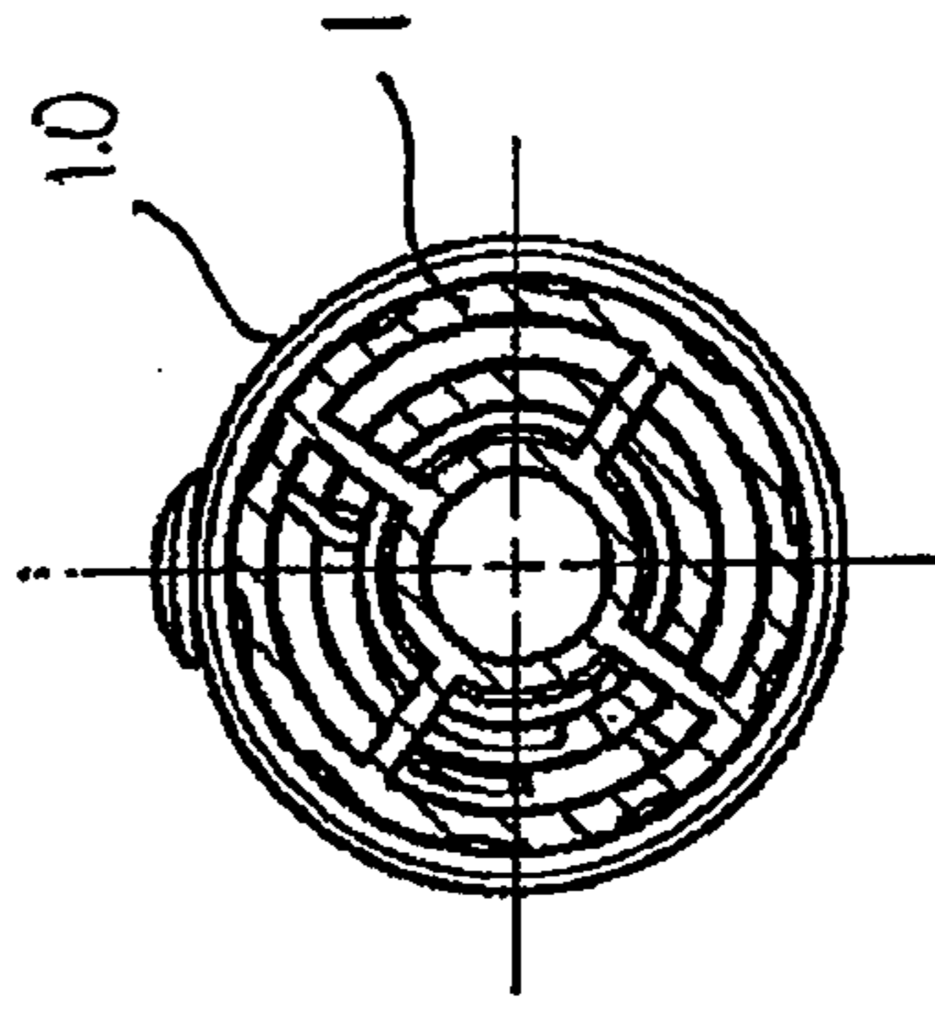
Fig. 4C C-C M 2:1
