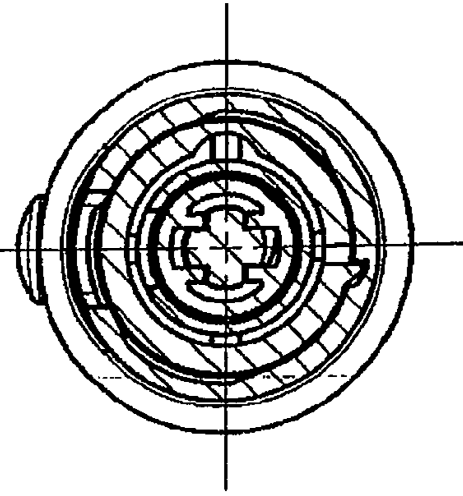
Fig. 6C C-C M 2:1
