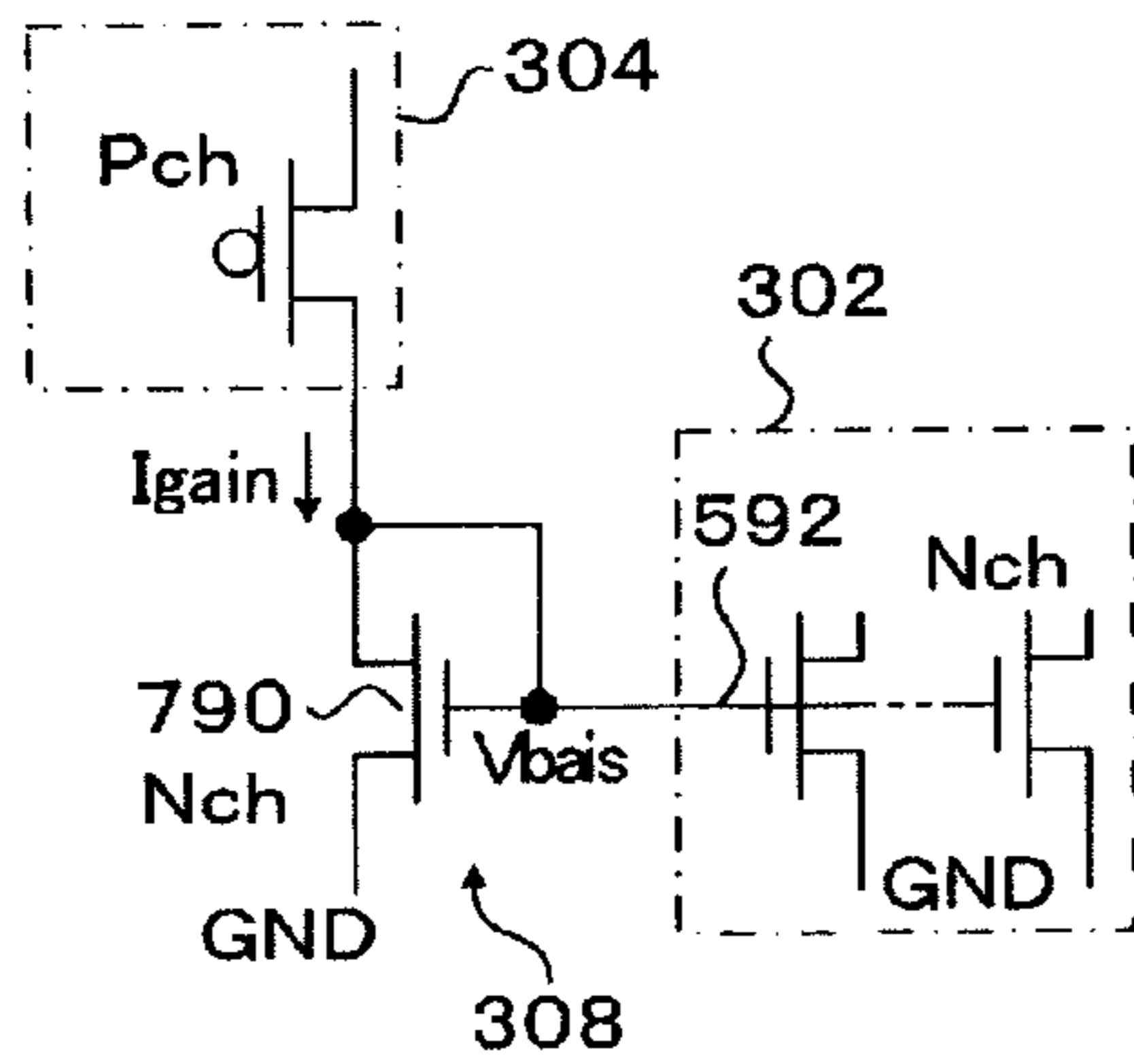
FIG. 4D
