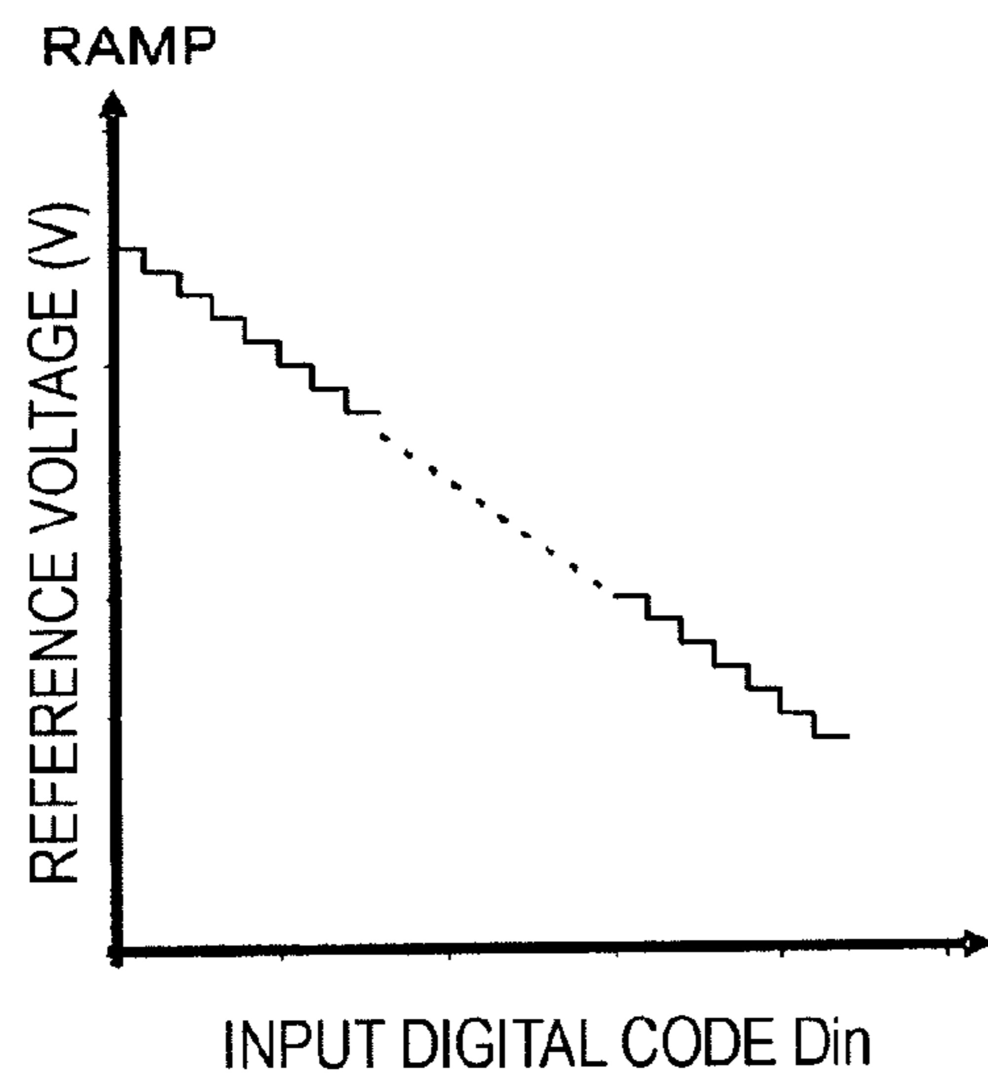
FIG. 11C
