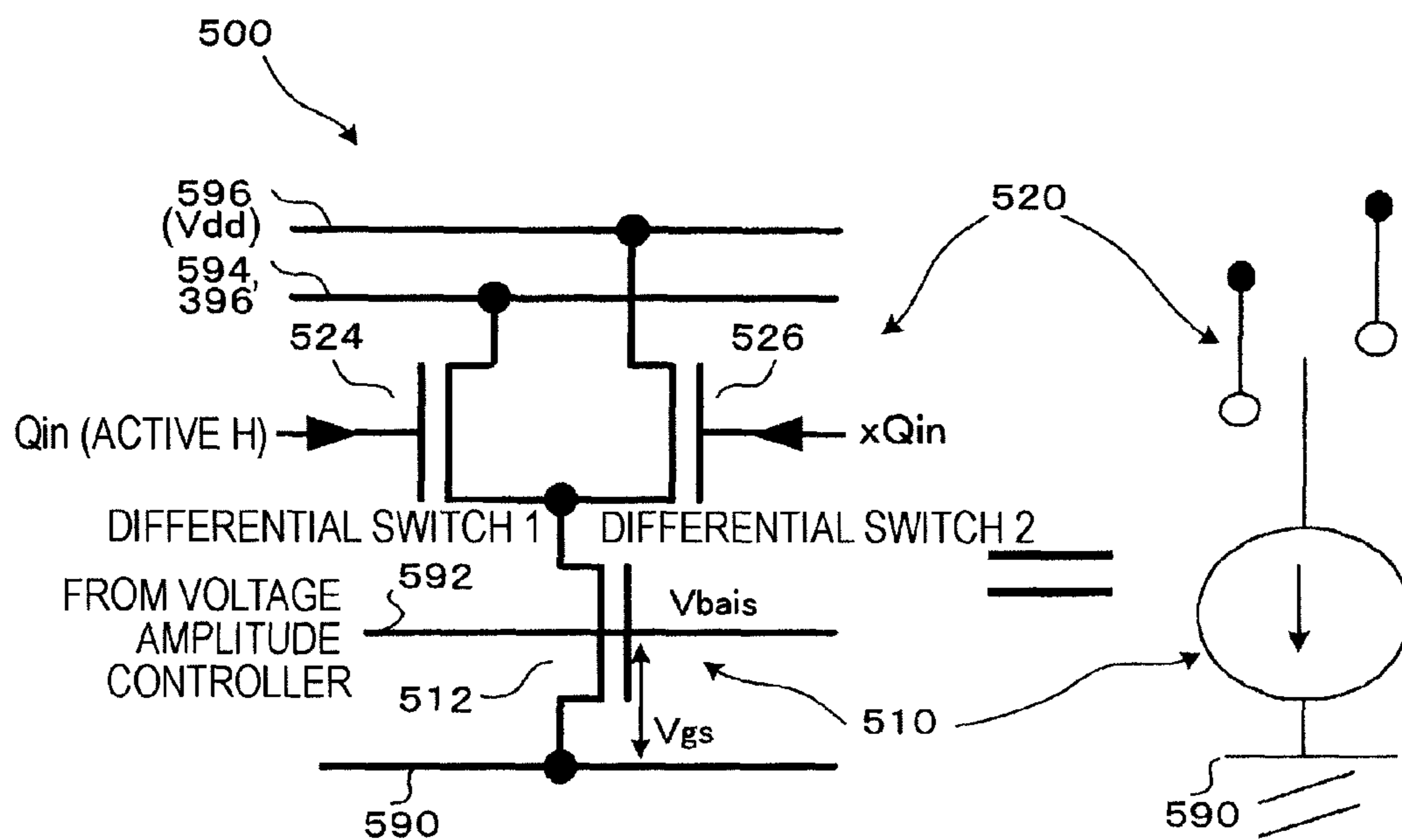
FIG. 8A
