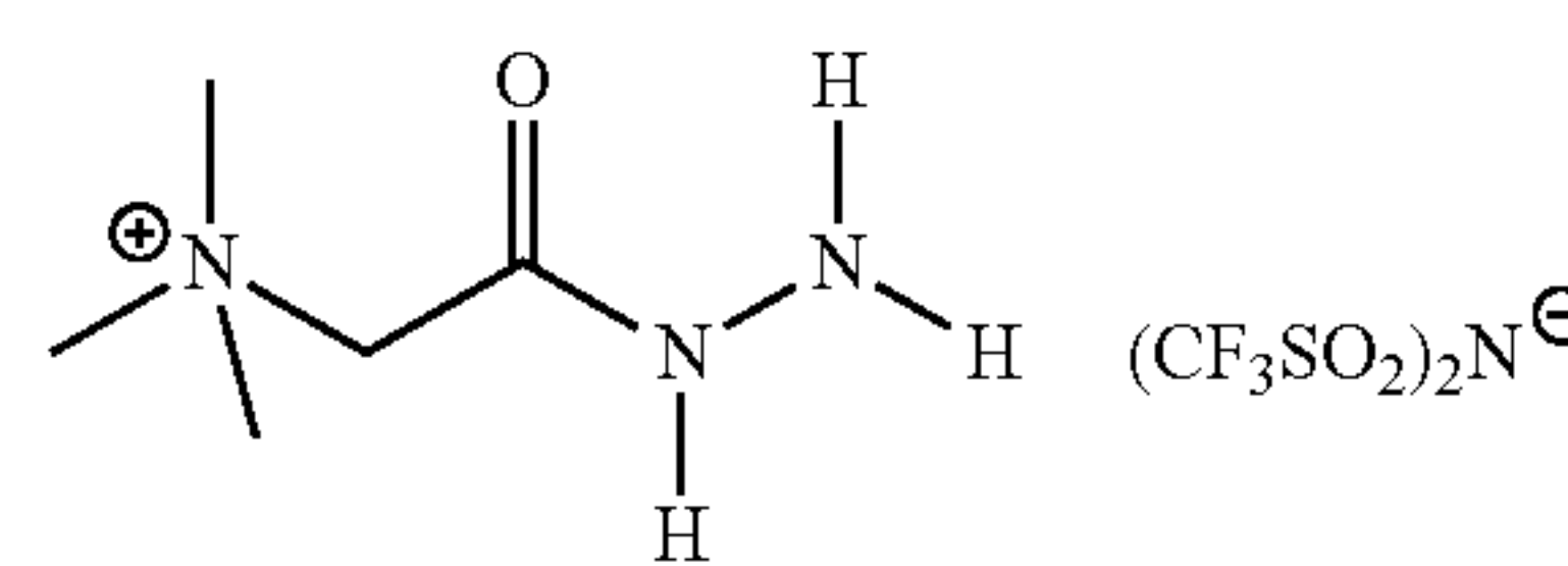
Amine IL 6
