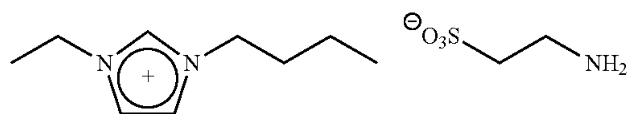
Amine IL 5
