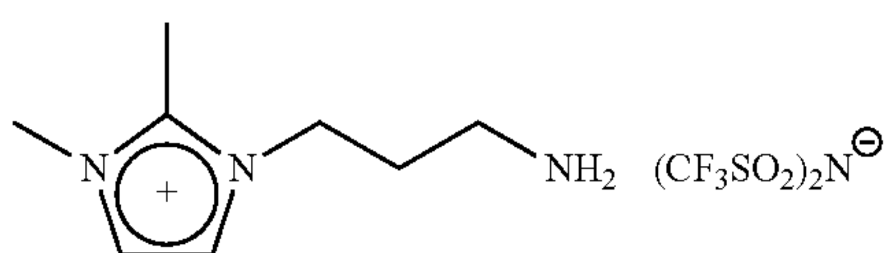
Amine IL 1
