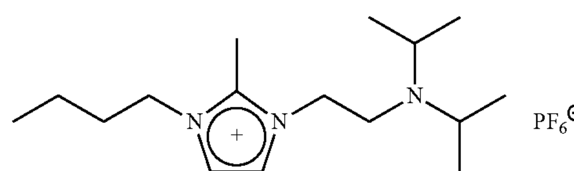
Amine IL 2
