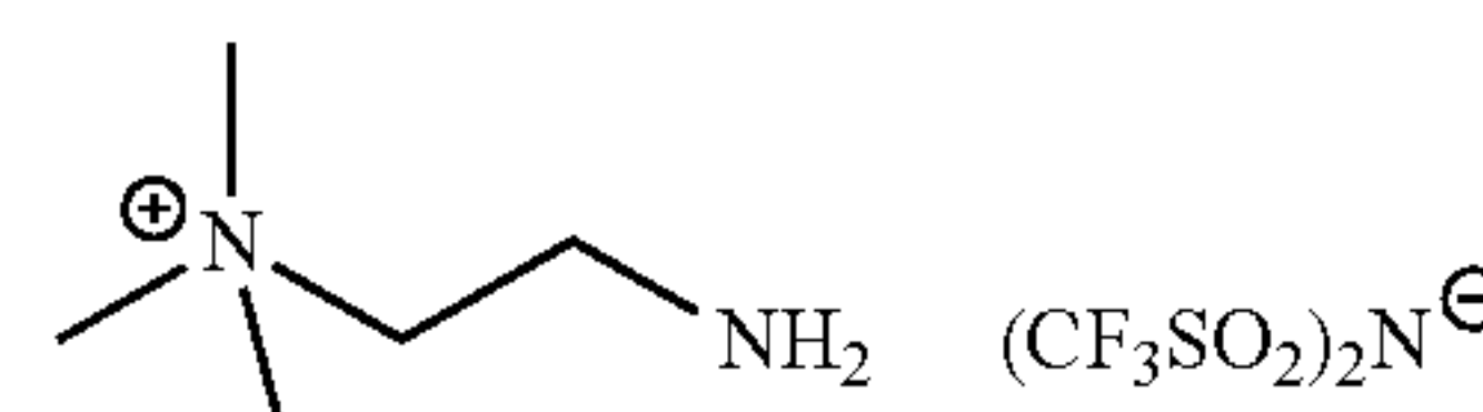
Amine IL 7
