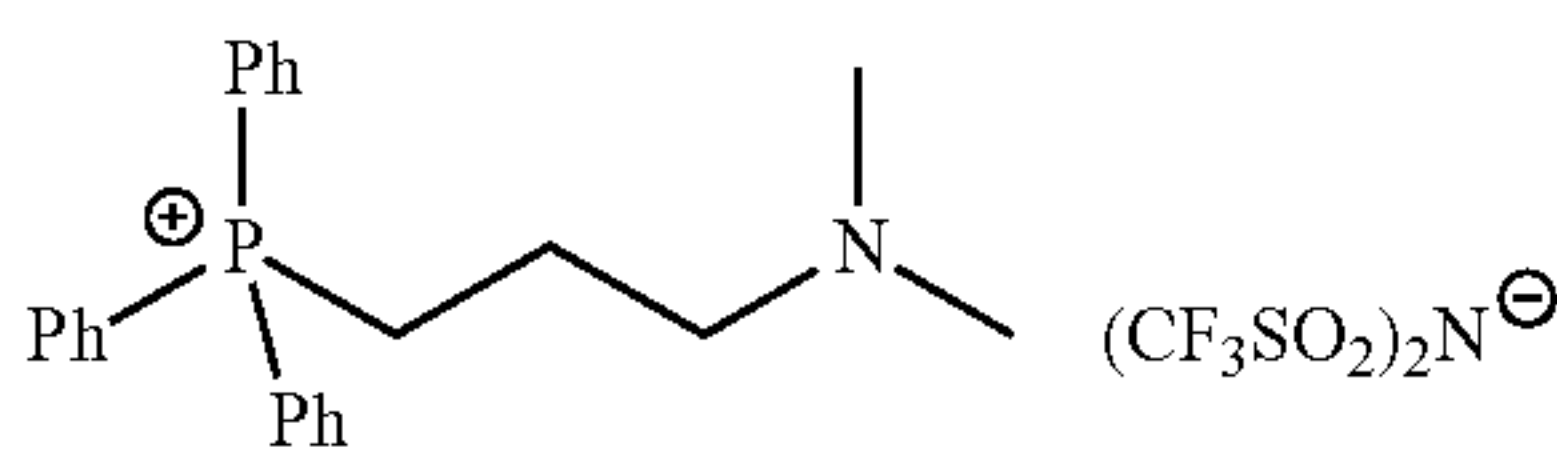
Amine IL 4
