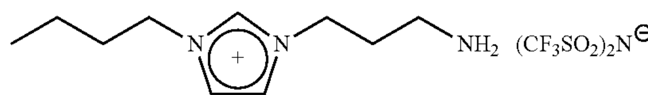
Amine IL 3
