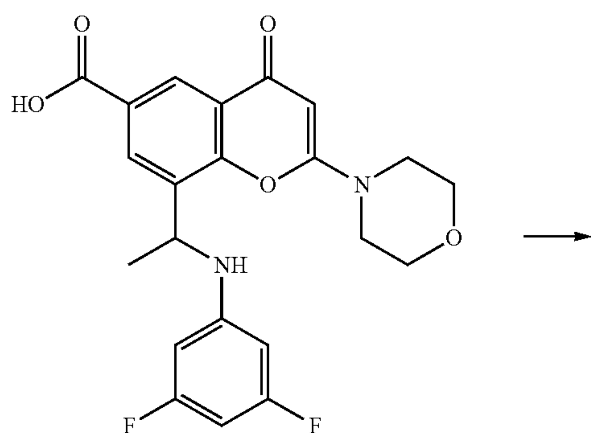
enantiomer 2
