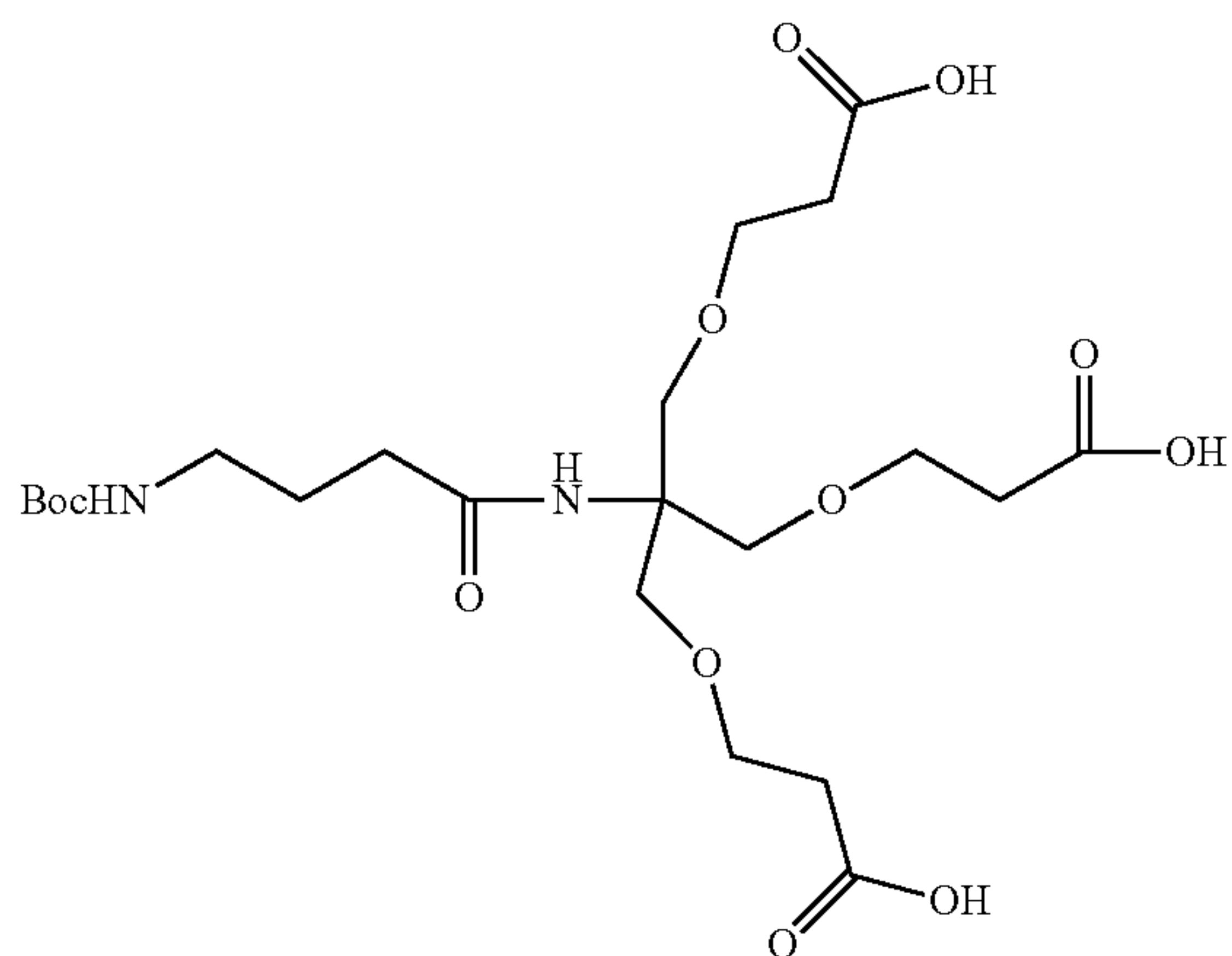
Boc-[3]-acid
