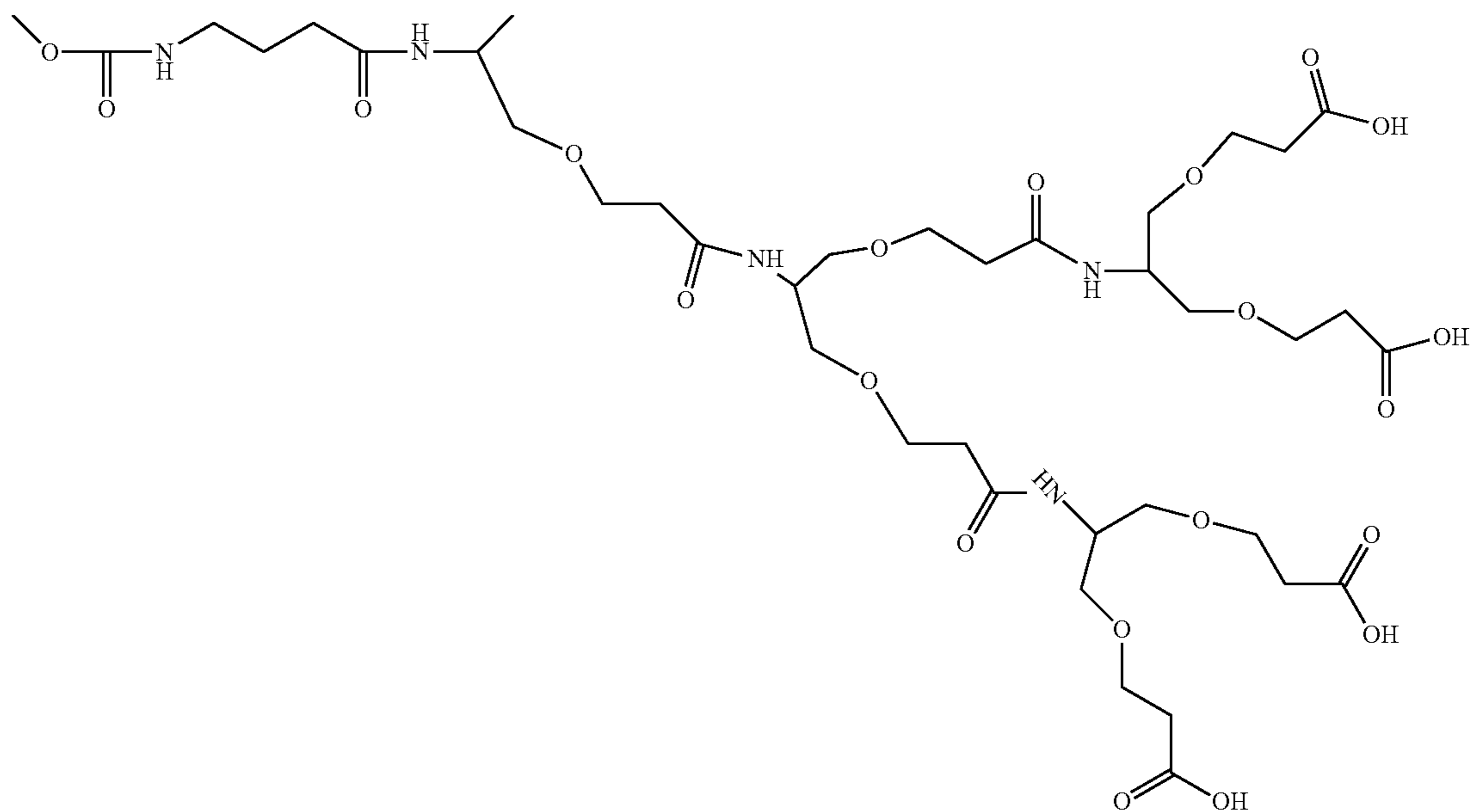
A-[8]-Acid
