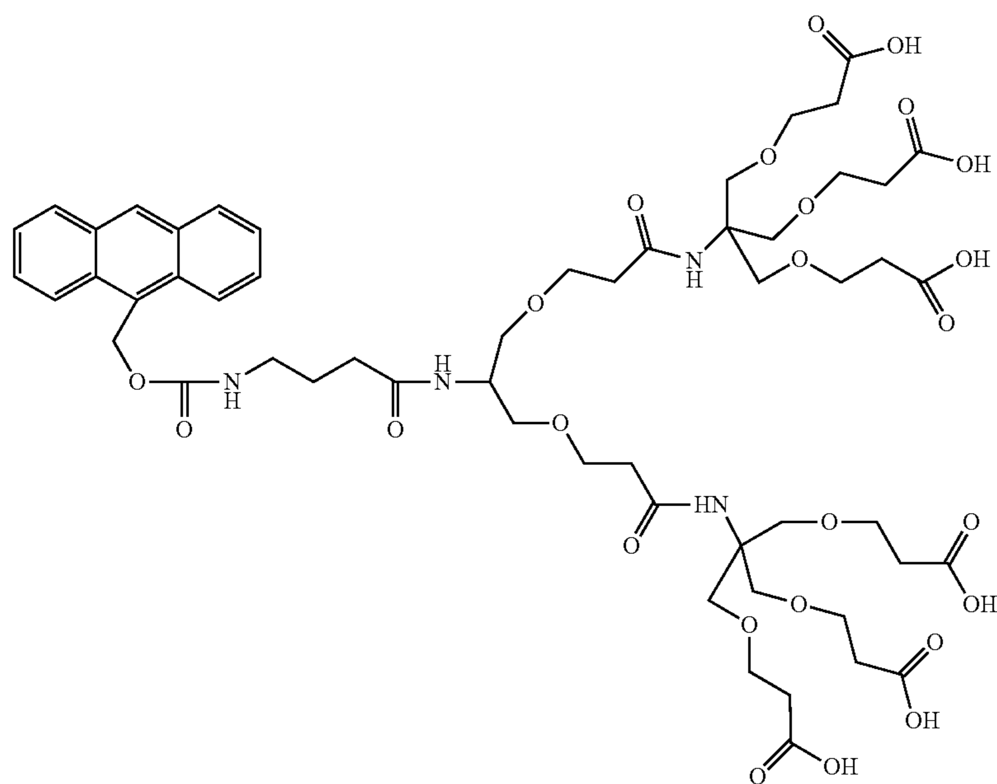
A-[6]-acid
