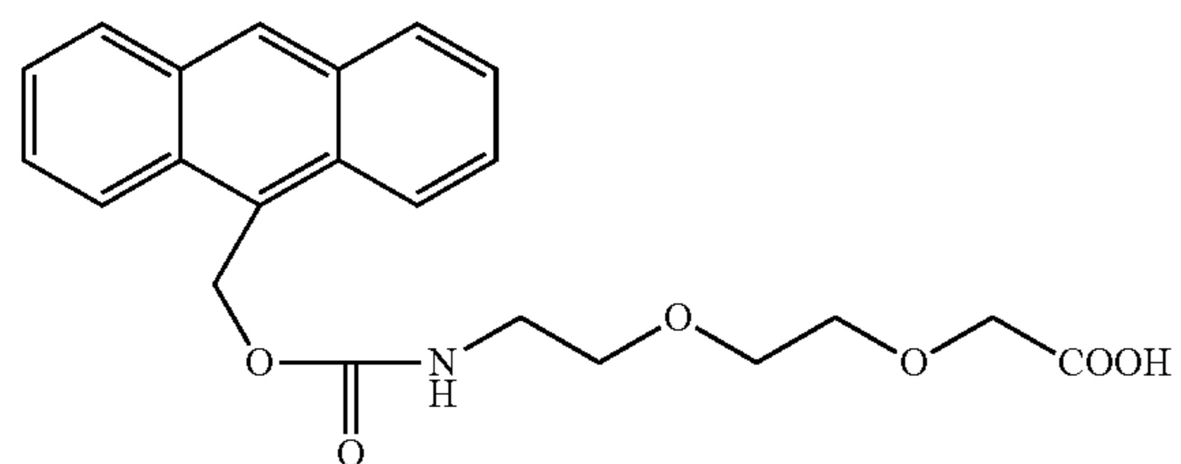
AE-[1]-acid
