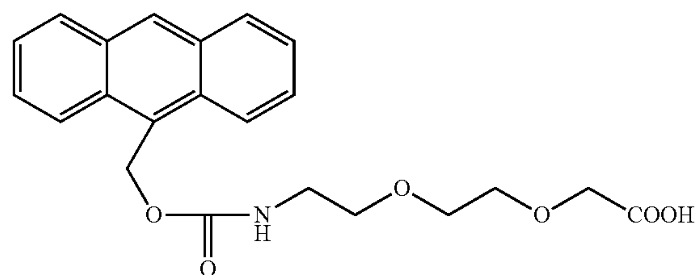
AE-[1]-acid
