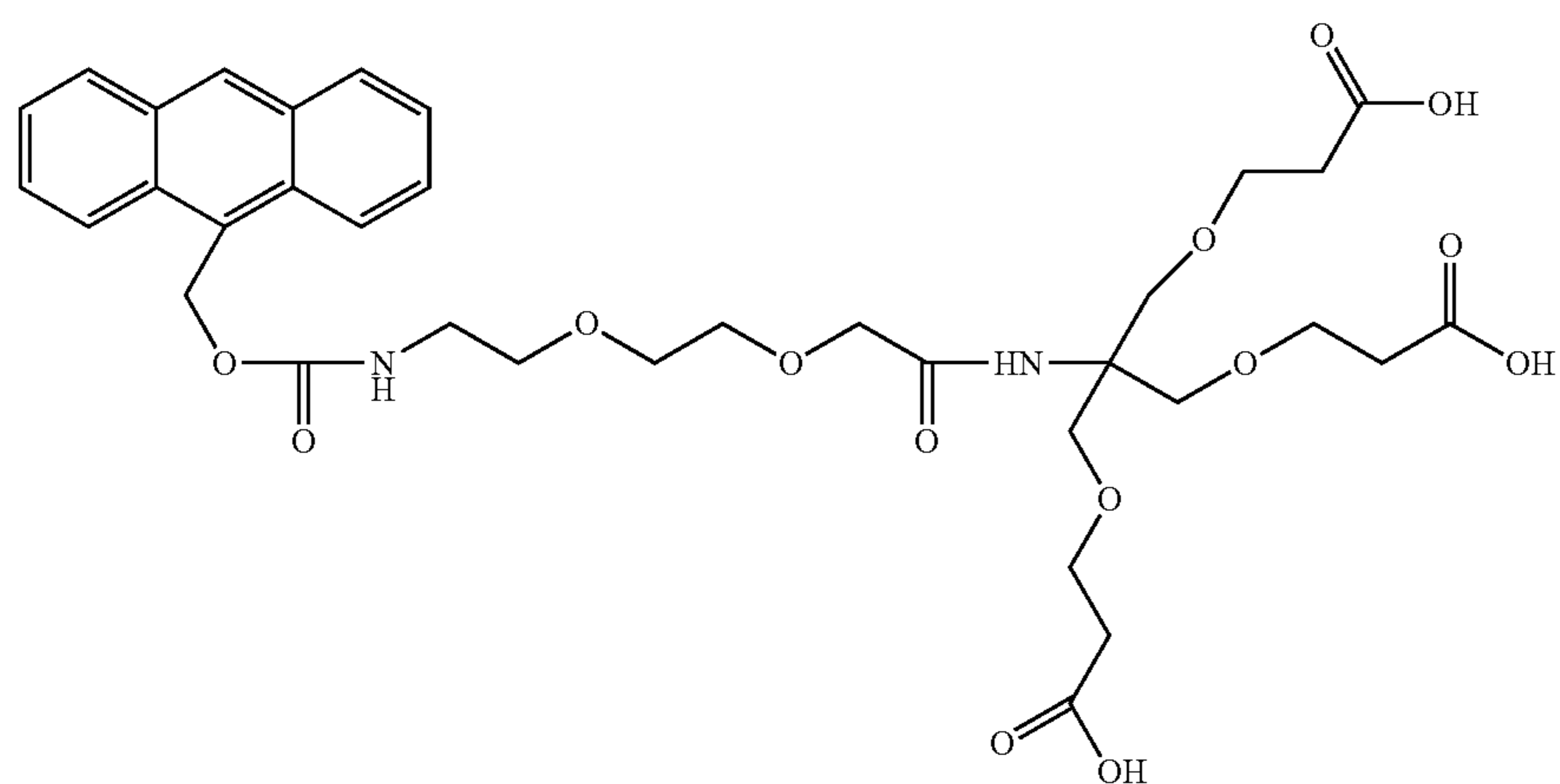
AE-[3]-acid
