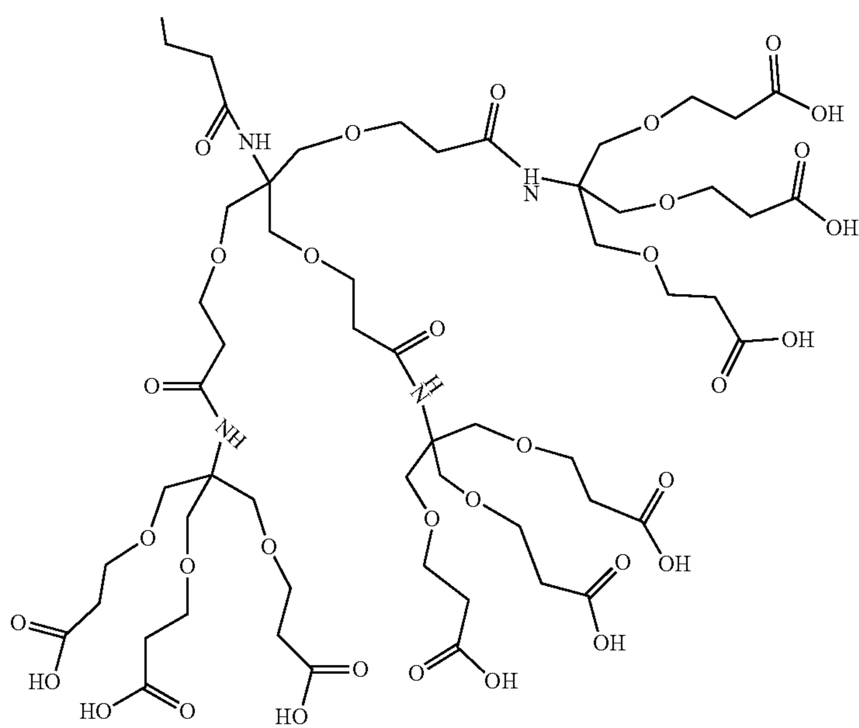
A-[18]-Acid
