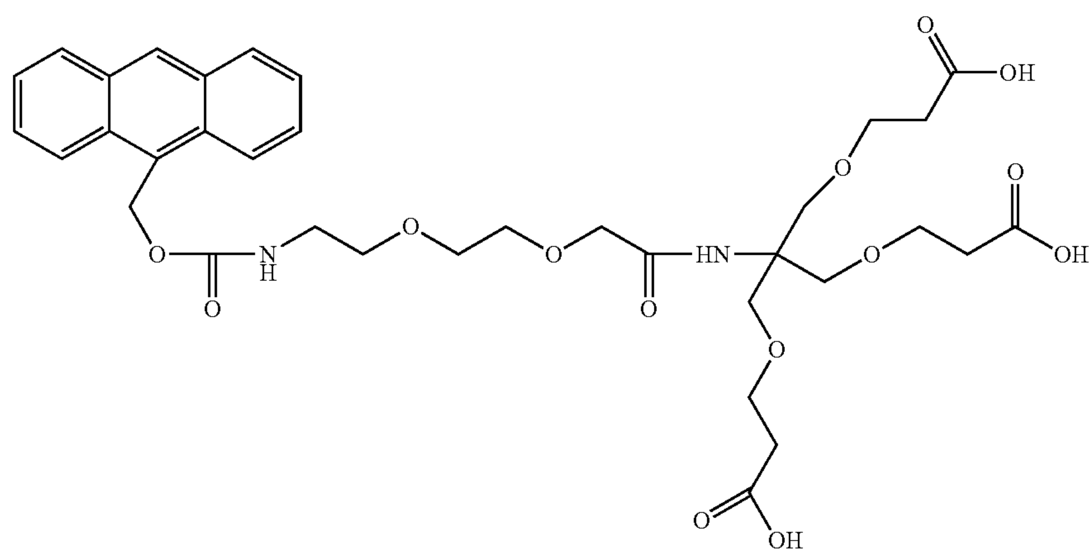
AE-[3]-acid
