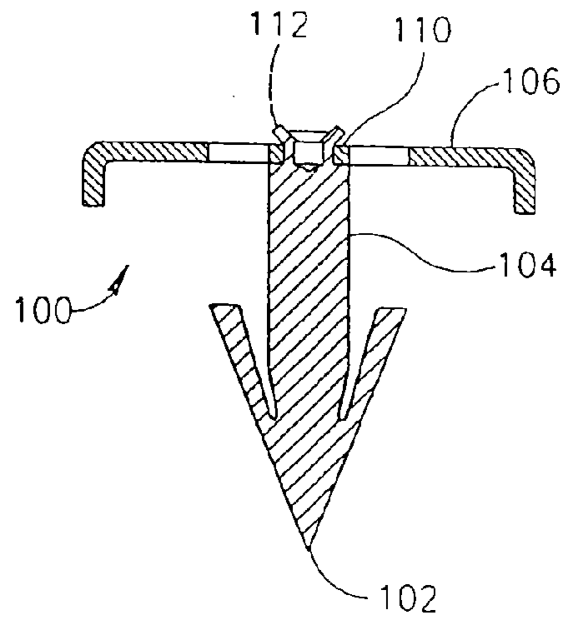
FIG. 9D
