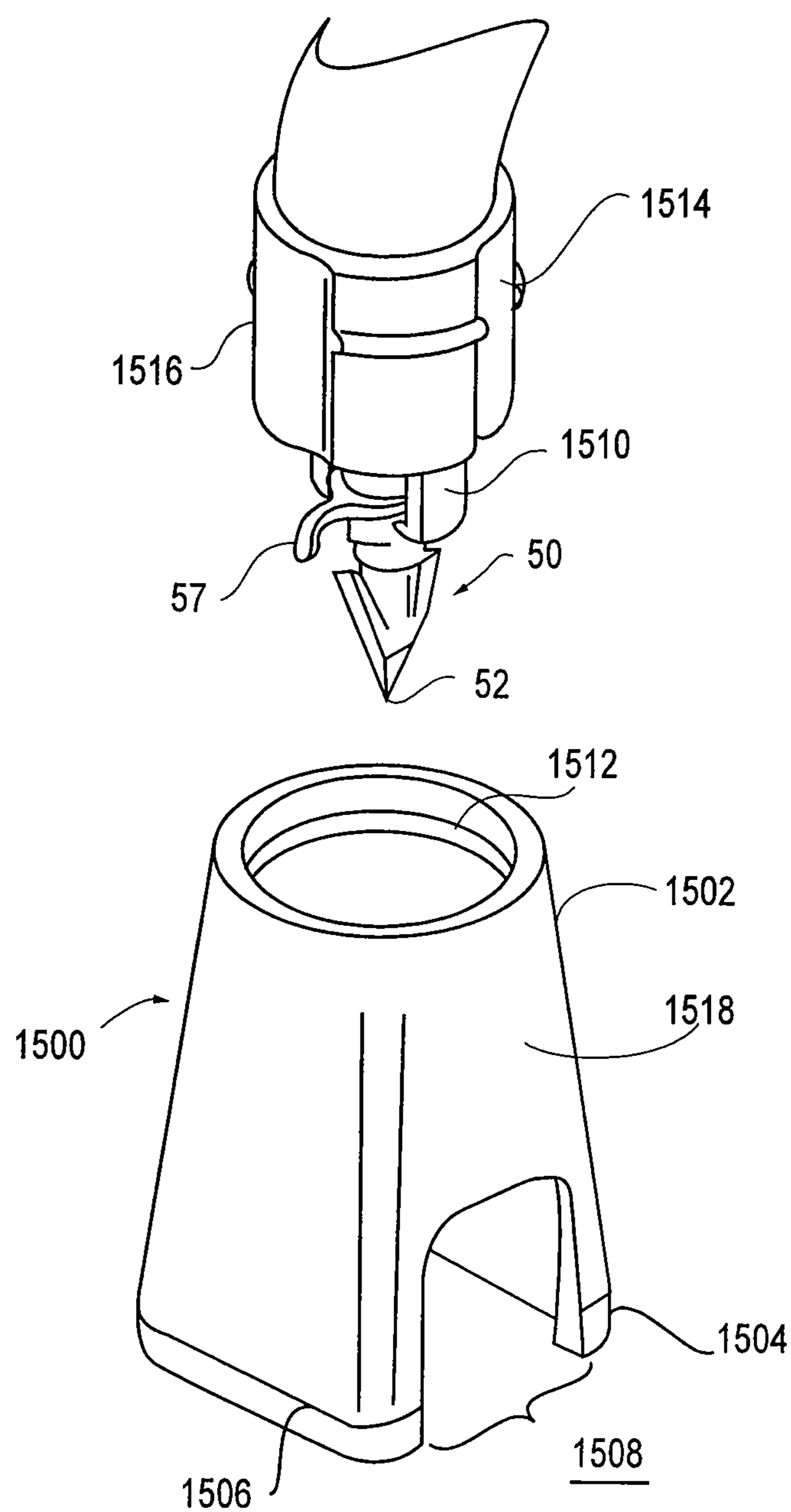
FIG. 15B
