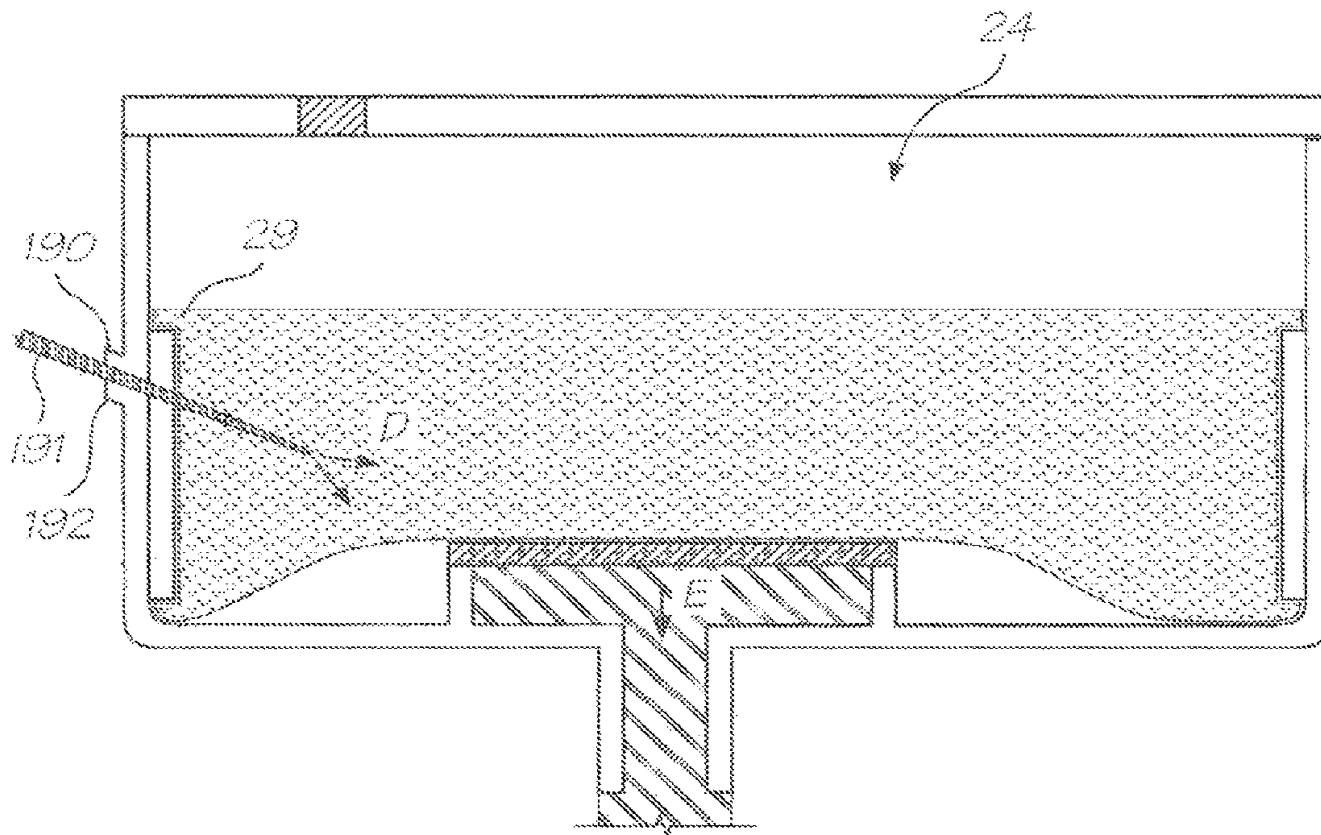
FIG. 40
