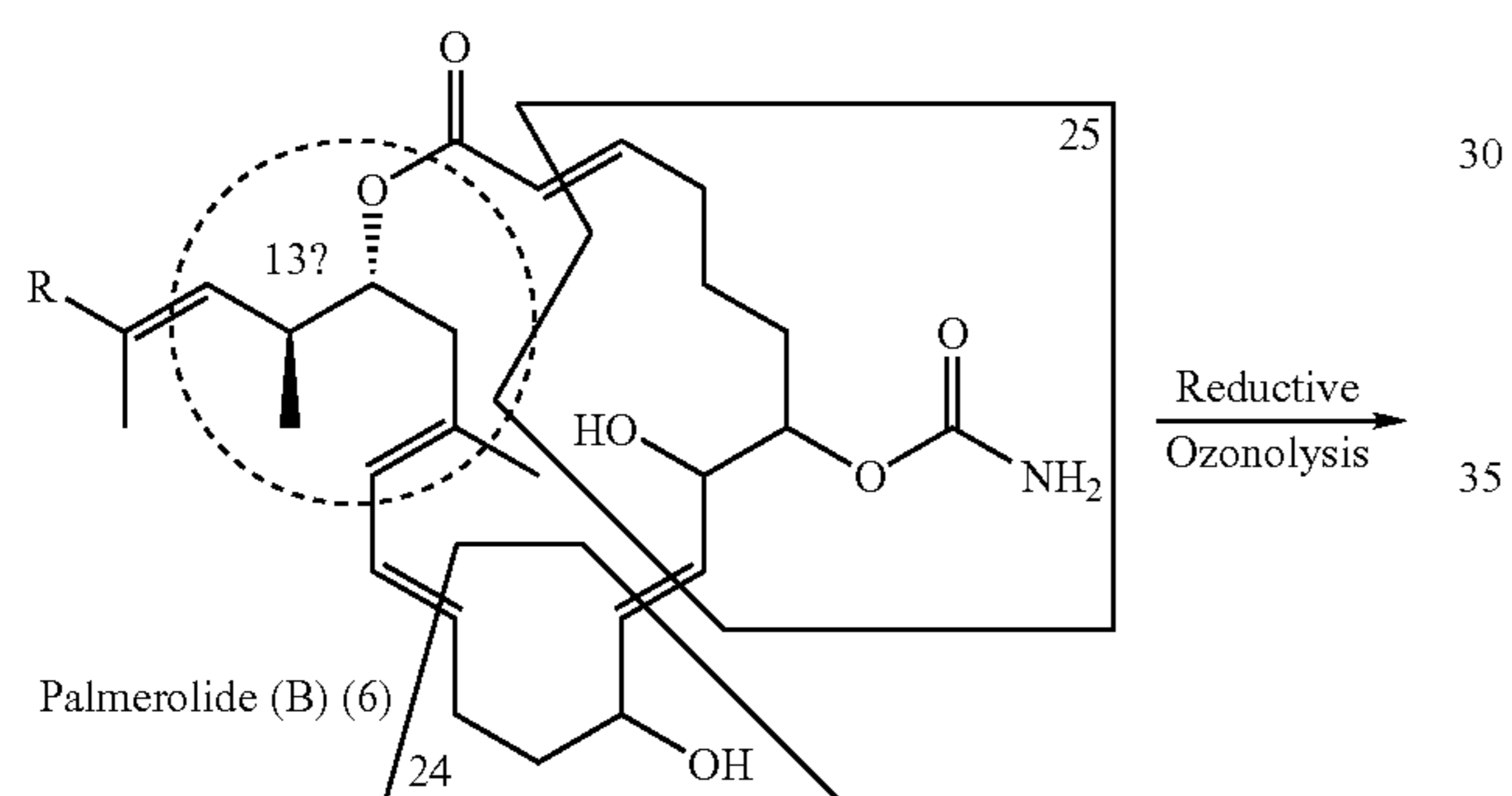
Scheme 4. Ozonolysis of palmerolide B (6).
